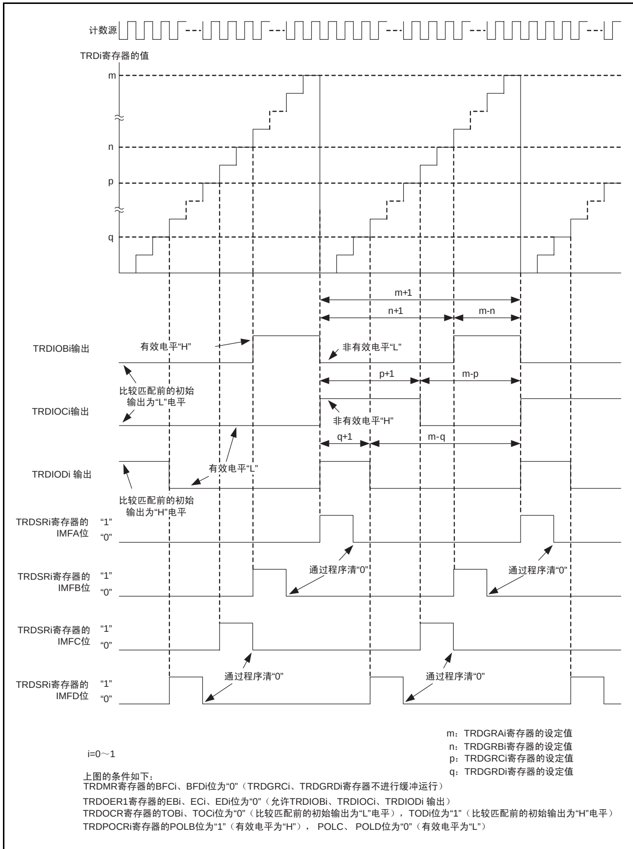
图14 PWM模式的运行示例
