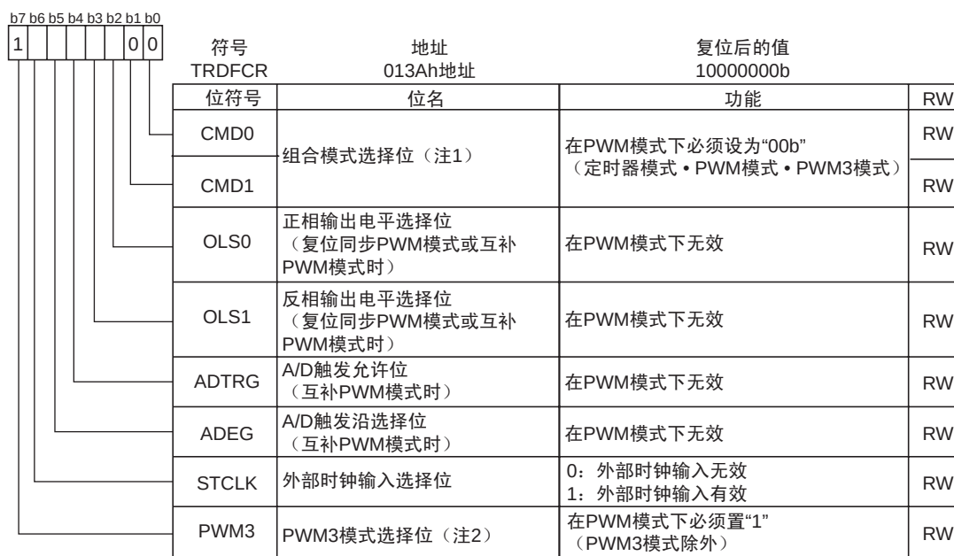
定时器RD功能控制寄存器
