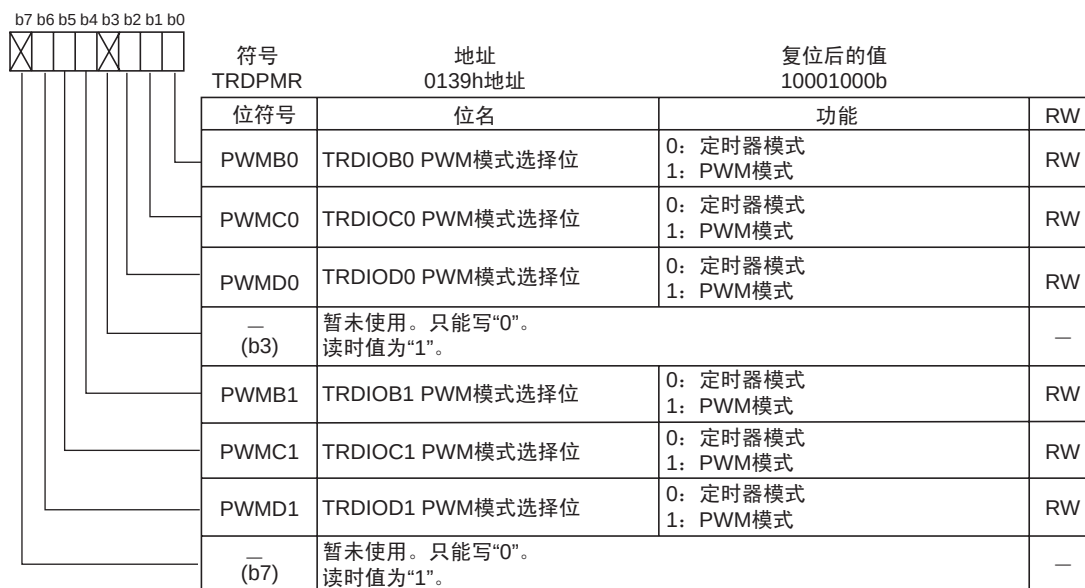
定时器RD PWM模式寄存器
