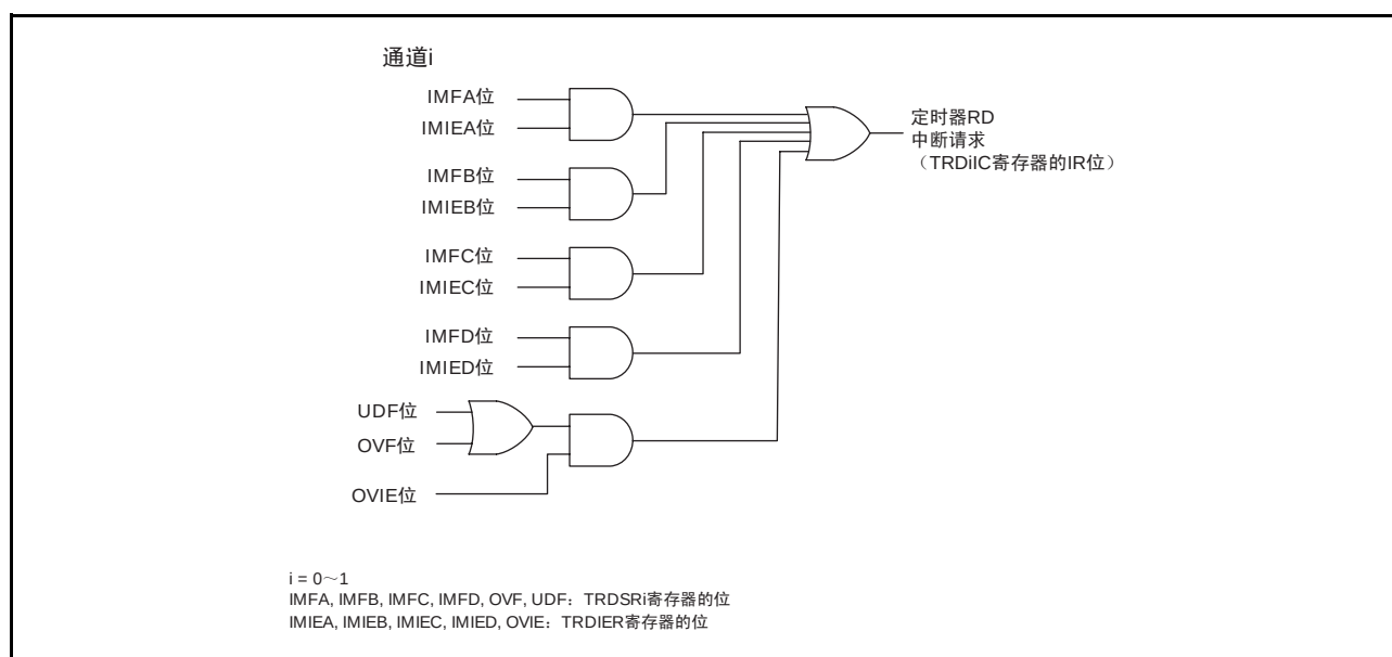
图 16 定时器 RD 中断的框图
