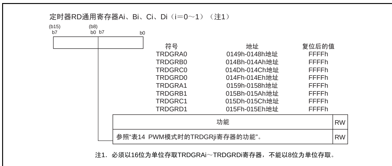
图13 PWM模式时的TRDGRAi、TRDGRBi、TRDGRCi、TRDGRDi寄存器
