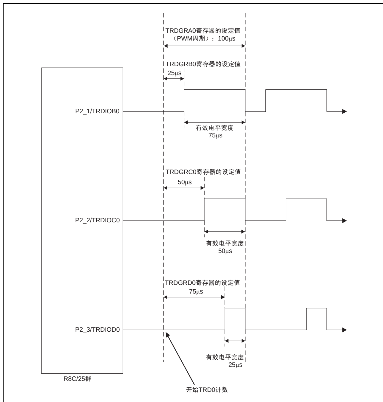
图17 使用的引脚
