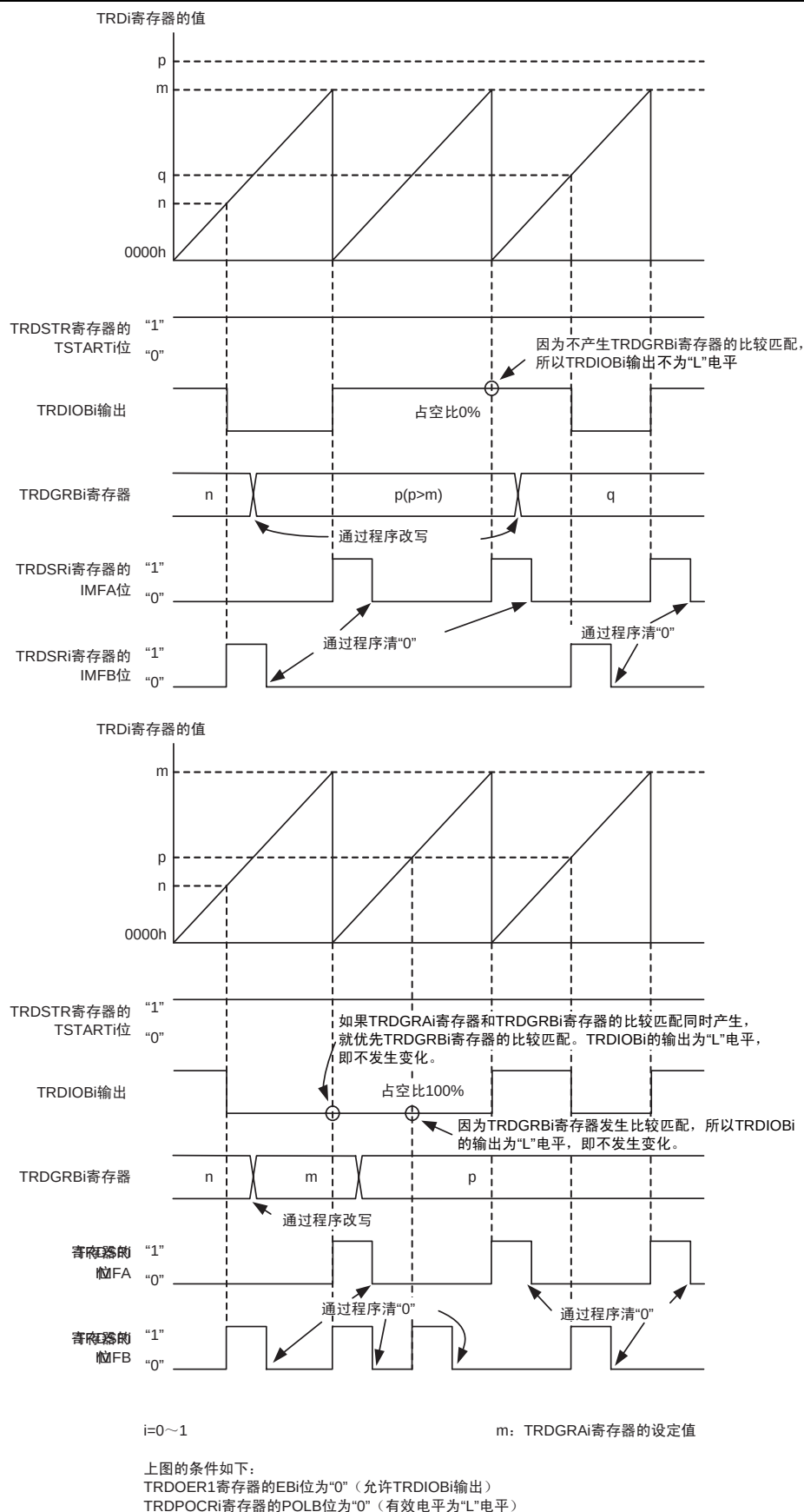
图15 PWM模式时的运行示例 (占空比0%、占空比100%)
