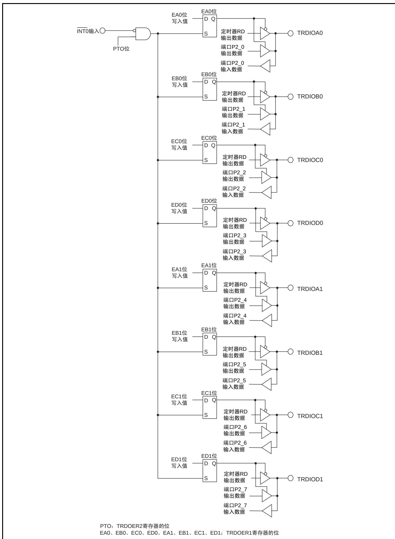
图3 脉冲输出强制截止
