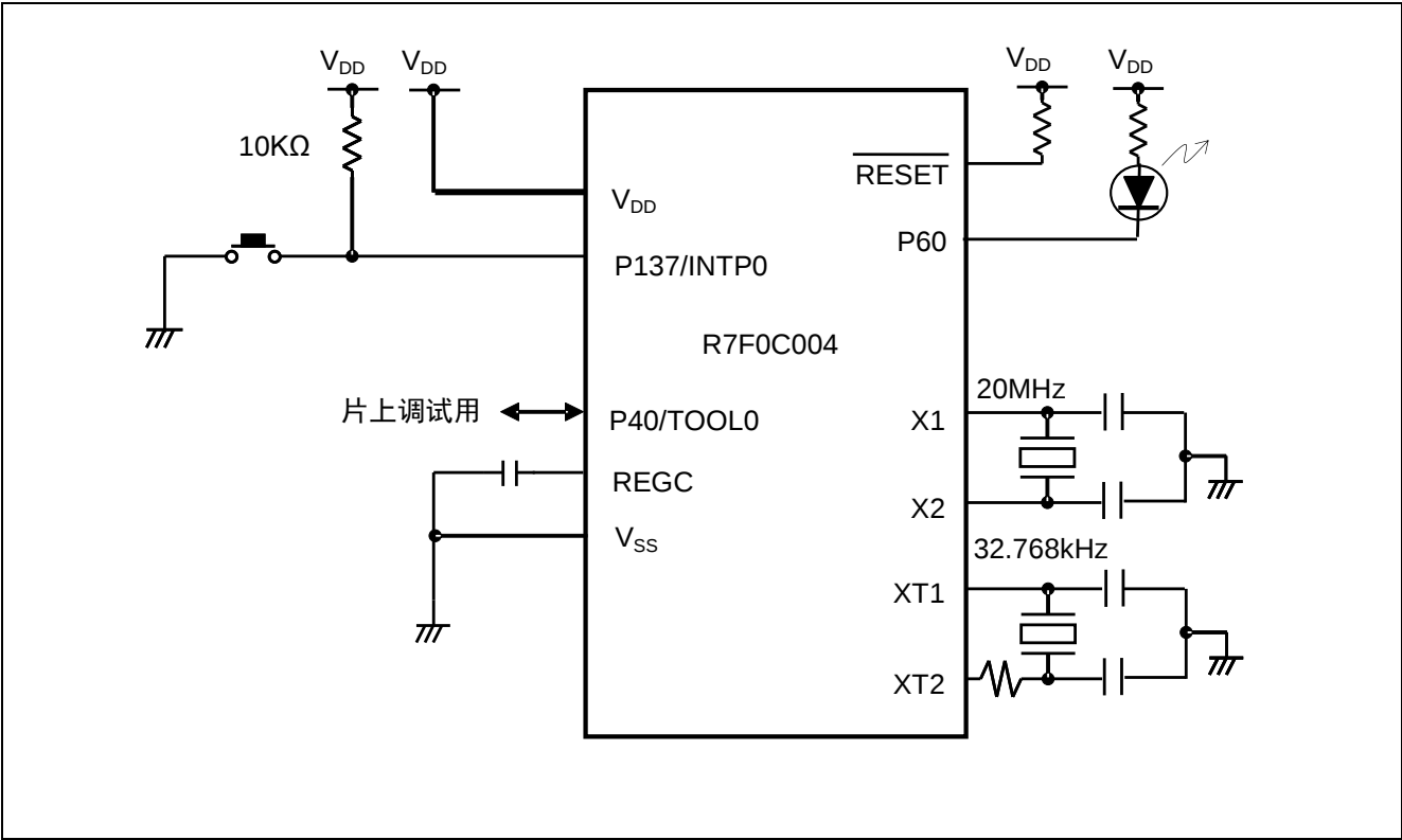
图 3.1 硬件配置
