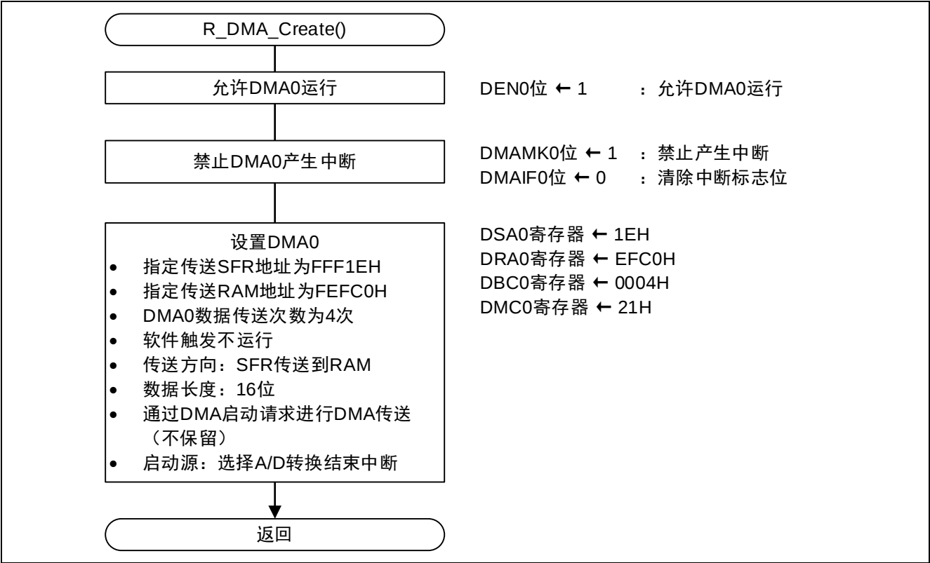
图 4.7 DMA 初始化设置
