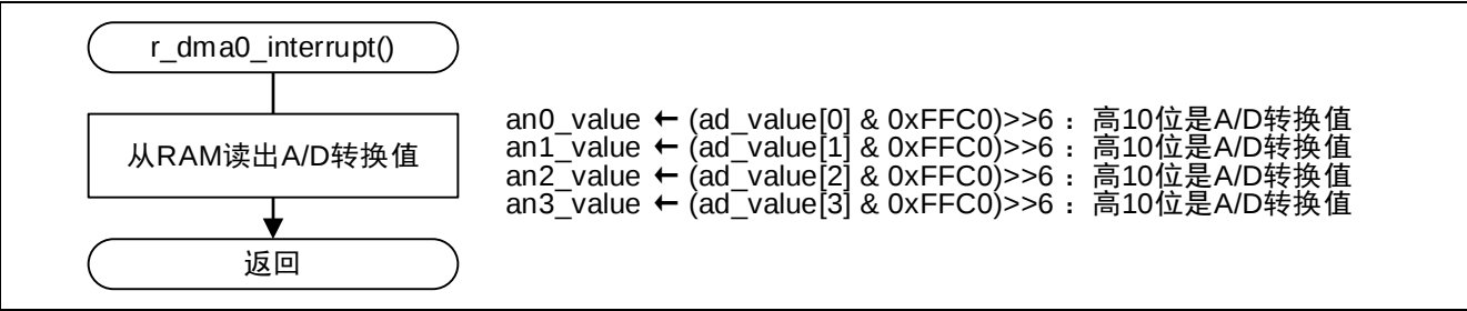
图 4.11 DMA0 传送结束中断
