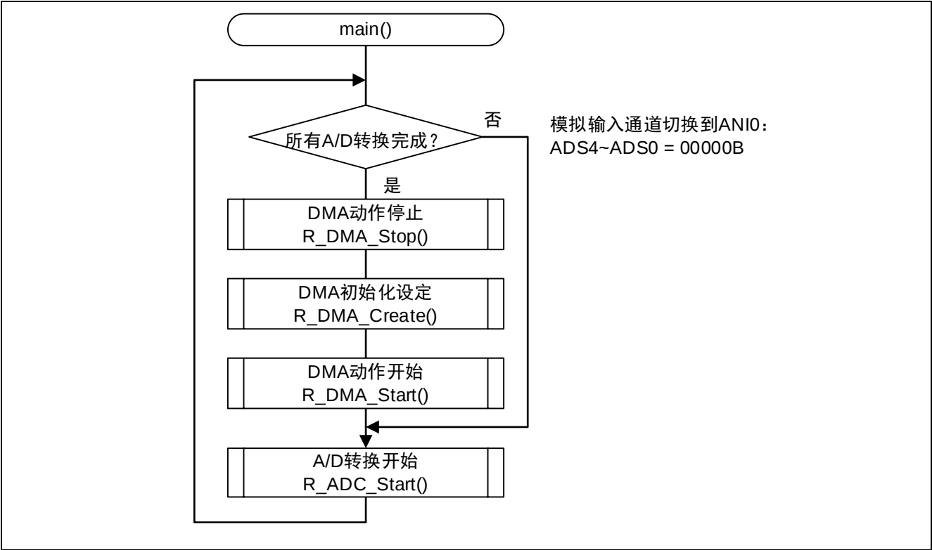
图 4.8 主函数处理
