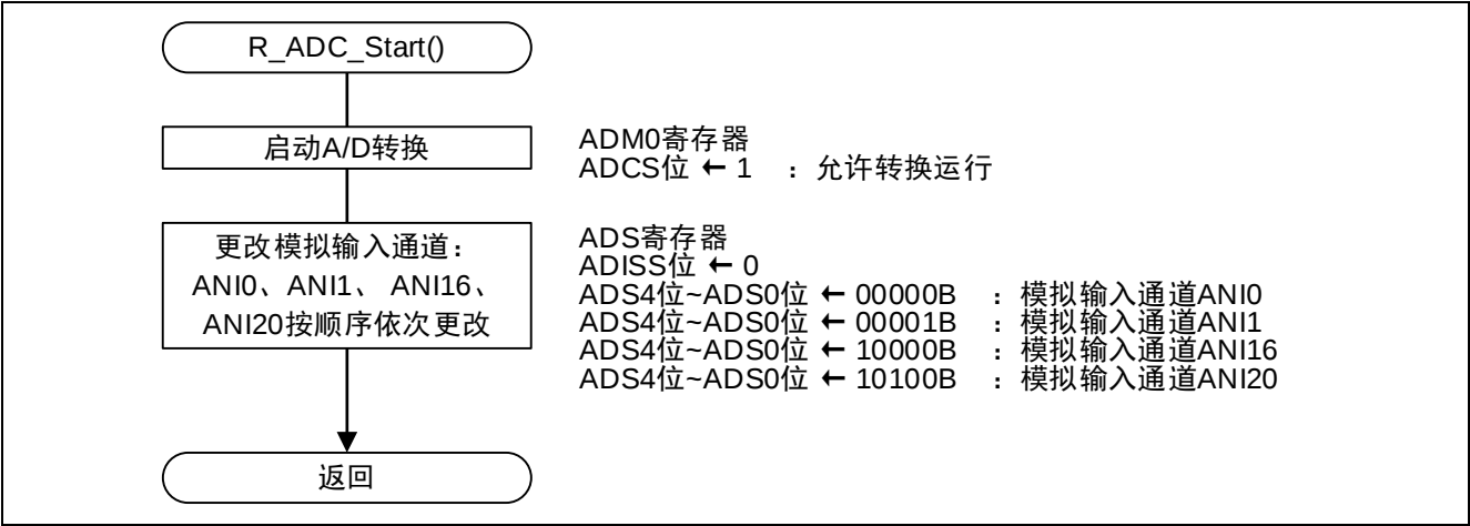
图 4.10 A/D 转换动作开始
