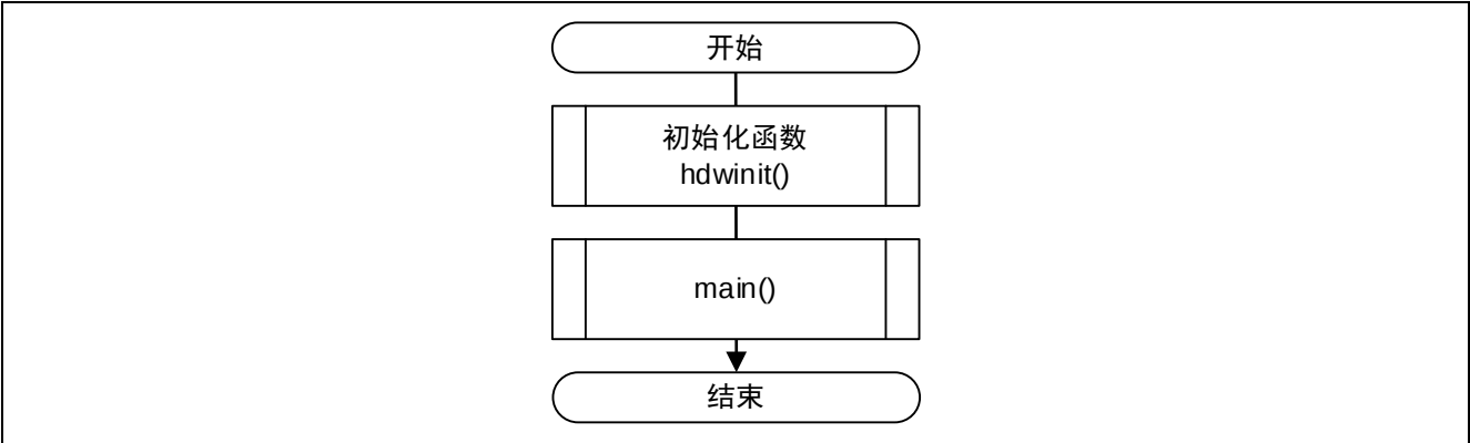
图 4.2 整体流程图
