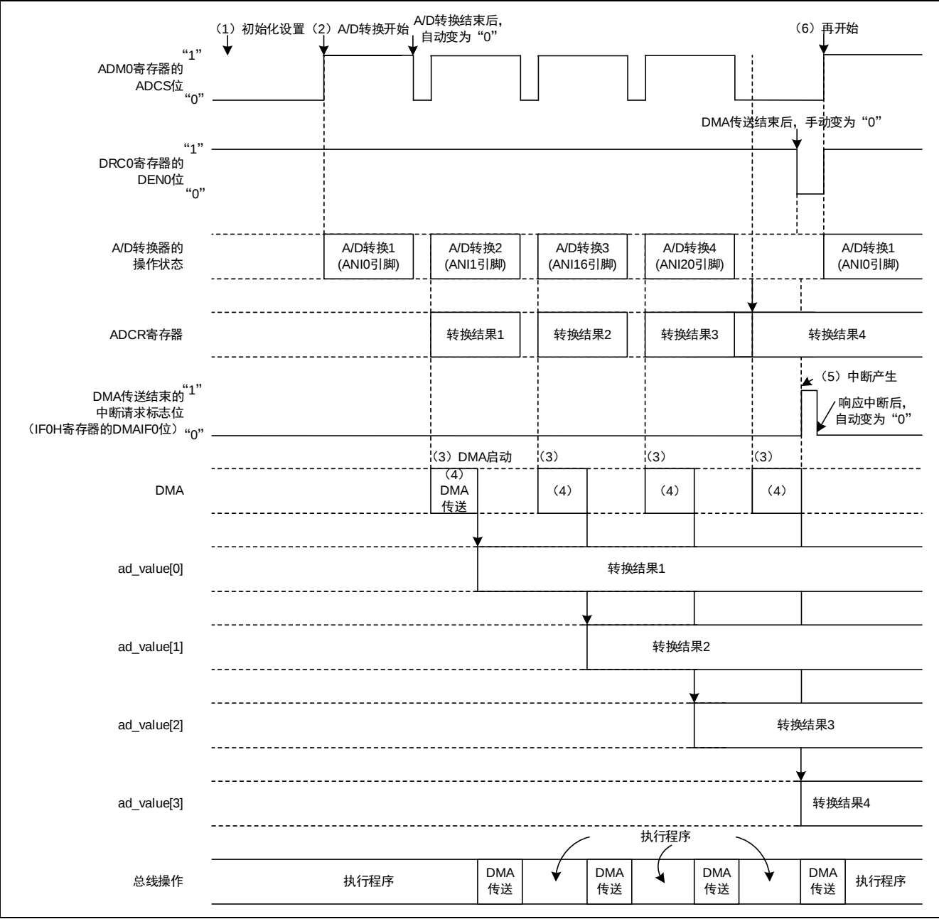
图 4.1 DMA 传送和 A/D 转换的时序图
