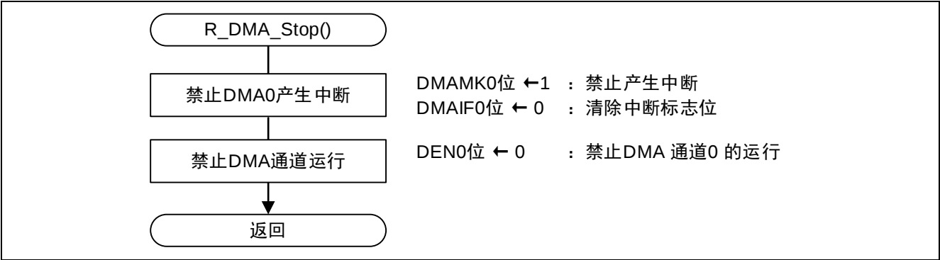
图 4.12 DMA 动作停止
