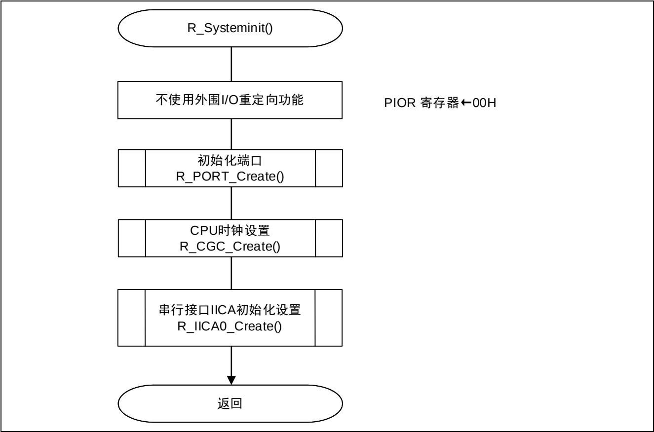
图 5.3 系统函数
