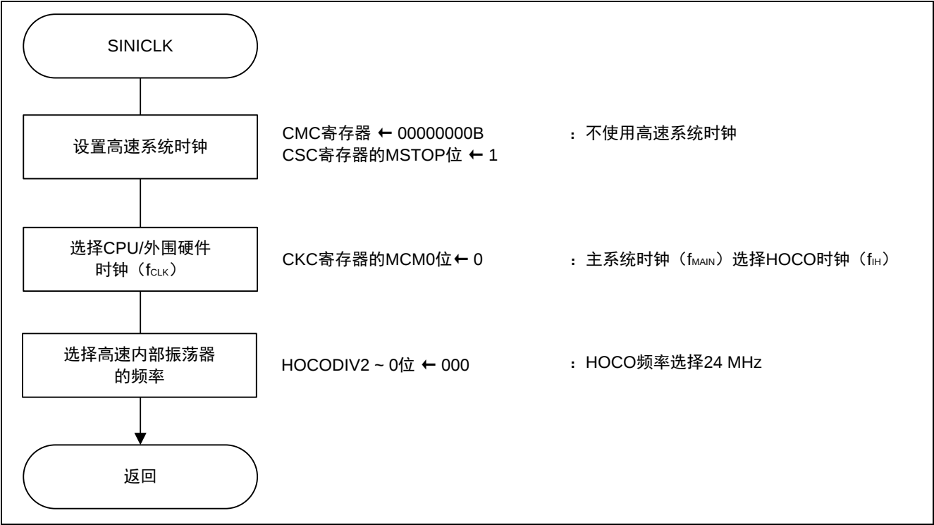
图 4.4 设置时钟发生电路
