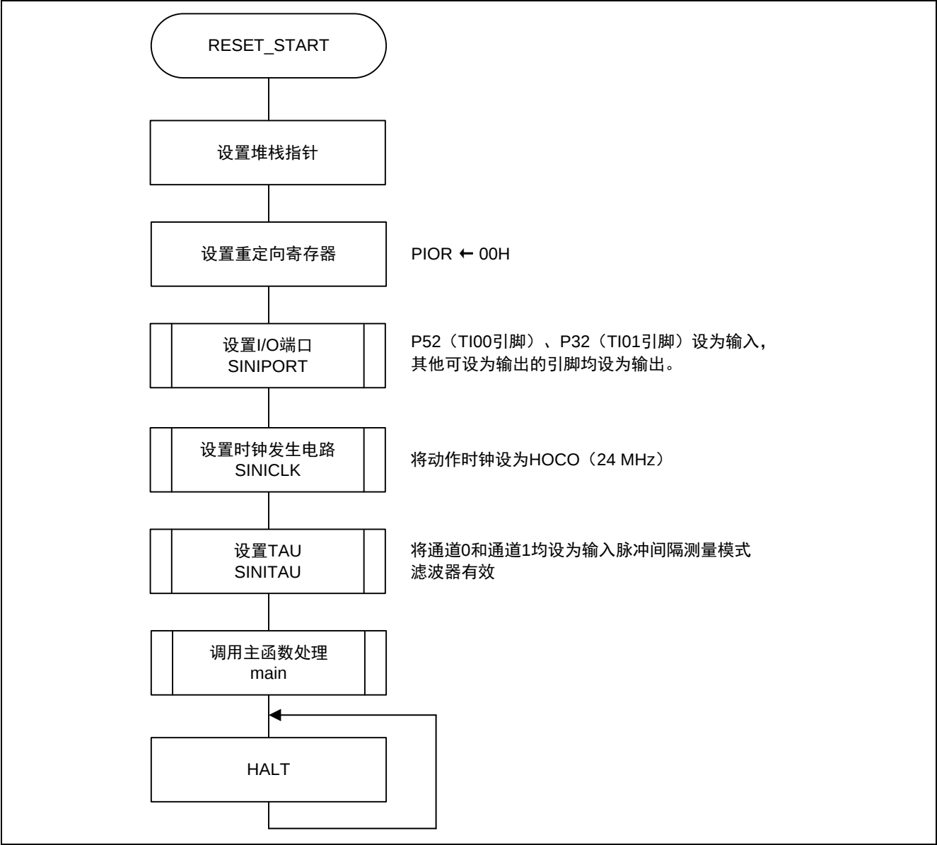
图 4.2 整体流程图
