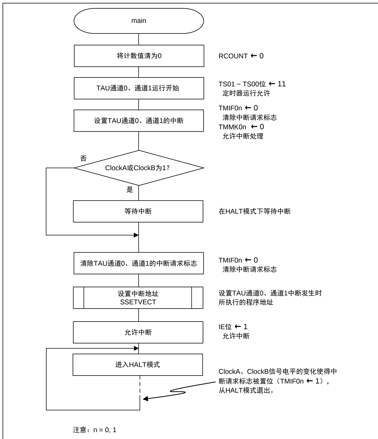
图 4.6 主函数处理
