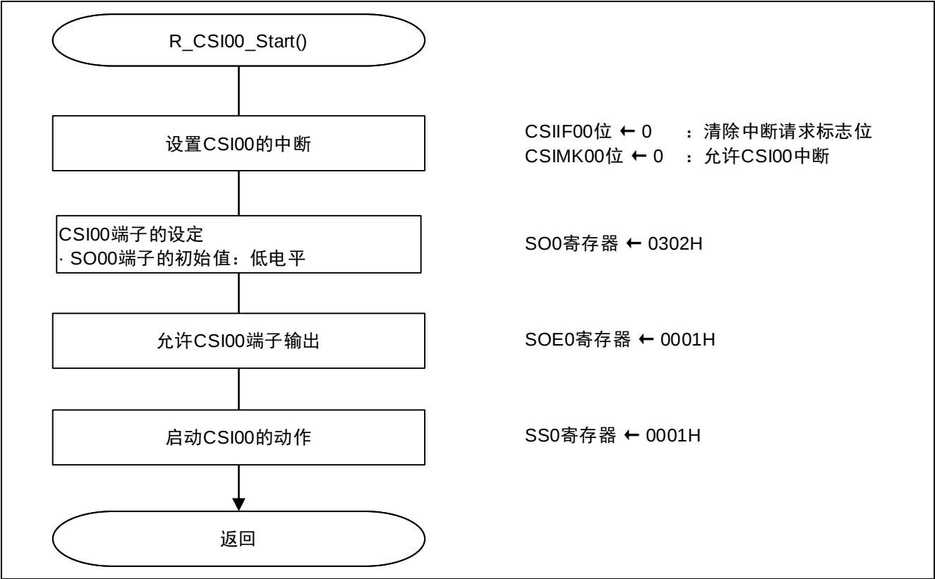
图 5.9 启动 SAU0 通道 0（CSI00）的处理
