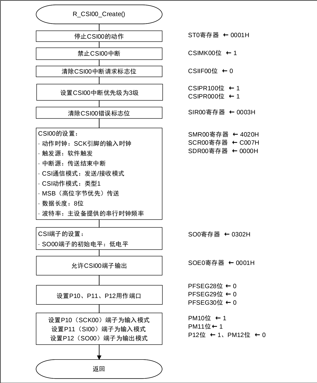
图 5.7 SAU0 通道 0（CSI00）的动作设置
