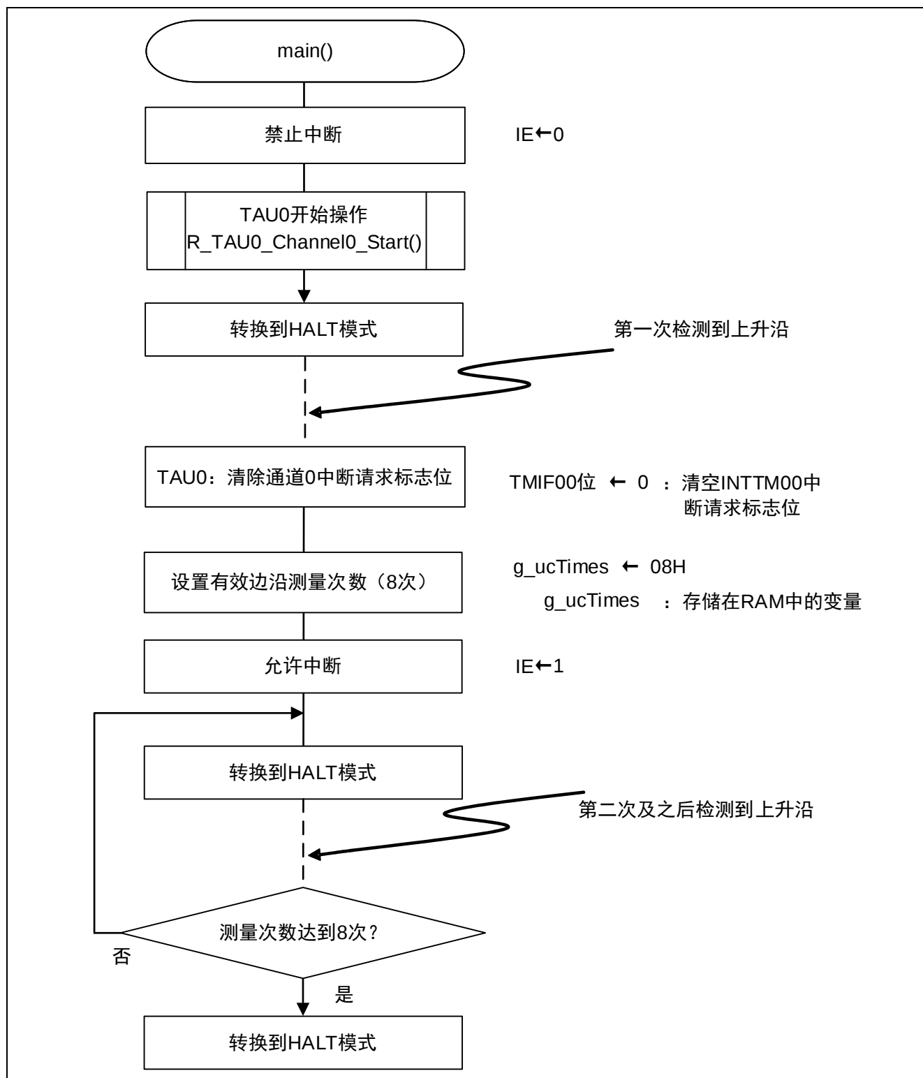
图 4.7 主函数处理
