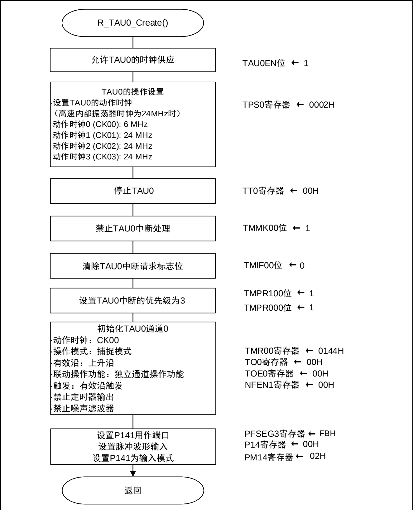
图 4.6 TAU0 初始化
