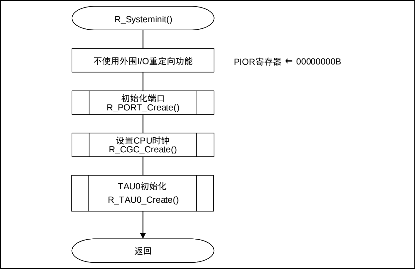
图 4.3 系统函数
