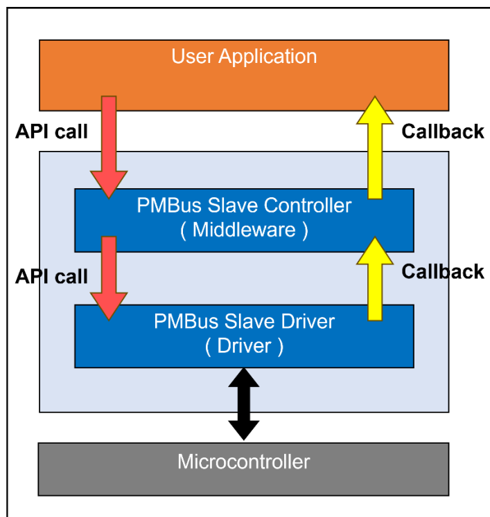
図 1-1 モジュール構成
