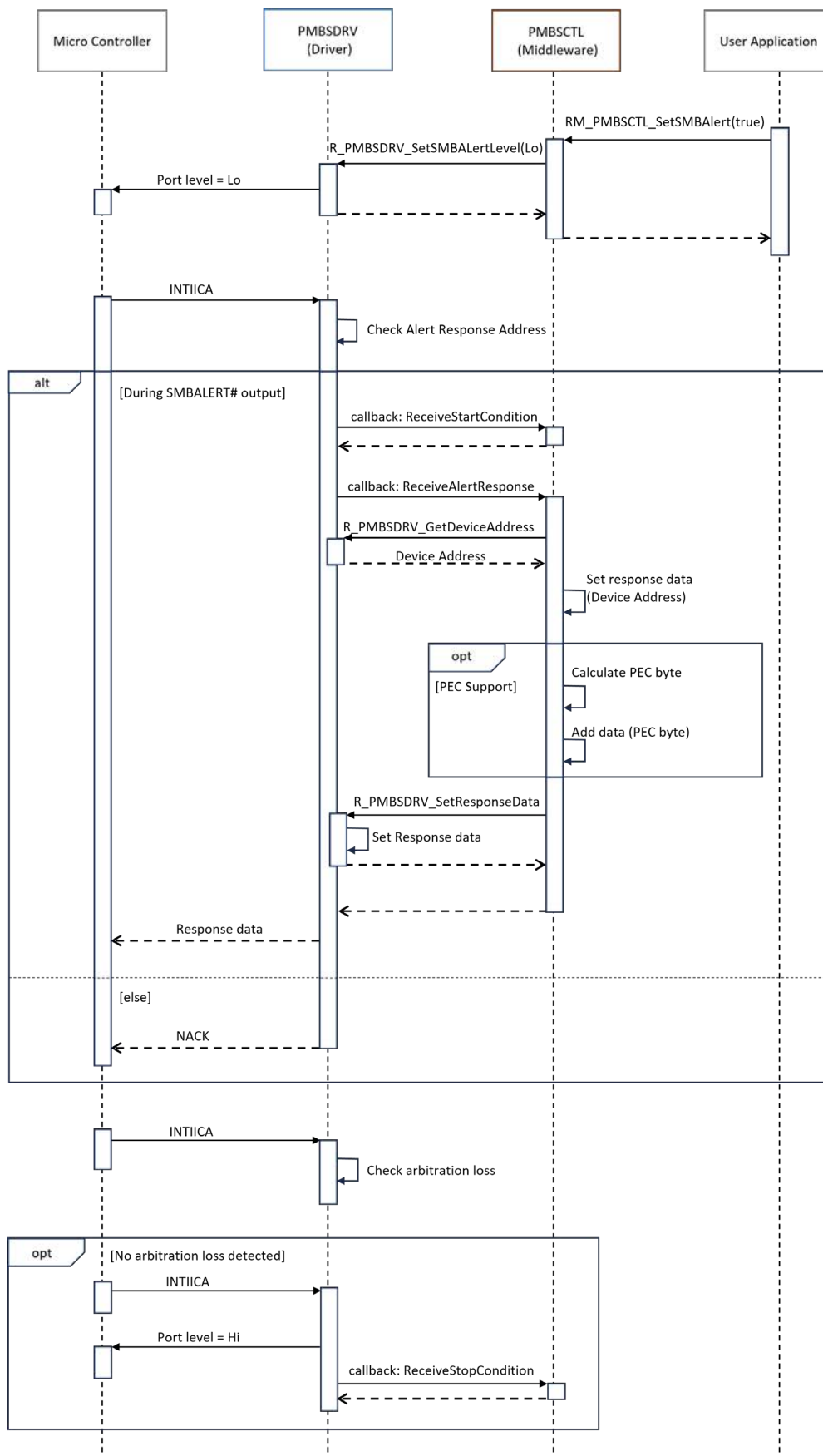
図 5-7 SMBALERT# sequence
