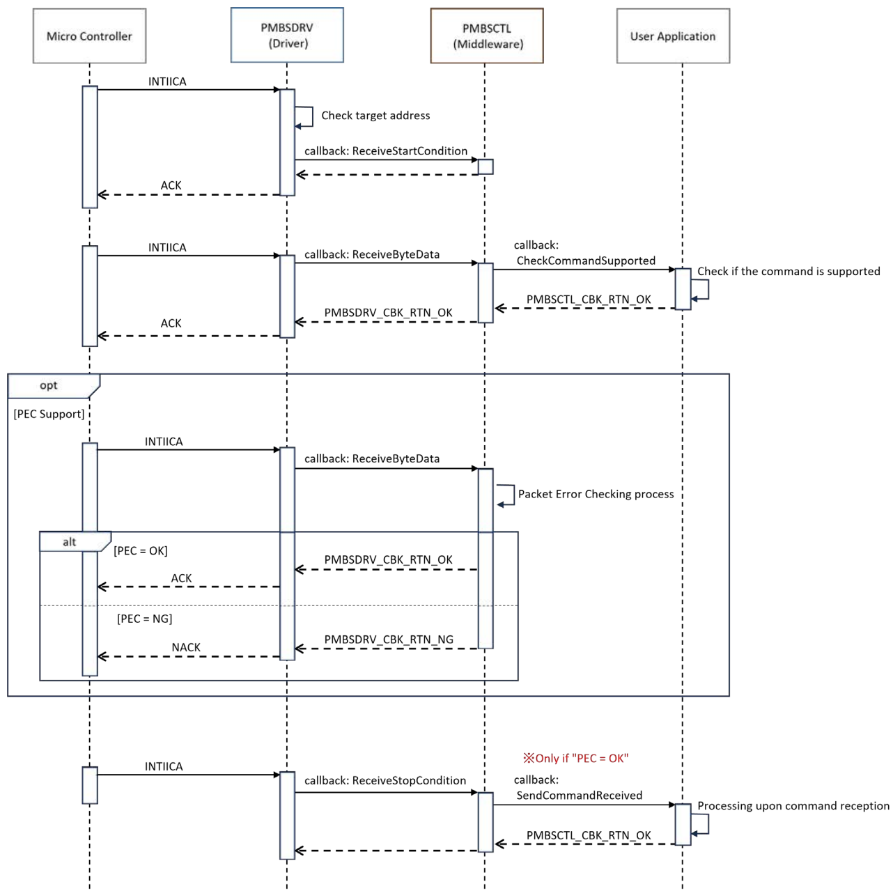
図 5-1 Send Byte sequence
