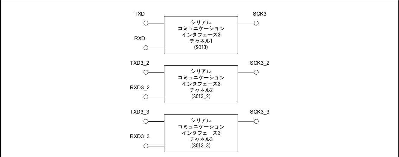
図 1.1 シリアルコミュニケーションインタフェース 3 (SCI3)のブロック図
