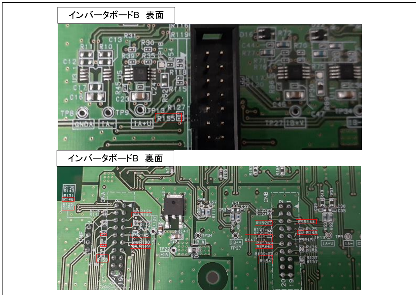
図 2-6 インバータボード B 抵抗実装
