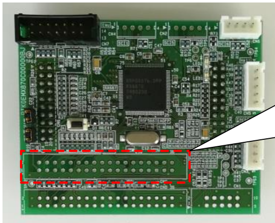
図 2-9 CPU カードピンヘッダ実装
