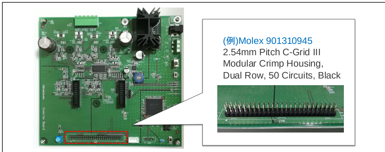
図 2-5 インバータボード B へのピンヘッダ実装
