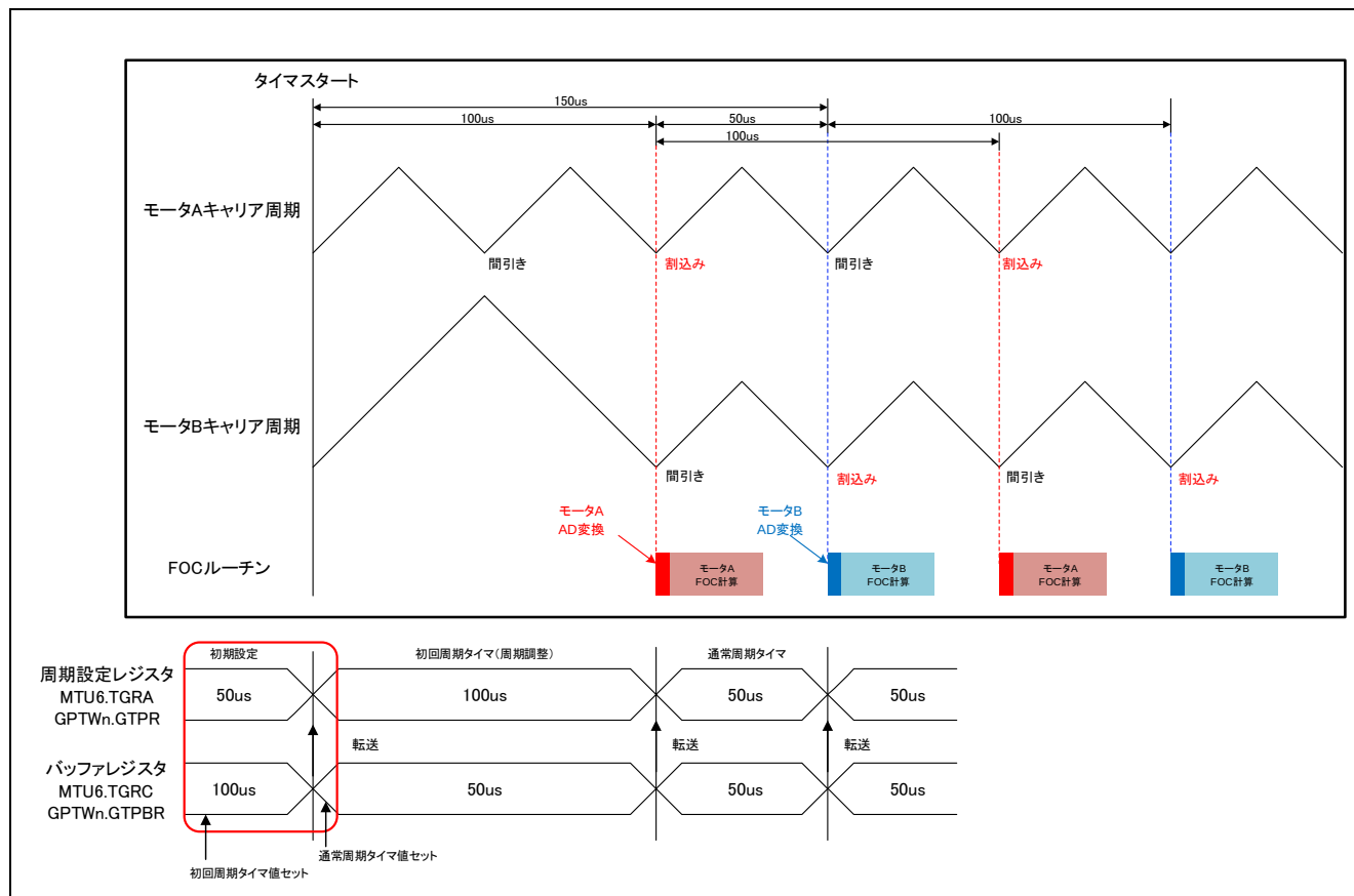
図 3-5 キャリア出力調整
