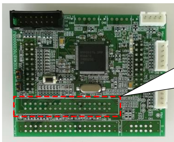
図 2-7 CPU カードピンヘッダ実装
