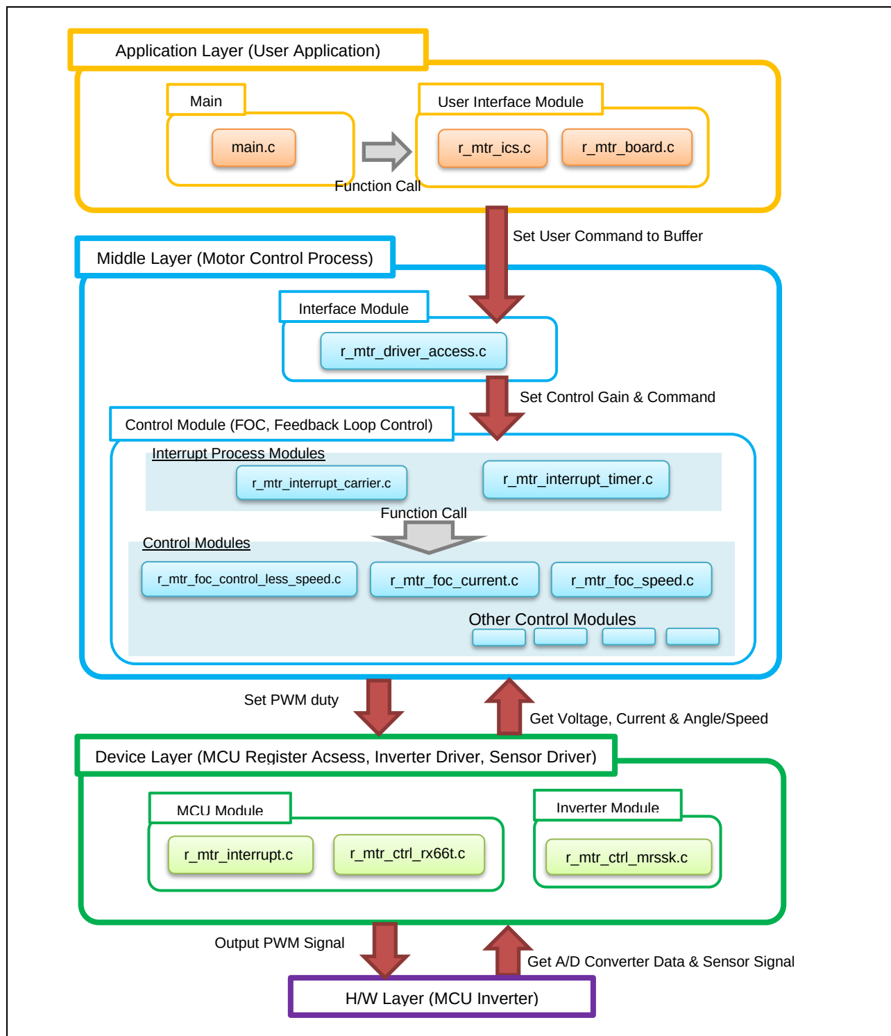
図 2-14 モジュール構成
