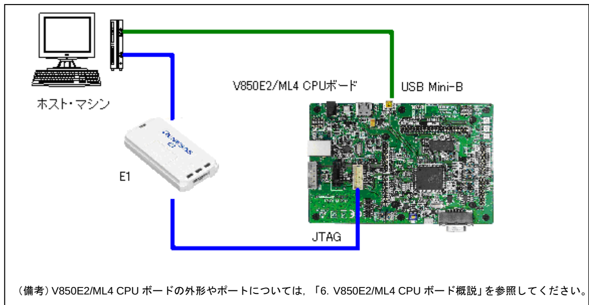
図 5-8 V850E2/ML4 CPU ボードの接続
