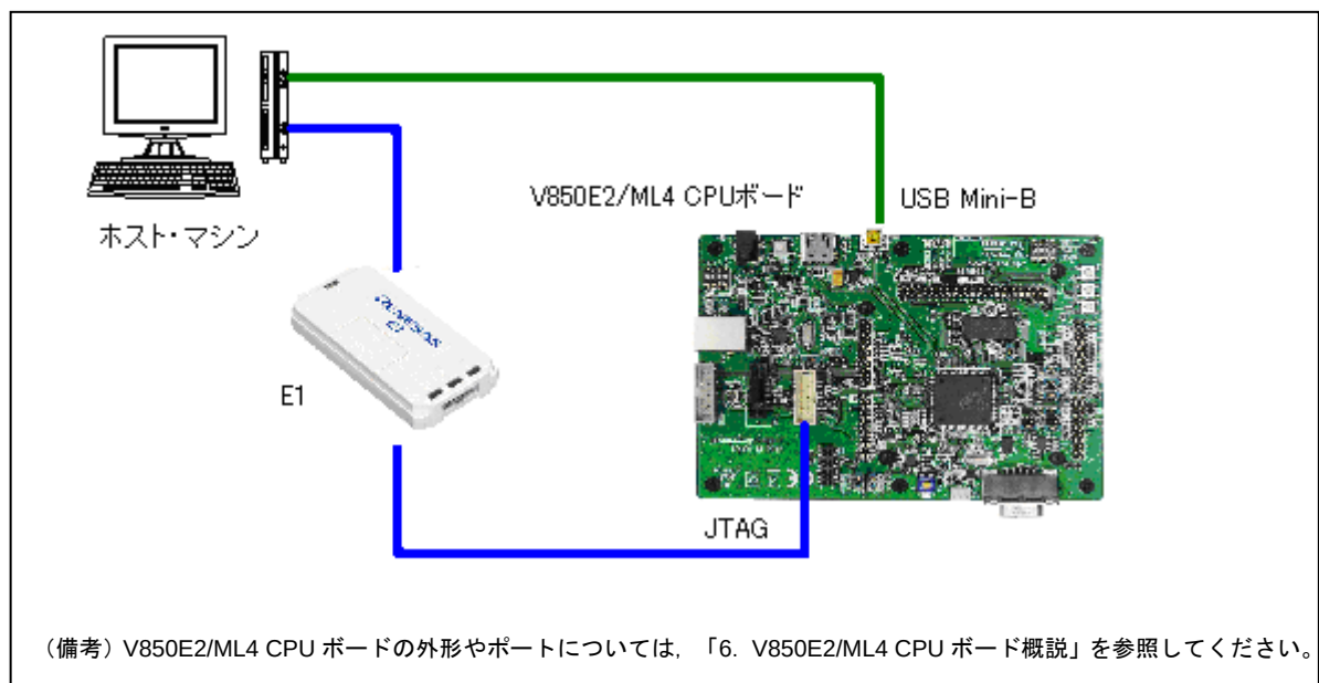
図 5-1 開発環境のシステム構成
