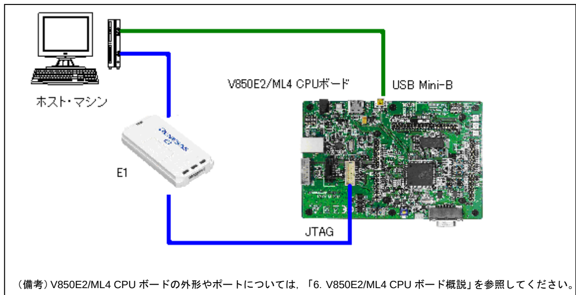
図 5-13 V850E2/ML4 CPU ボードの接続
