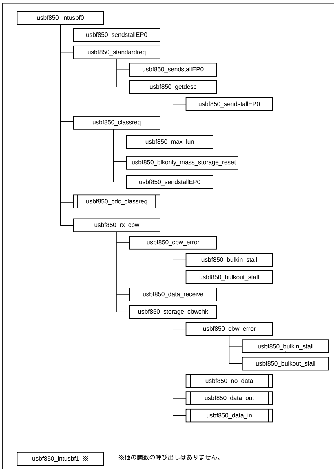
図 4-18 USB 割り込み処理での関数の呼び出し
