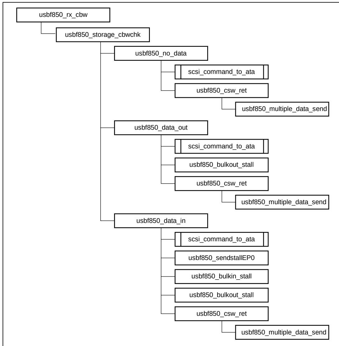
図 4-19 CBW/CSW 処理での関数の呼び出し
