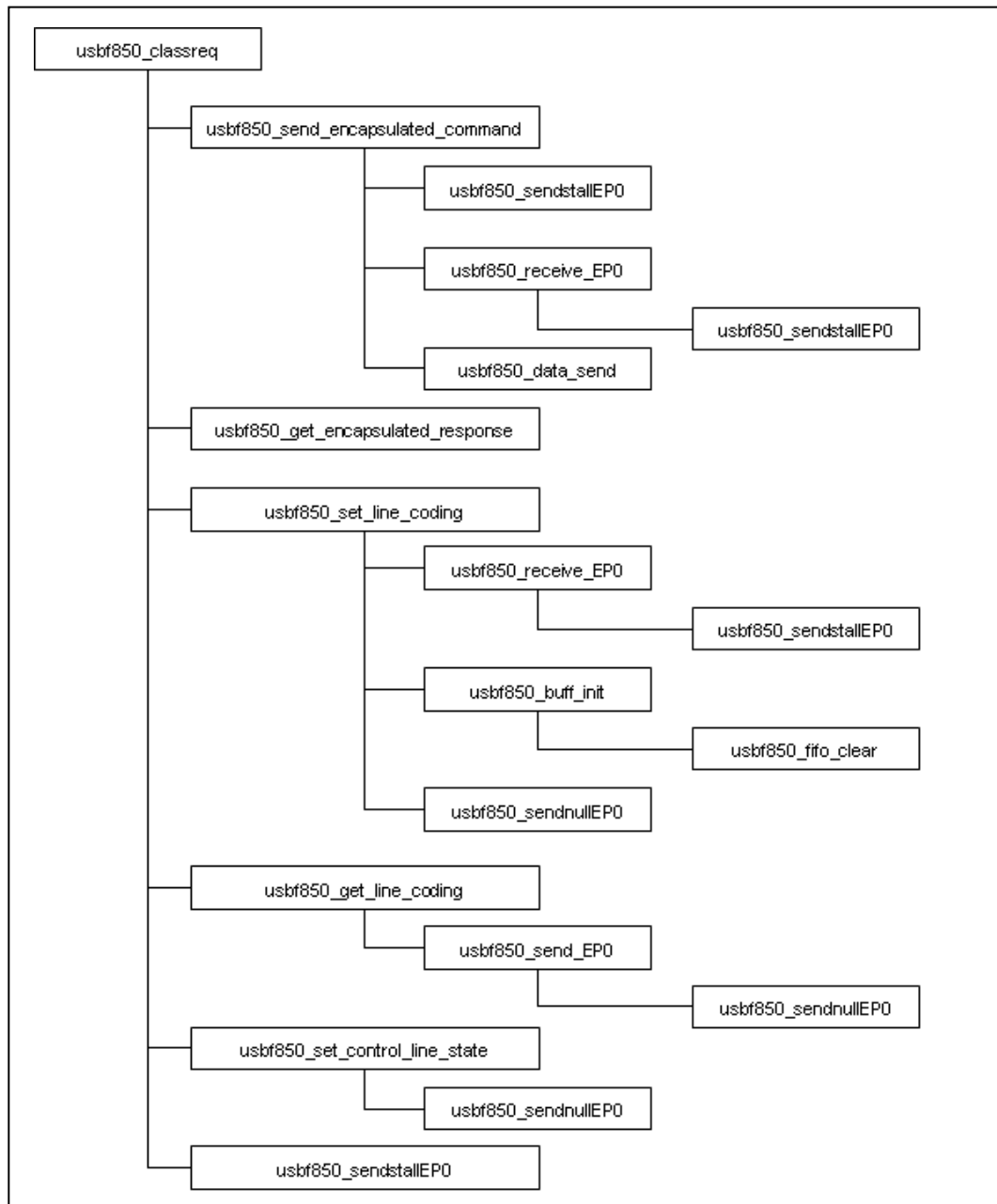
図 4-21 USB コミュニケーション・クラス用処理での関数の呼び出し(1/2)
