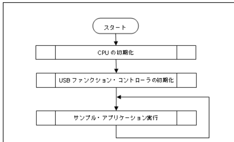
図 4-8 サンプルプログラムの処理フロー
