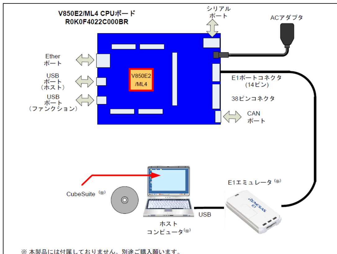
図 6-1 V850E2/ML4 CPU ボードの接続イメージ
