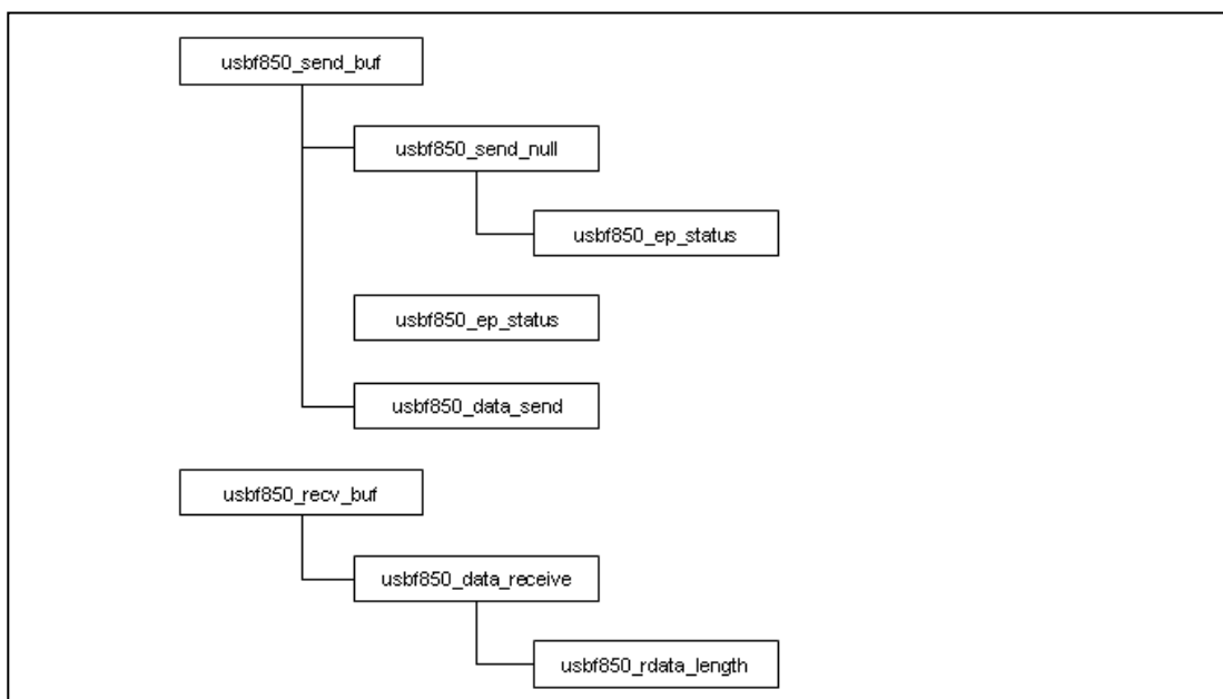
図 4-22 USB コミュニケーション・クラス用処理での関数の呼び出し(2/2)
