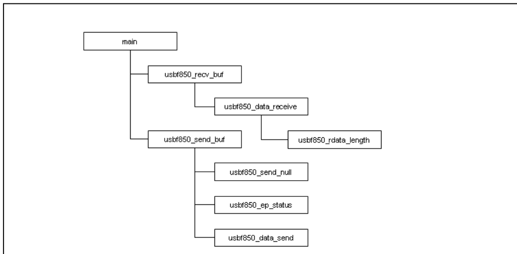
図 4-17 main 処理での関数の呼び出し
