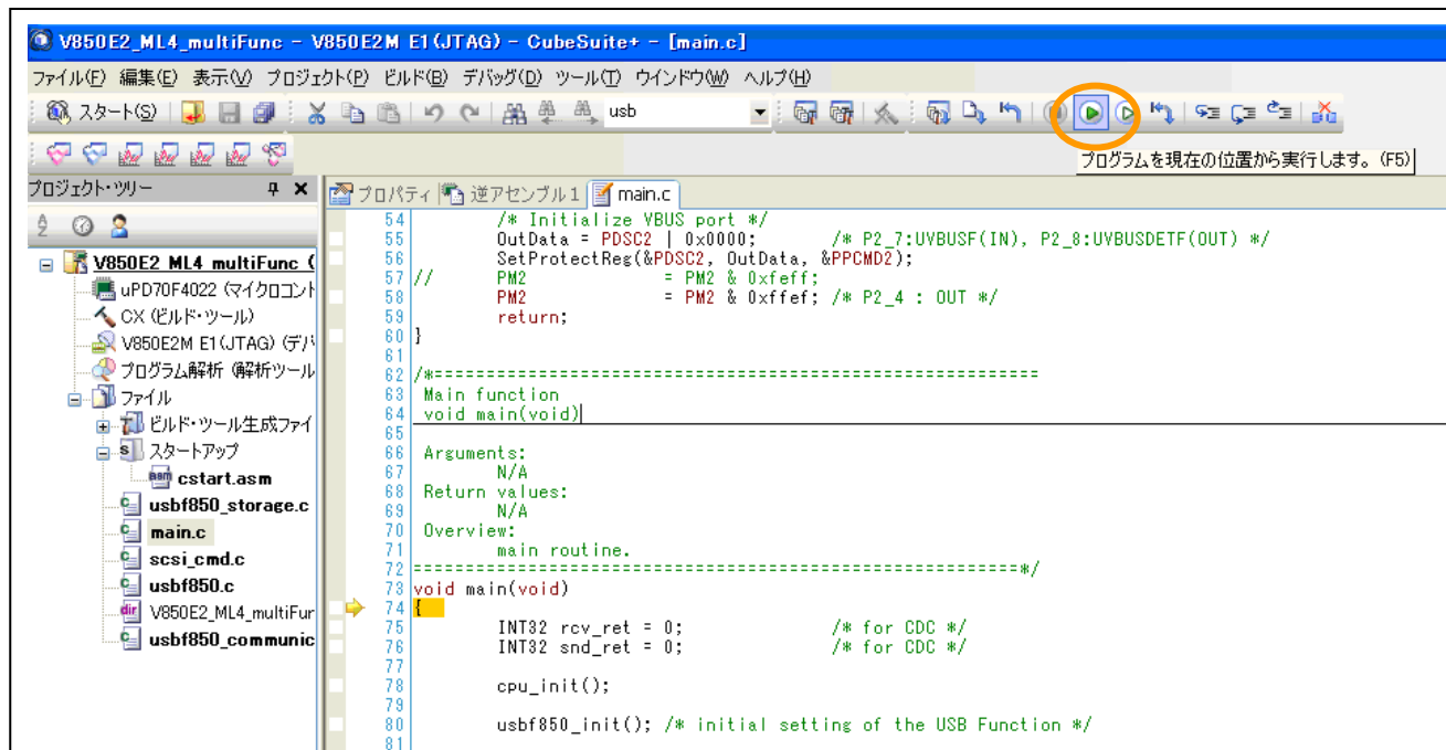
図 5-12 実行開始
