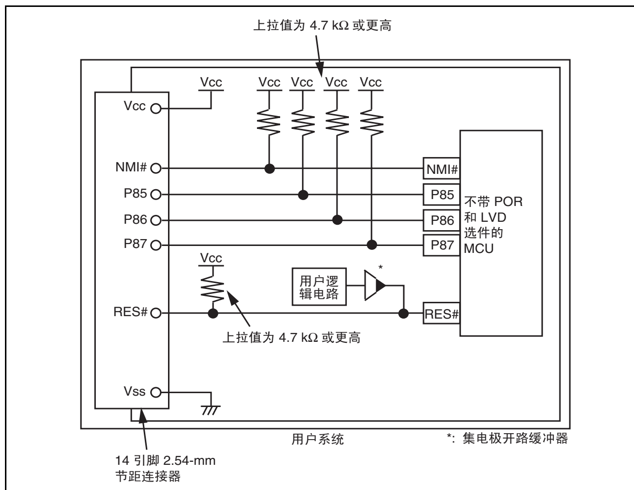
图 4.1 仿真器连接示例（不带 POR 和 LVD 选件的 MCU）
