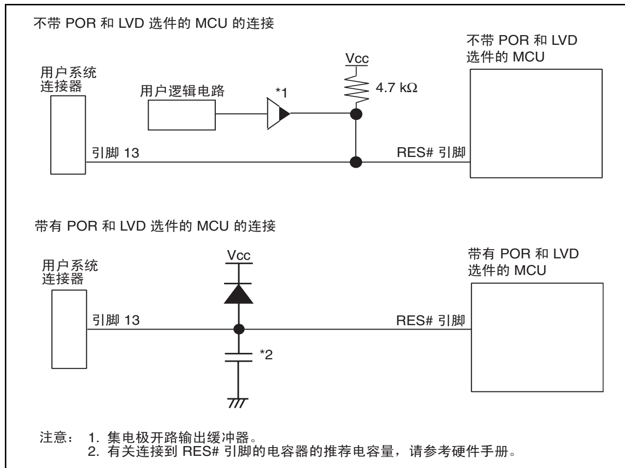
图 4.5 复位电路示例
