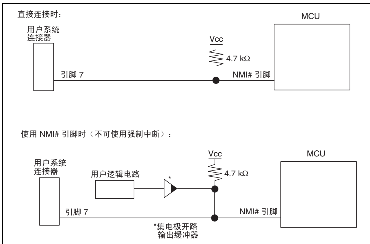
图 4.4 仿真器和 NMI# 引脚的连接
