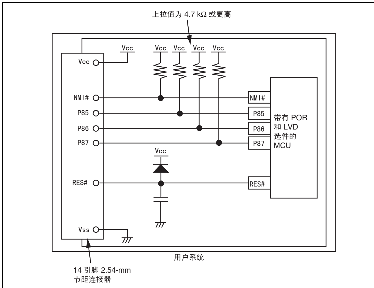
图 4.2 仿真器连接示例（带 POR 和 LVD 选件的 MCU）
