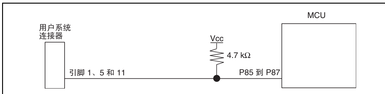
图 4.3 仿真器和 P85 到 P87 引脚的连接
