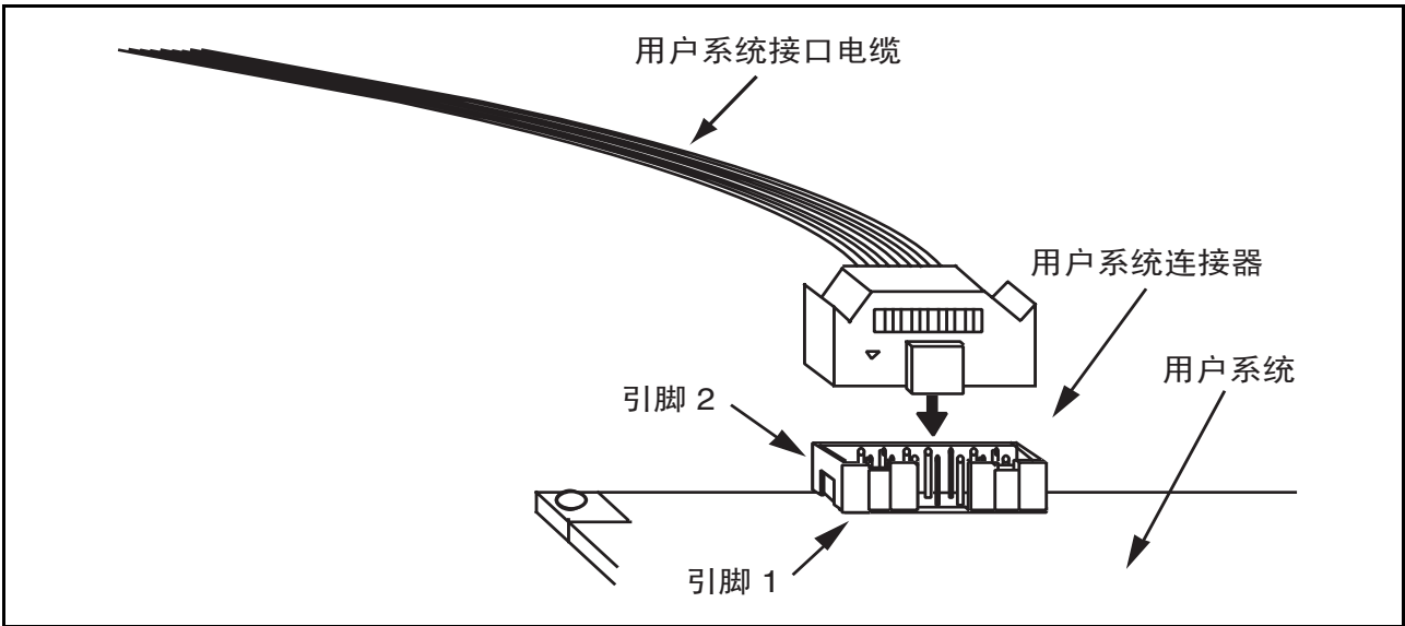
图 2.1 将用户系统接口电缆连接到用户系统
