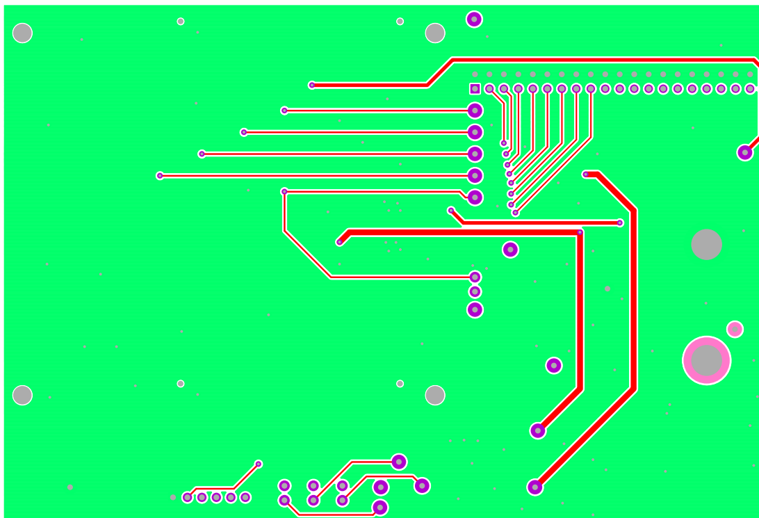
Figure 24. Bottom Layer
