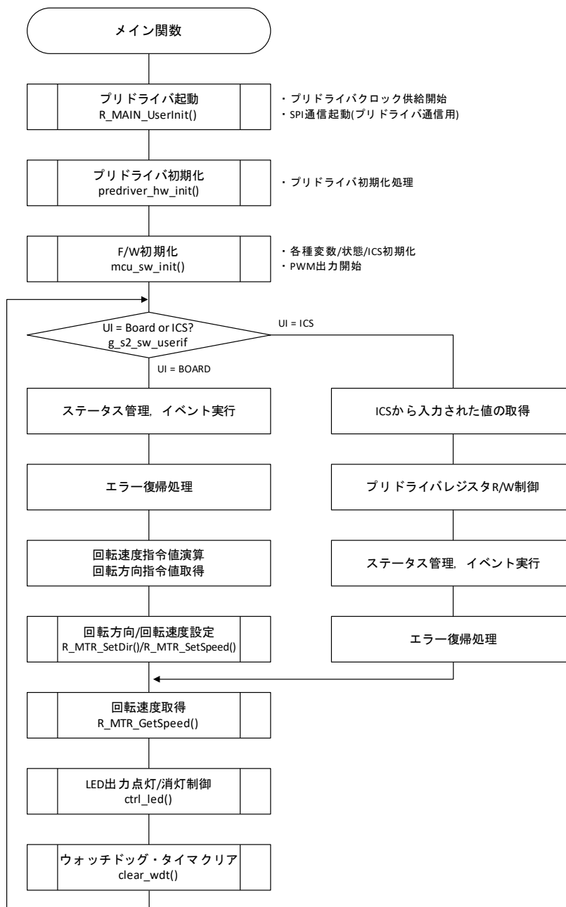
Figure 3-7 フローチャート(メイン関数)
