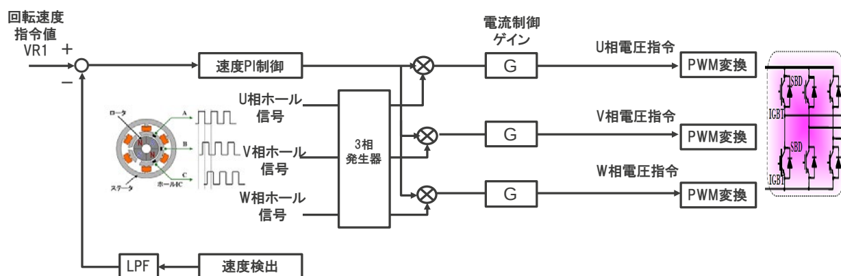
Figure 2-5 ソフトウェアの基本仕様
