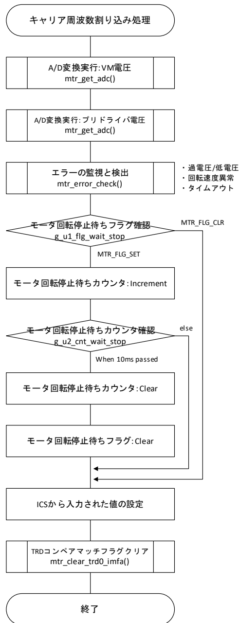
Figure 3-10 フローチャート(キャリア周波数割り込み処理)
