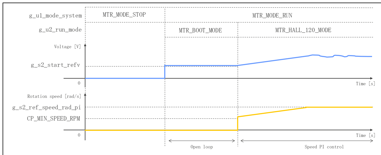
Figure 3-5 始動方法
