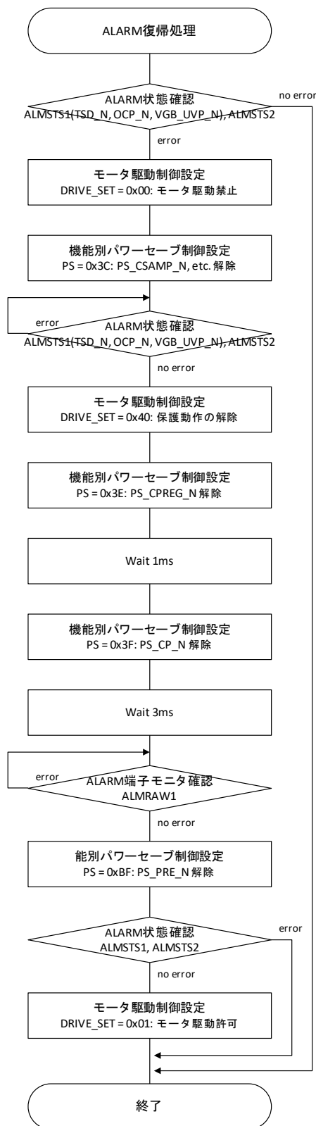
Figure 3-13 フローチャート(ALARM 復帰処理)
