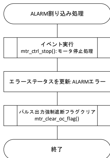
Figure 3-12 フローチャート(ALARM 割り込み処理)
