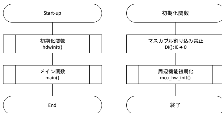
Figure 3-6 フローチャート(全体、初期化関数)
