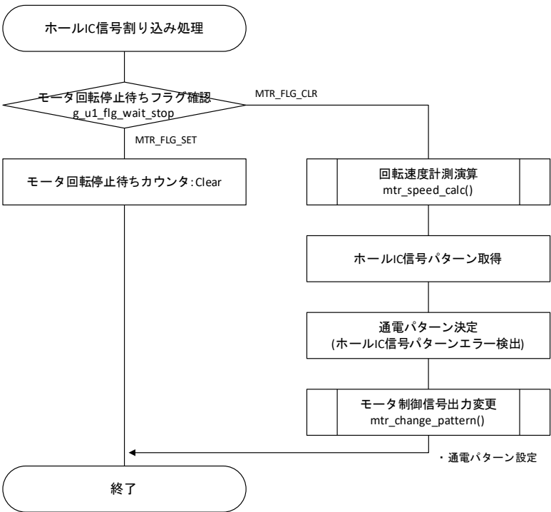
Figure 3-9 フローチャート(ホール IC 信号割り込み処理)
