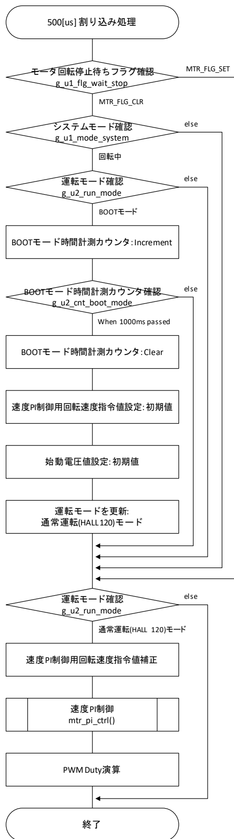
Figure 3-11 フローチャート(500[us] 割り込み処理)
