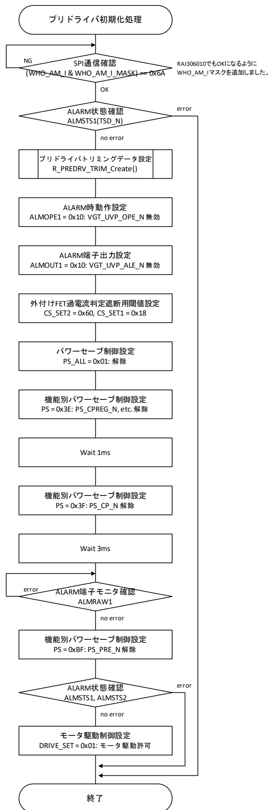
Figure 3-8 フローチャート(プリドライバ初期化処理)
