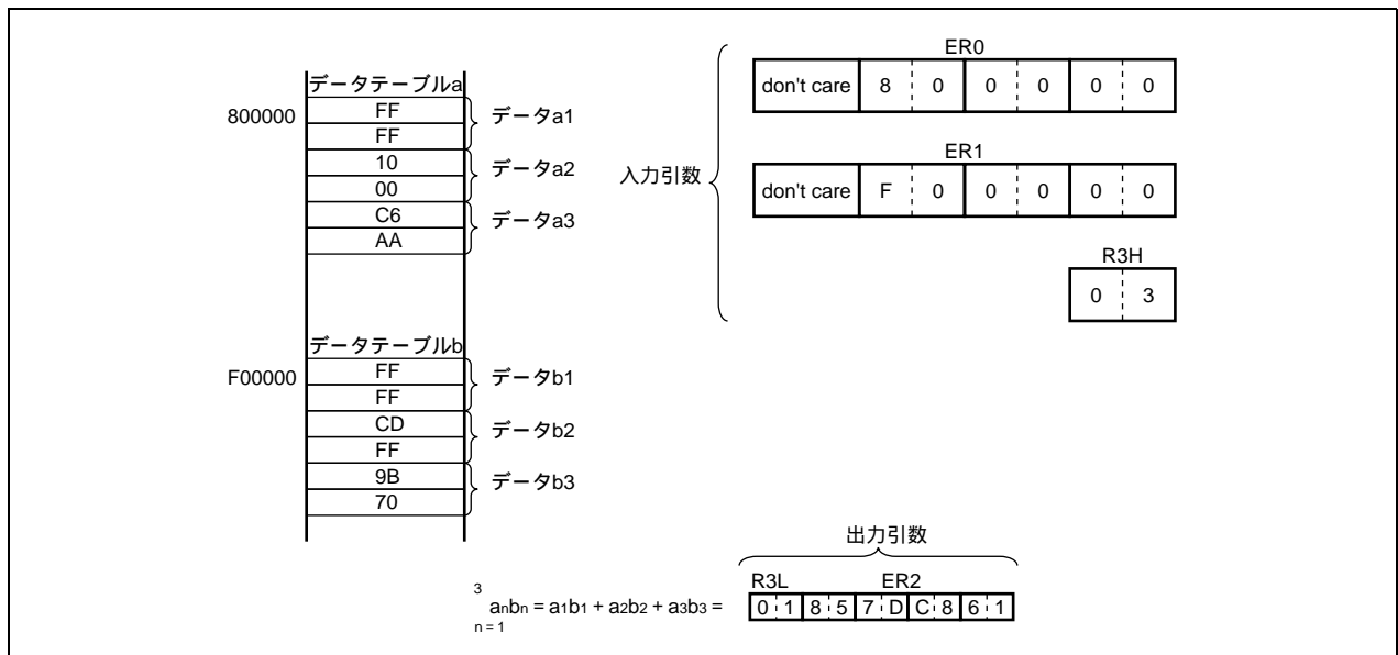
図 5.1 ソフトウェア SEKIWA の実行例
