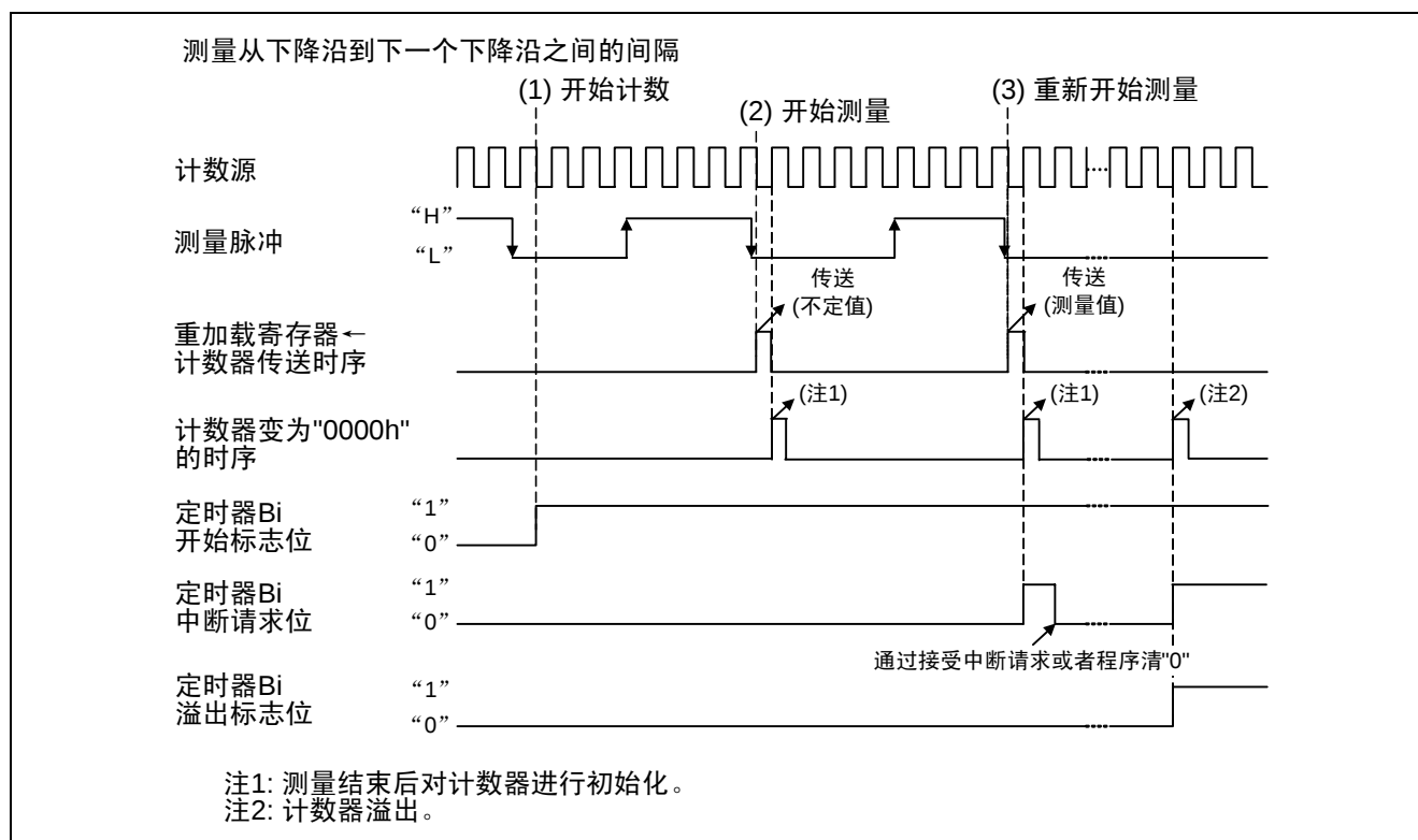
图 1. 脉冲周期测量模式工作时序图
