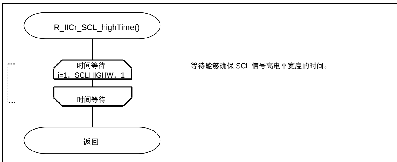
图 5.38 SCL 高电平时间等待处理
