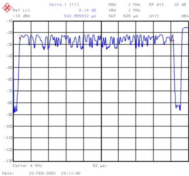
FIGURE 28. EDGE FRAME TIMING
