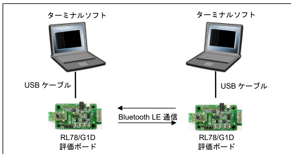
図 1-1 アプリケーション使用時の構成図
