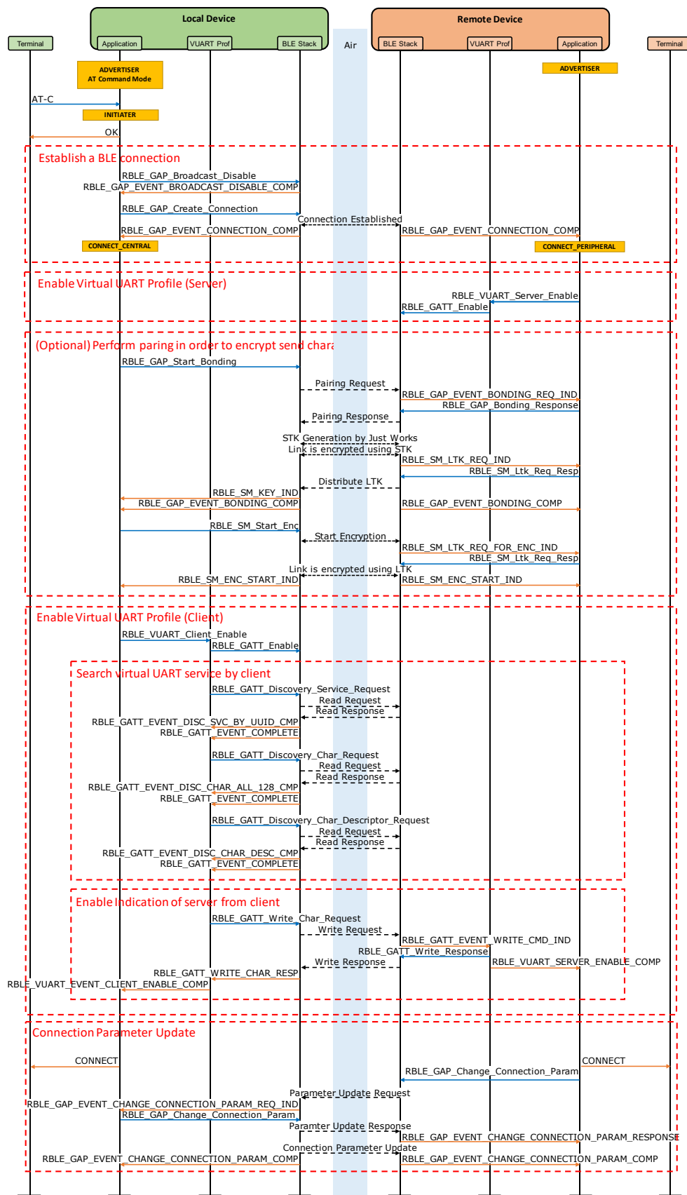
図 8-3 接続シーケンス
