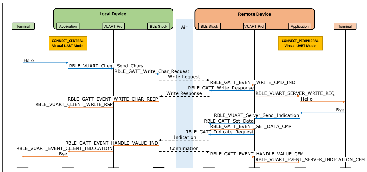
図 8-4 データ送受信シーケンス(Write Request/Indication)
