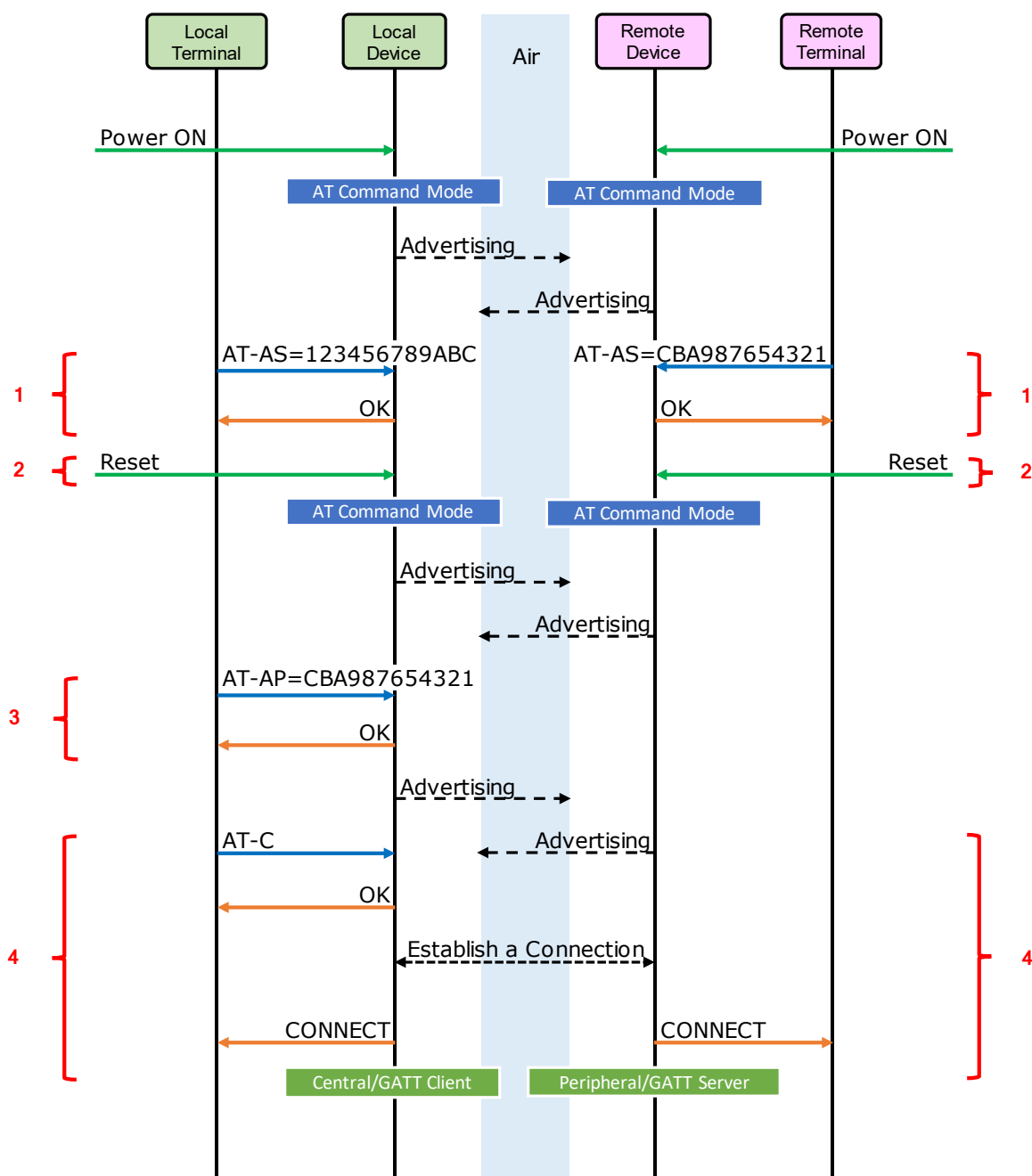
図 7-2 文字データ送受信 実行例のシーケンス (1/2)
