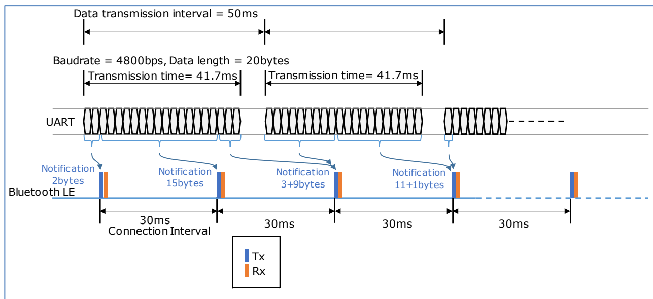
図 8-8 ターミナルからのデータ受信と Notification 通信例
