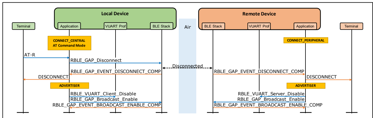
図 8-6 切断シーケンス
