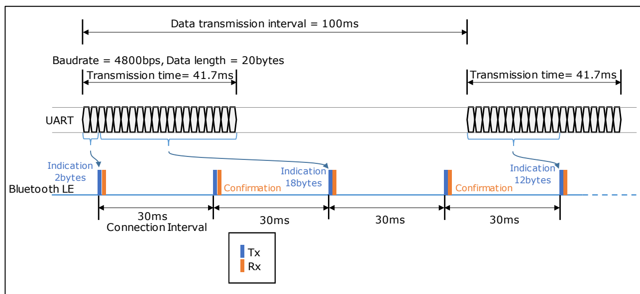
図 8-7 ターミナルからのデータ受信と Indication 通信例
