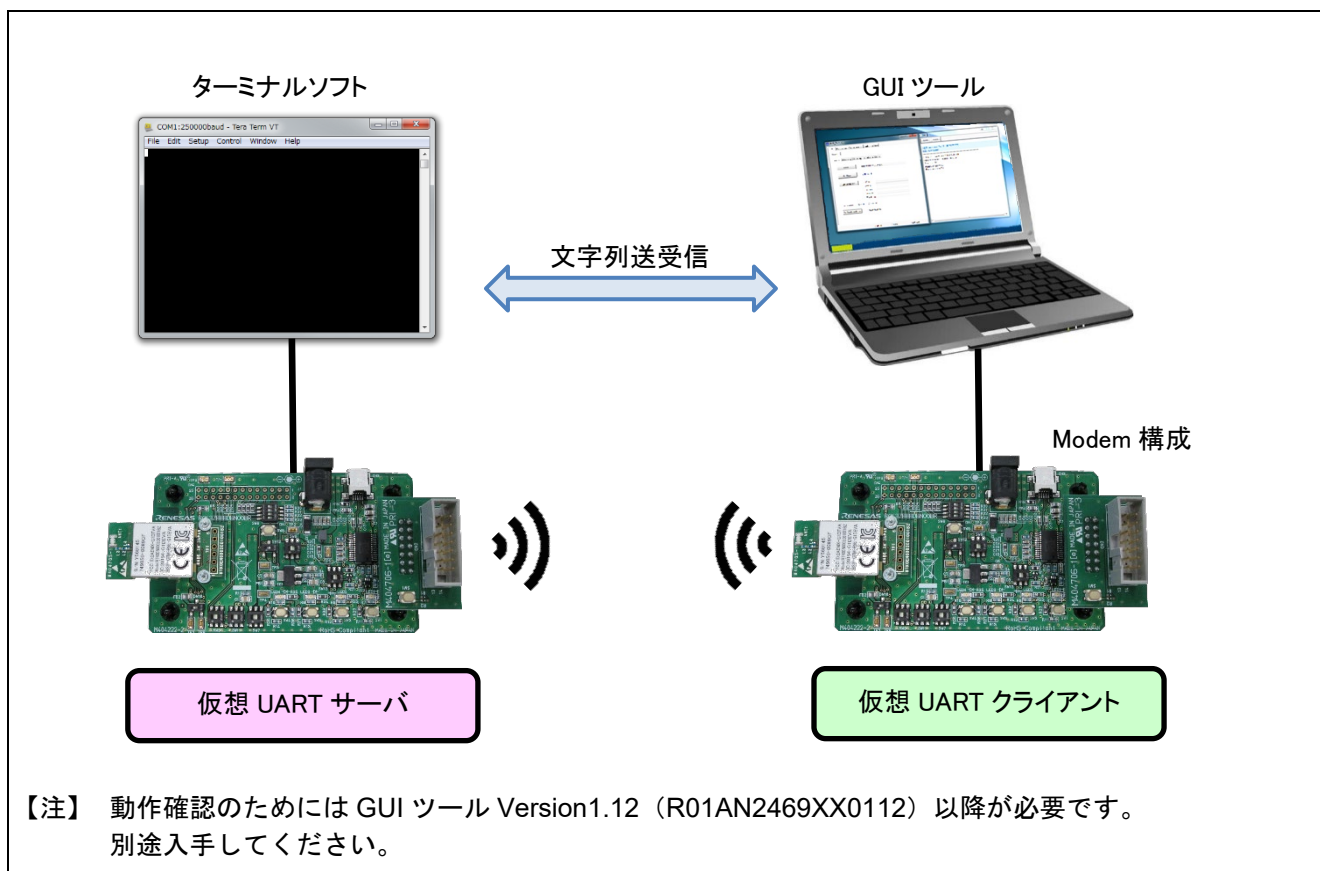
図 9-1 GUI ツールを使用した動作確認構成
