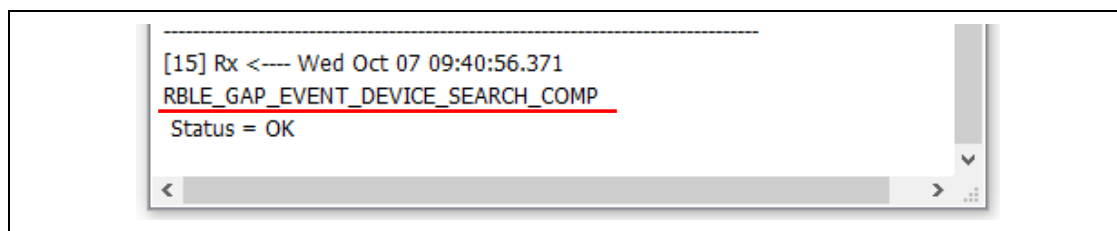
図 9-4 RBLE_GAP_EVENT_DEVICE_SEARCH_COMP イベントの確認
