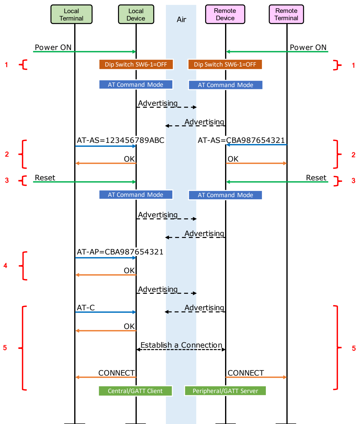
図 7-5 バイナリデータ送受信 実行例のシーケンス (1/2)
