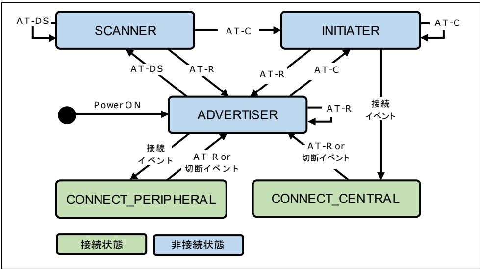
図 8-1 アプリケーションの状態遷移図
