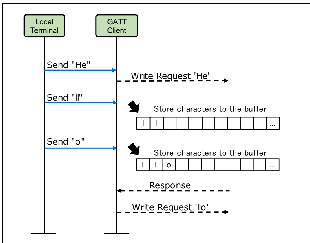
図 5-3 送信データのバッファリング (レスポンス有り)
