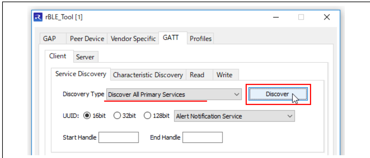
図 9-9 サービス検索
