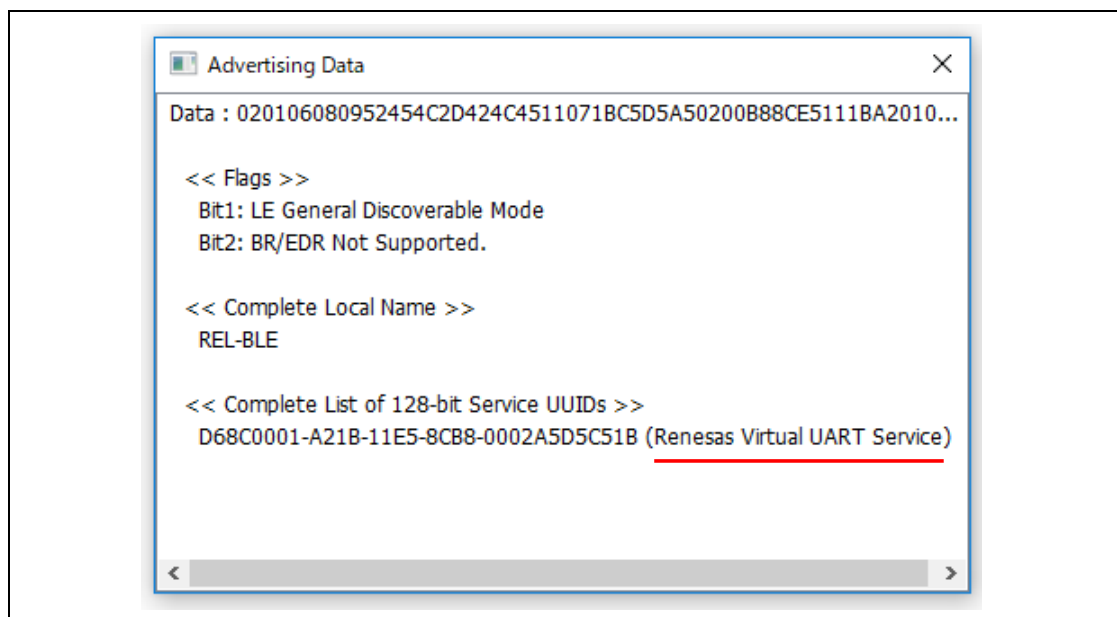
図 9-6 Advertising データ解析表示
