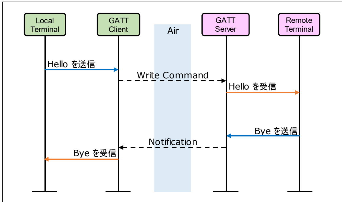
図 5-2 データの送受信時のシーケンス (レスポンス無し)
