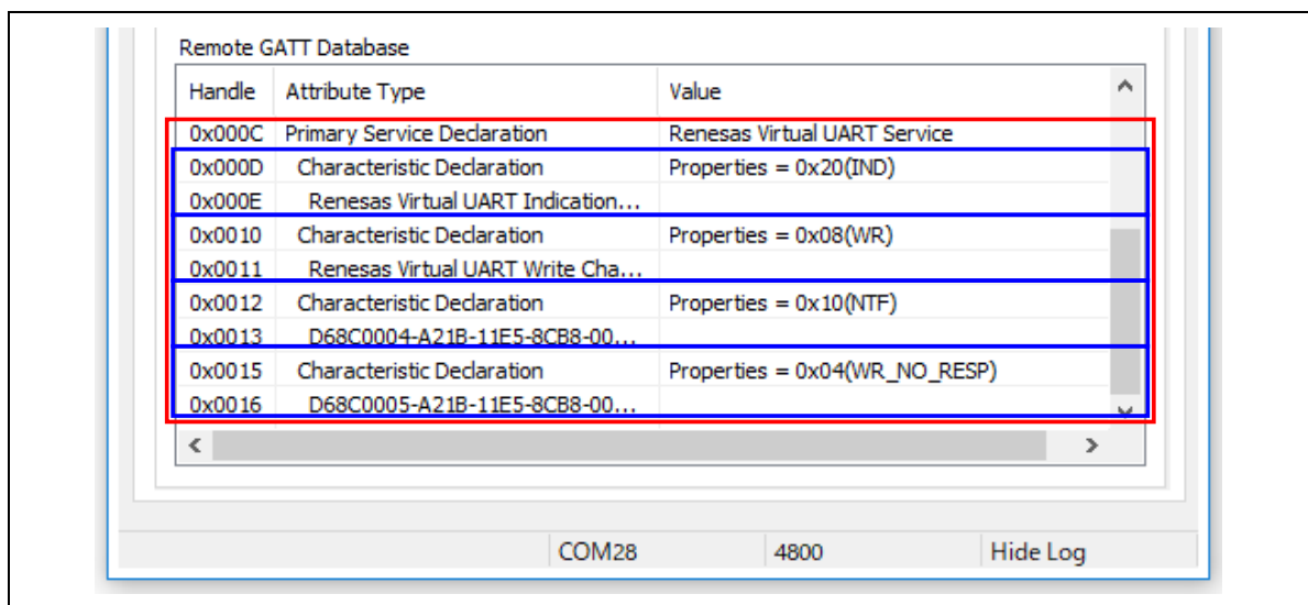
図 9-12 キャラクタリスティック検索結果
