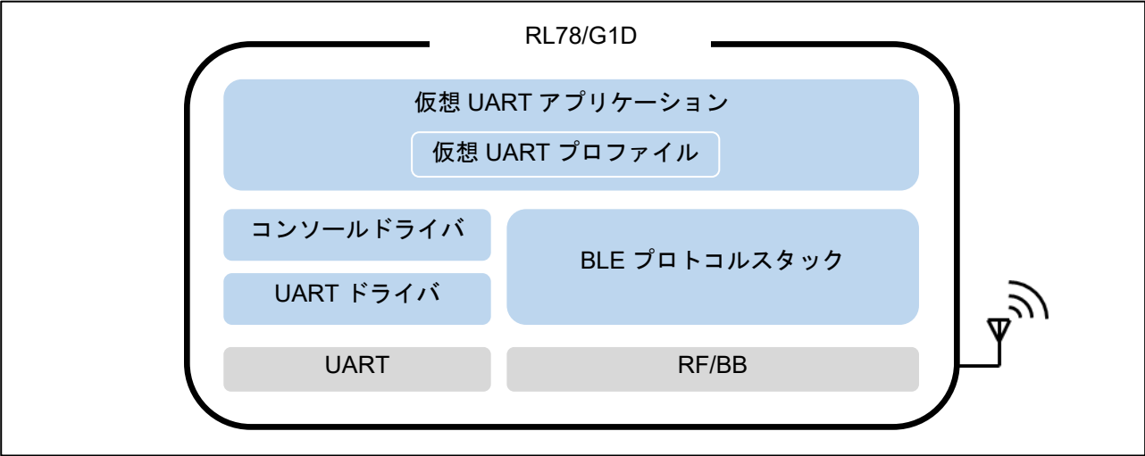
図 2-1 ソフトウェアの構成
