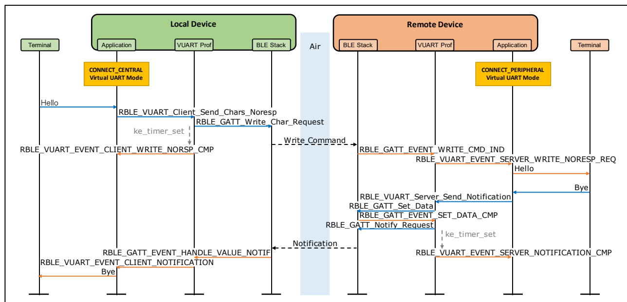
図 8-5 データ送受信シーケンス(Write Command/Notification)
