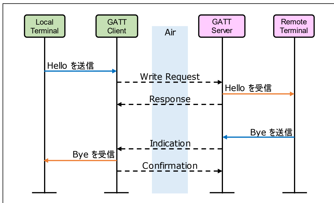
図 5-1 データ送受信時のシーケンス (レスポンス有り)
