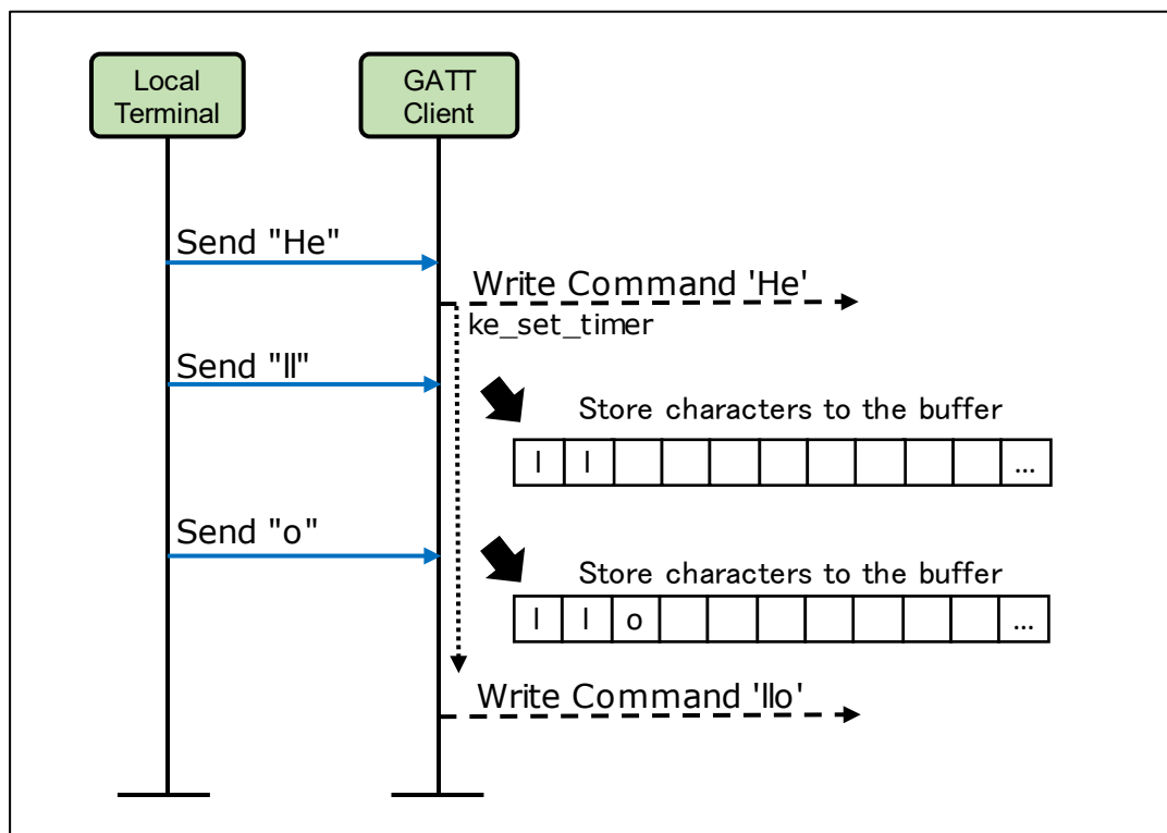
図 5-4 送信文字のバッファリング (レスポンス無し)
