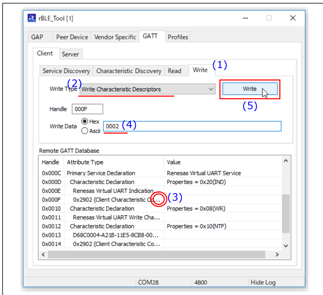
図 9-15 Indication の有効化
