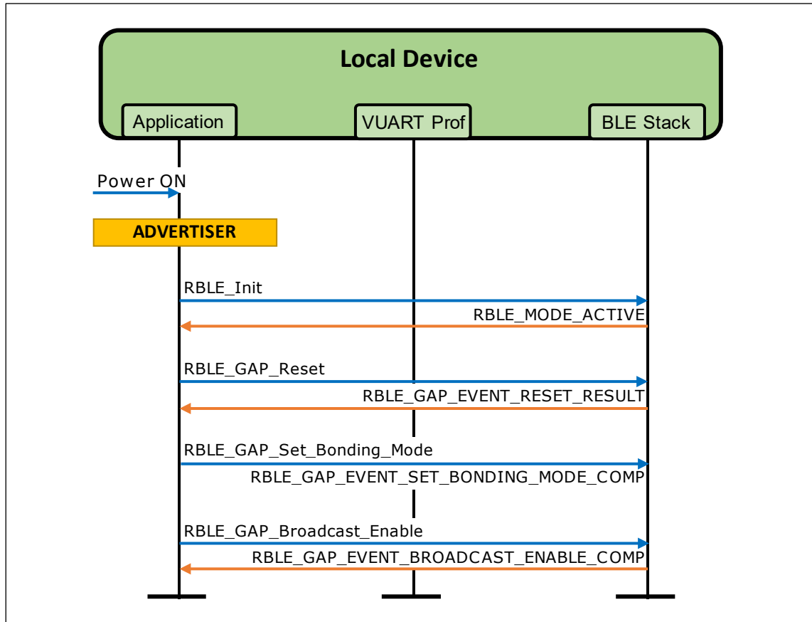
図 8-2 起動シーケンス
