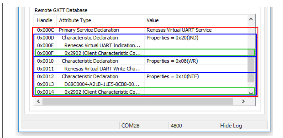
図 9-14 ディスクリプタ検索結果
