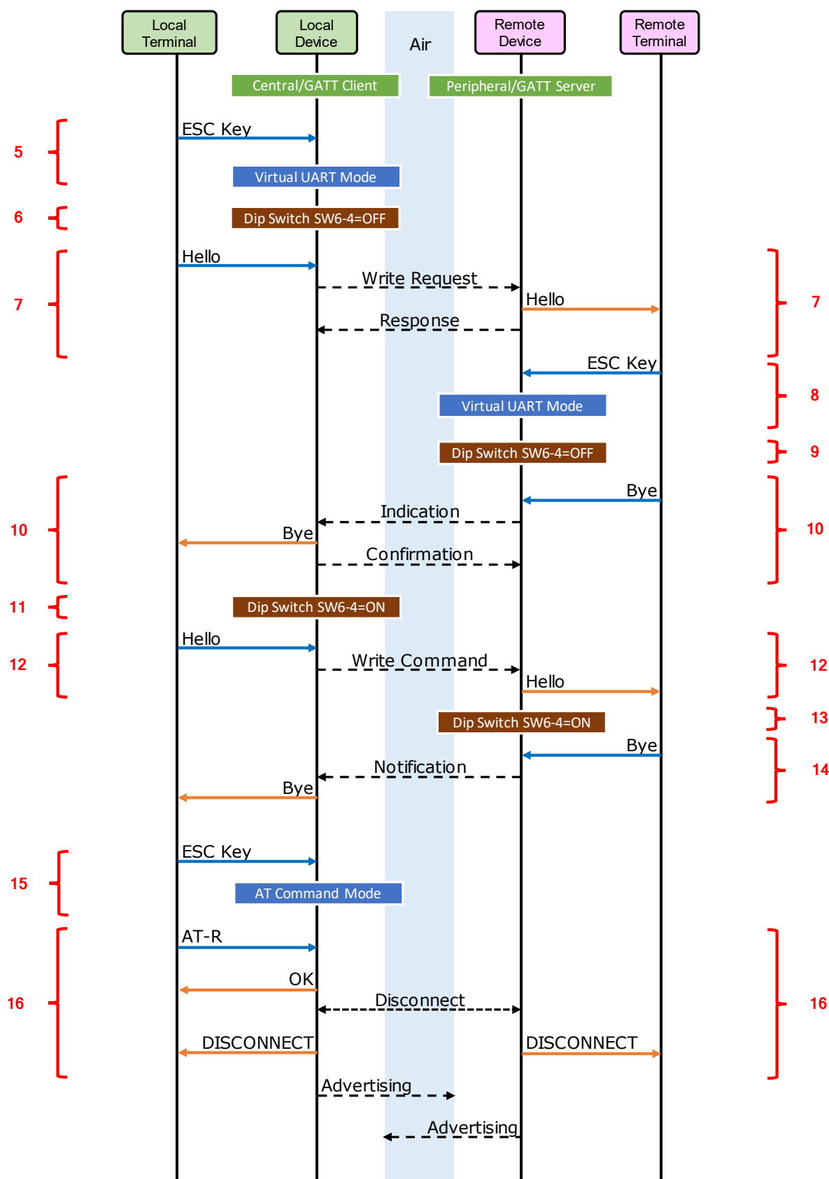
図 7-3 文字データ送受信 実行例のシーケンス (2/2)
