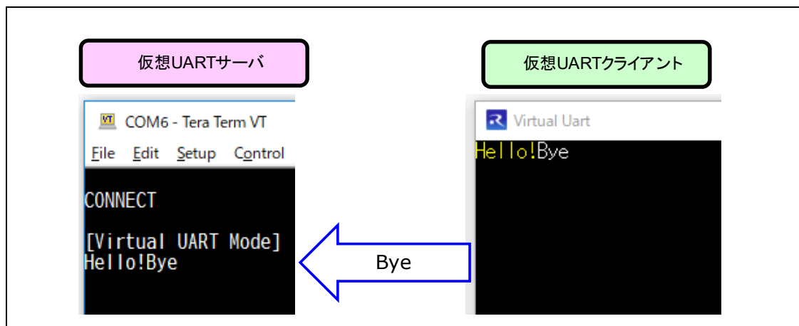
図 9-20 文字列送信（クライアント→サーバ）
