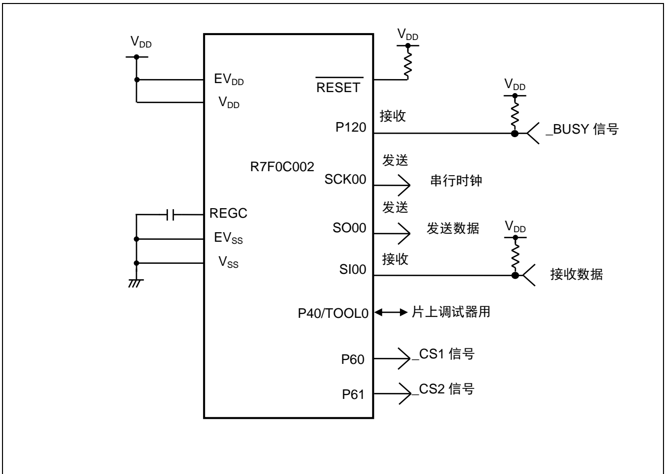
图 4.1 硬件配置
