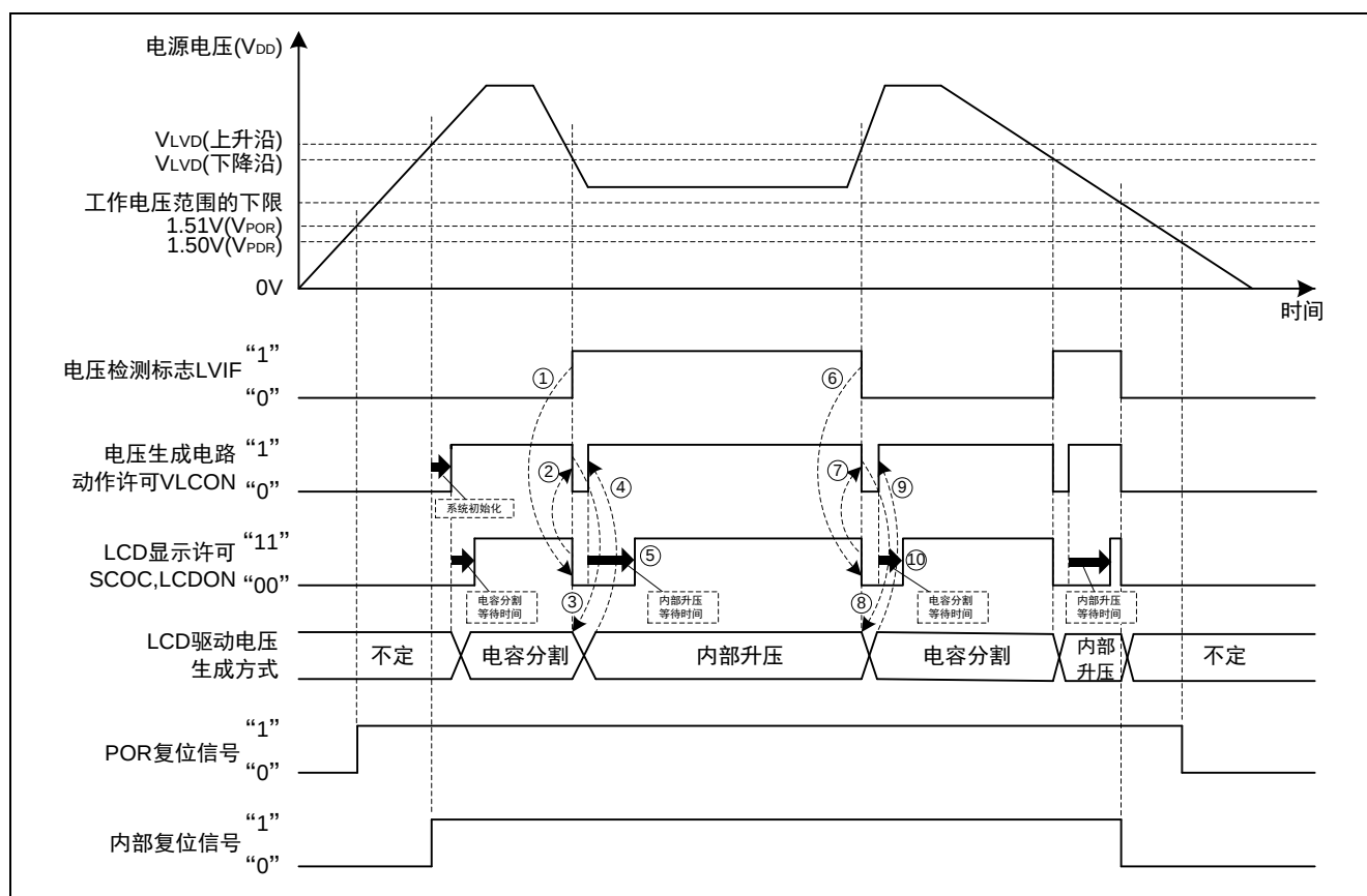
图 1.2 LCD 驱动电压生成方式根据电源电压 V_{DD} 变化的切换时序
