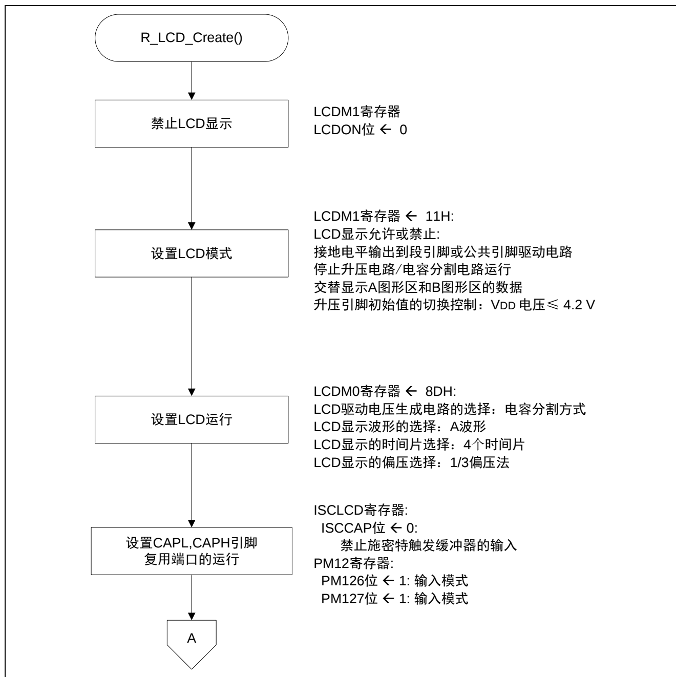
图 5.5 LCD 控制器/驱动器的初始设置 (1/2)
