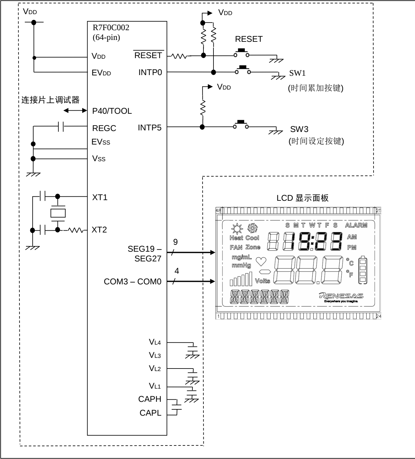
图 4.1 硬件配置
