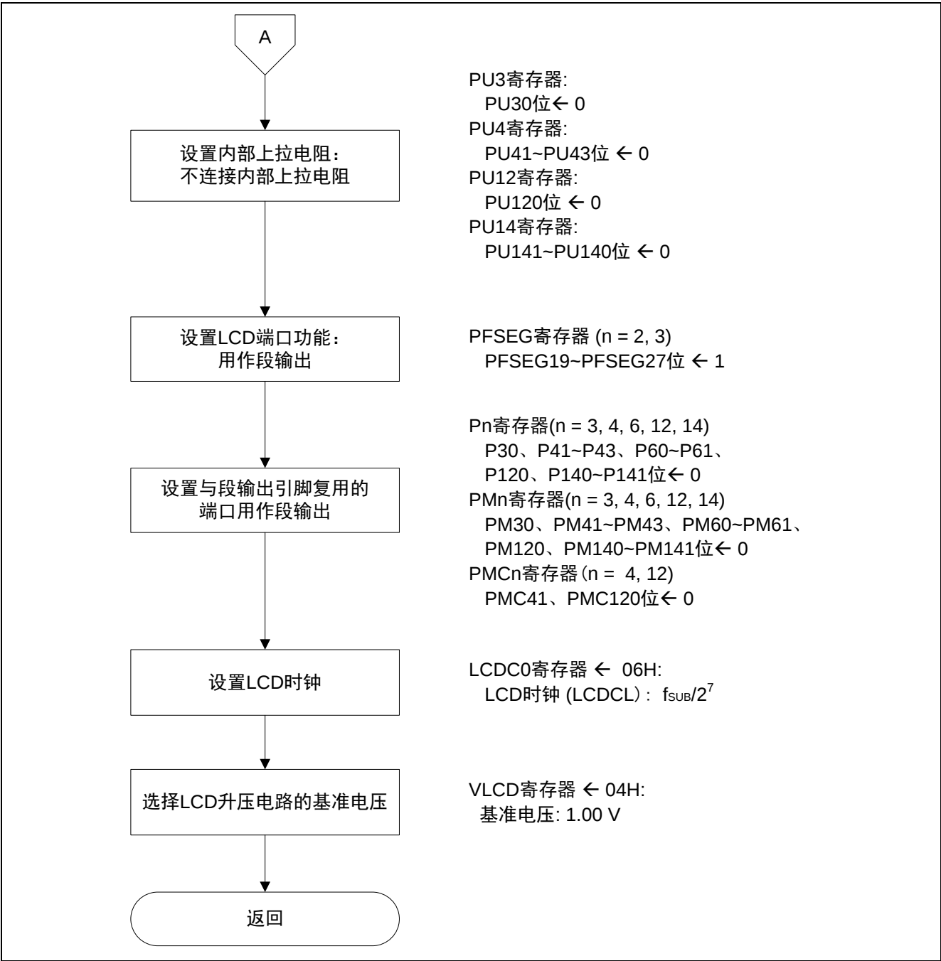
图 5.6 LCD 控制器/驱动器的初始设置 (2/2)
