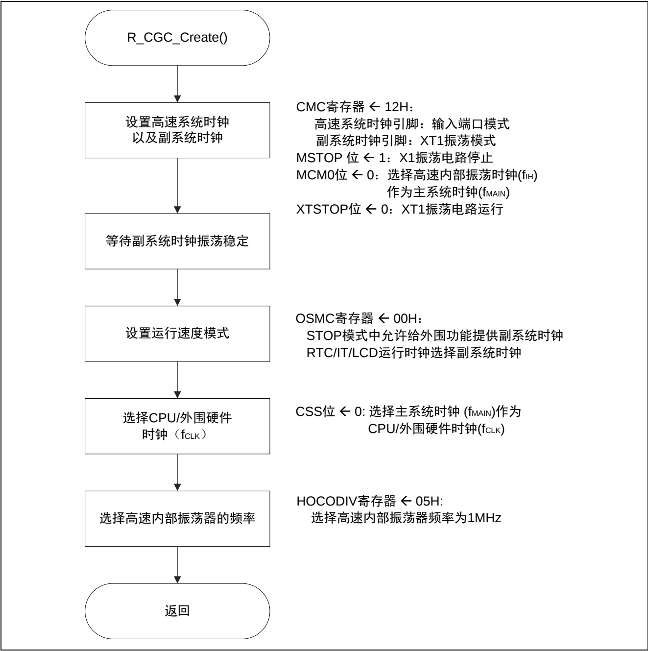
图 5.4 CPU 时钟的初始设置
