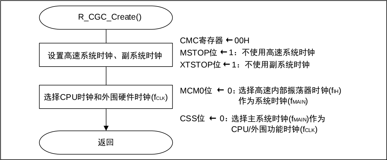
图 4.5 CPU 时钟设置
