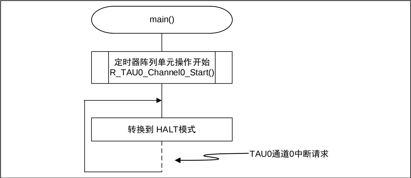
图 4.8 主函数处理
