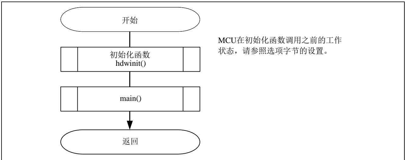
图 4.1 整体流程图
