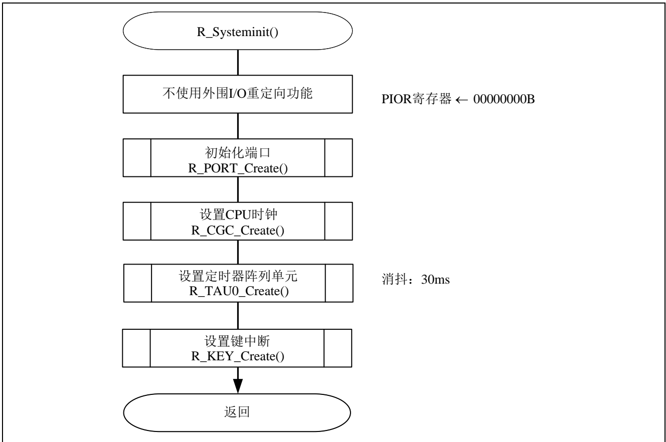
图 4.3 系统函数
