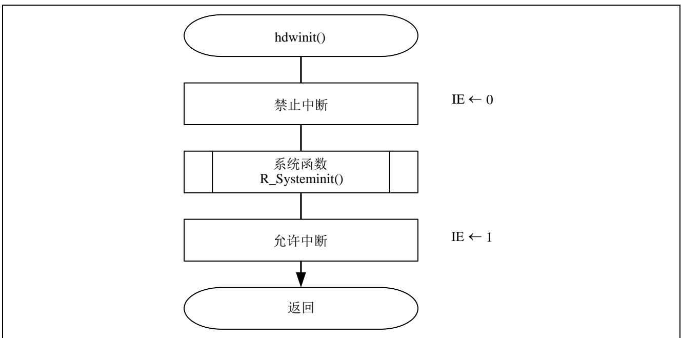
图 4.2 初始化函数
