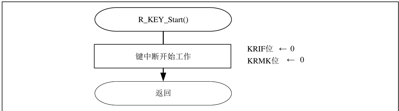
图 4.10 允许键中断
