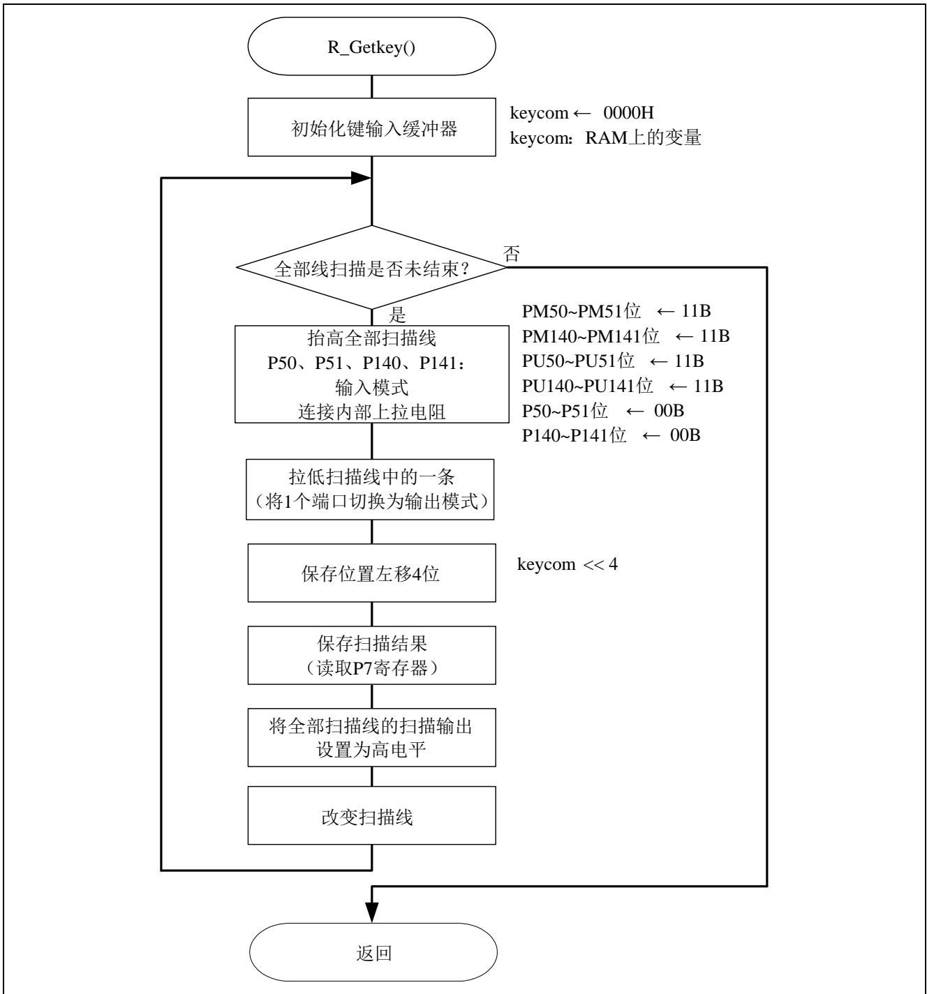
图 4.11 检测键中断
