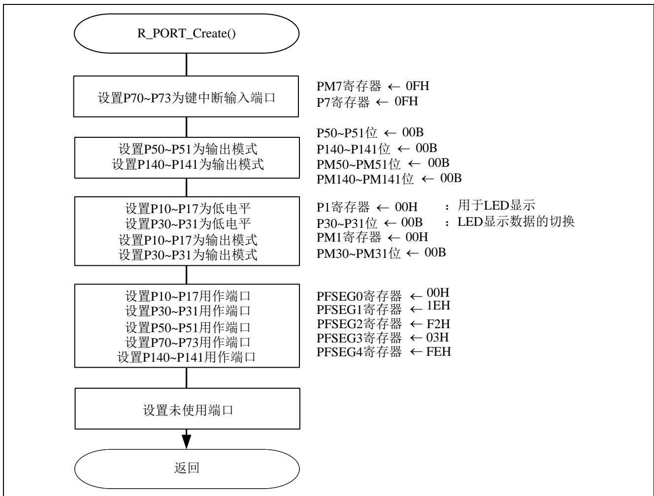
图 4.4 初始化端口
