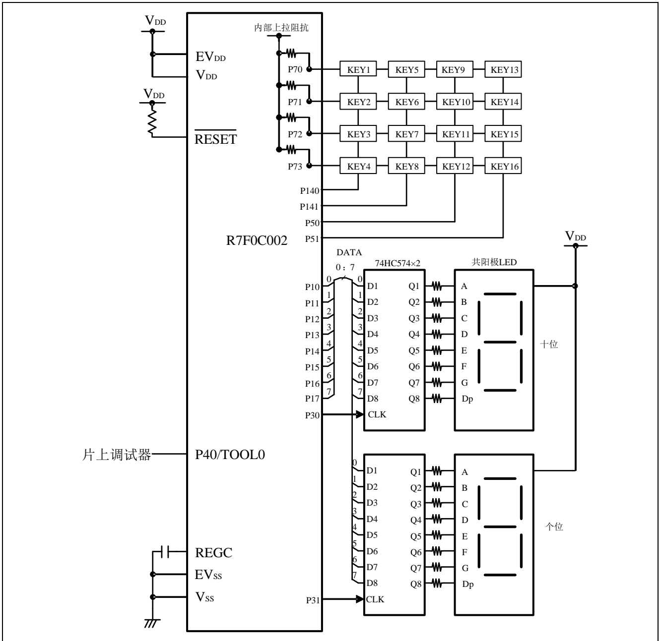
图 3.1 硬件配置
