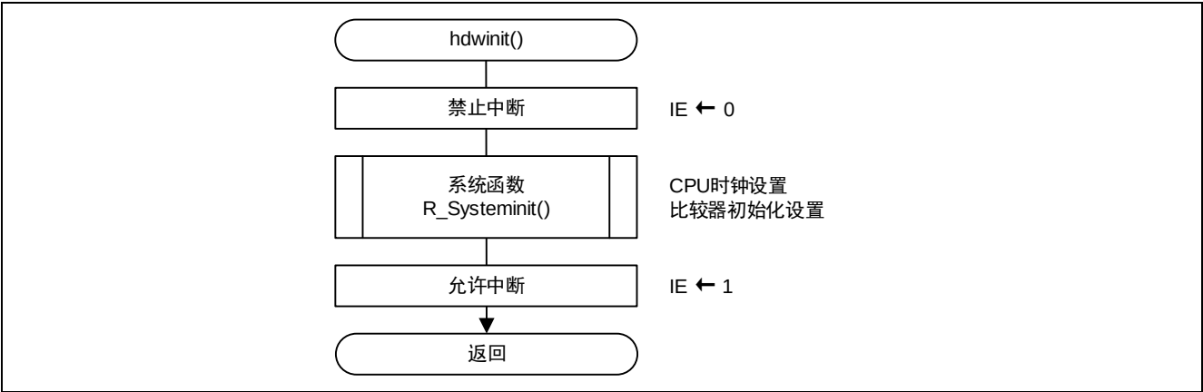
图 4.2 初始化函数
