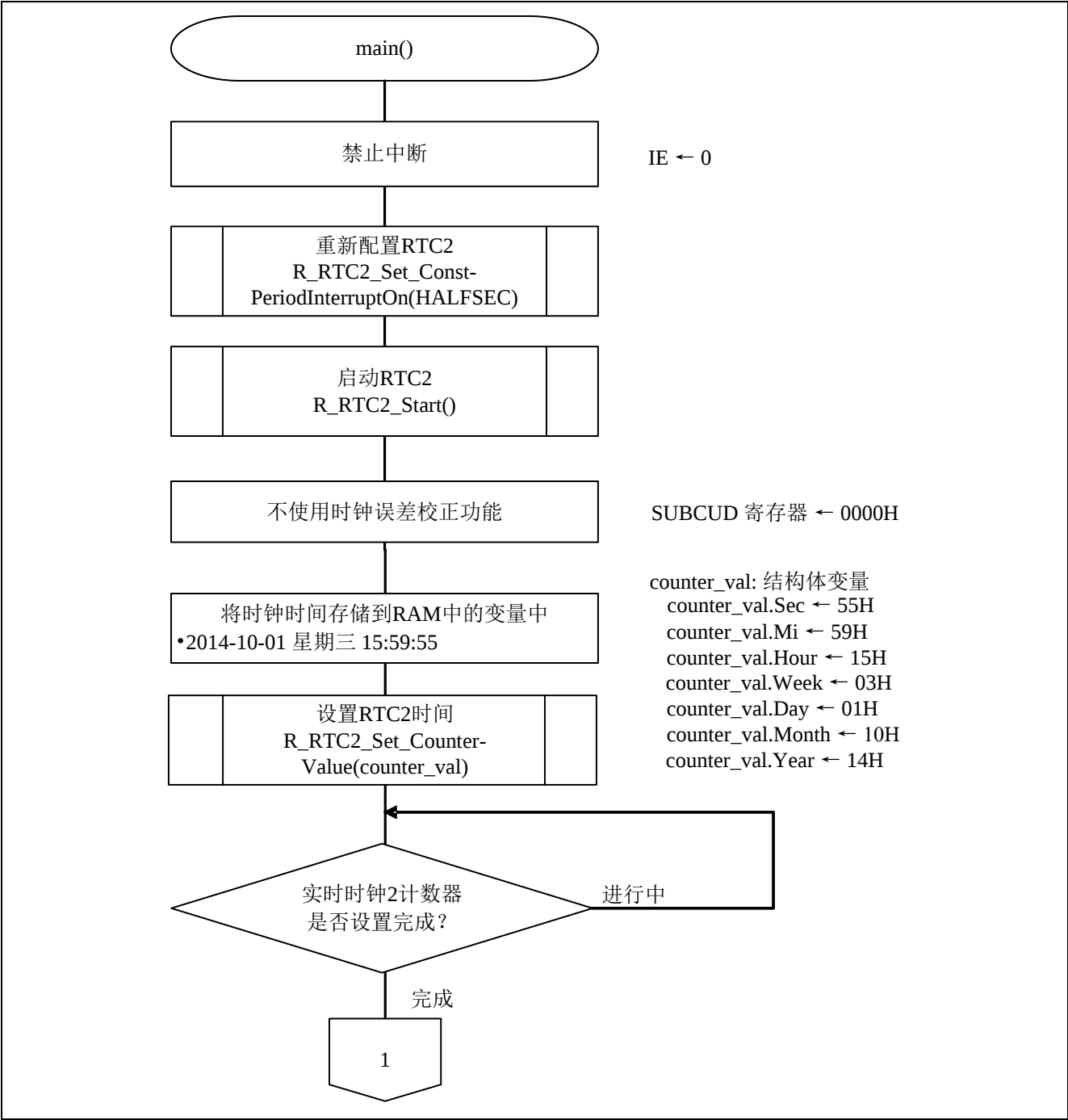
图 4.7 主函数处理 (1/2)
