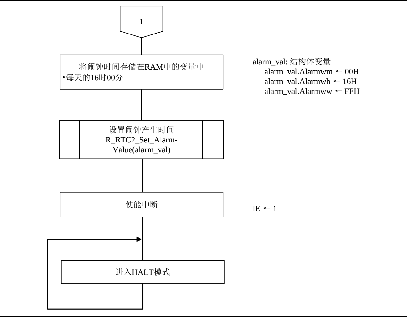
图 4.8 主函数处理（2/2）
