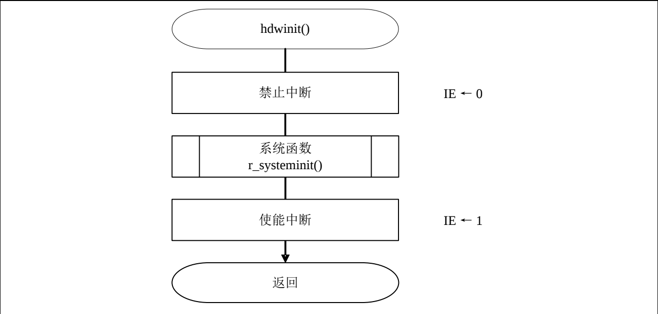
图 4.2 初始化函数
