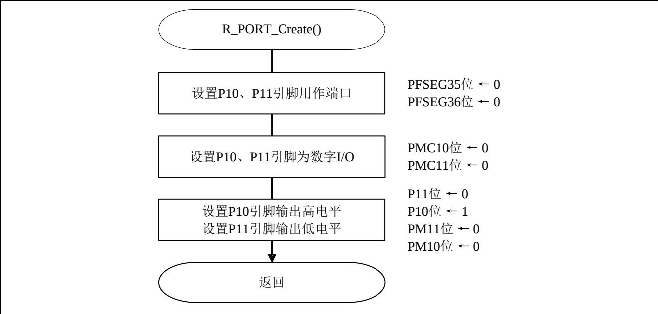
图 4.4 初始化端口
