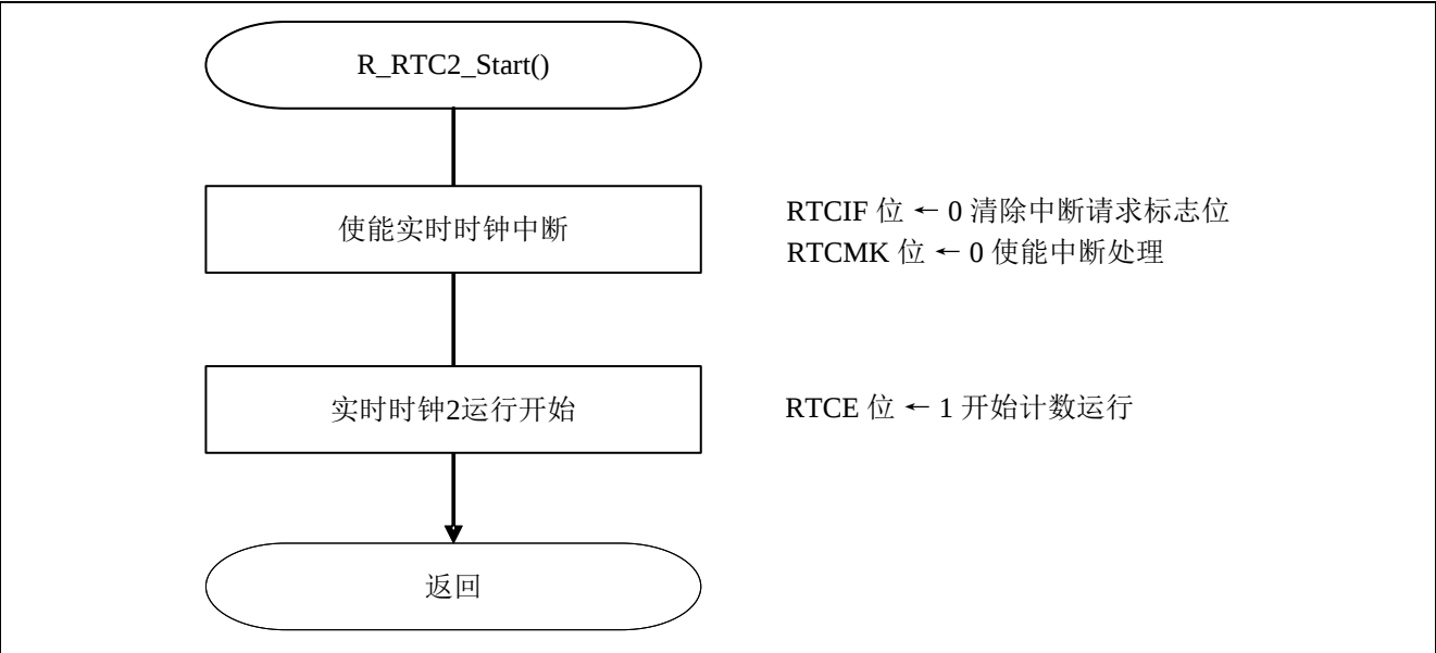
图 4.10 启动 RTC2
