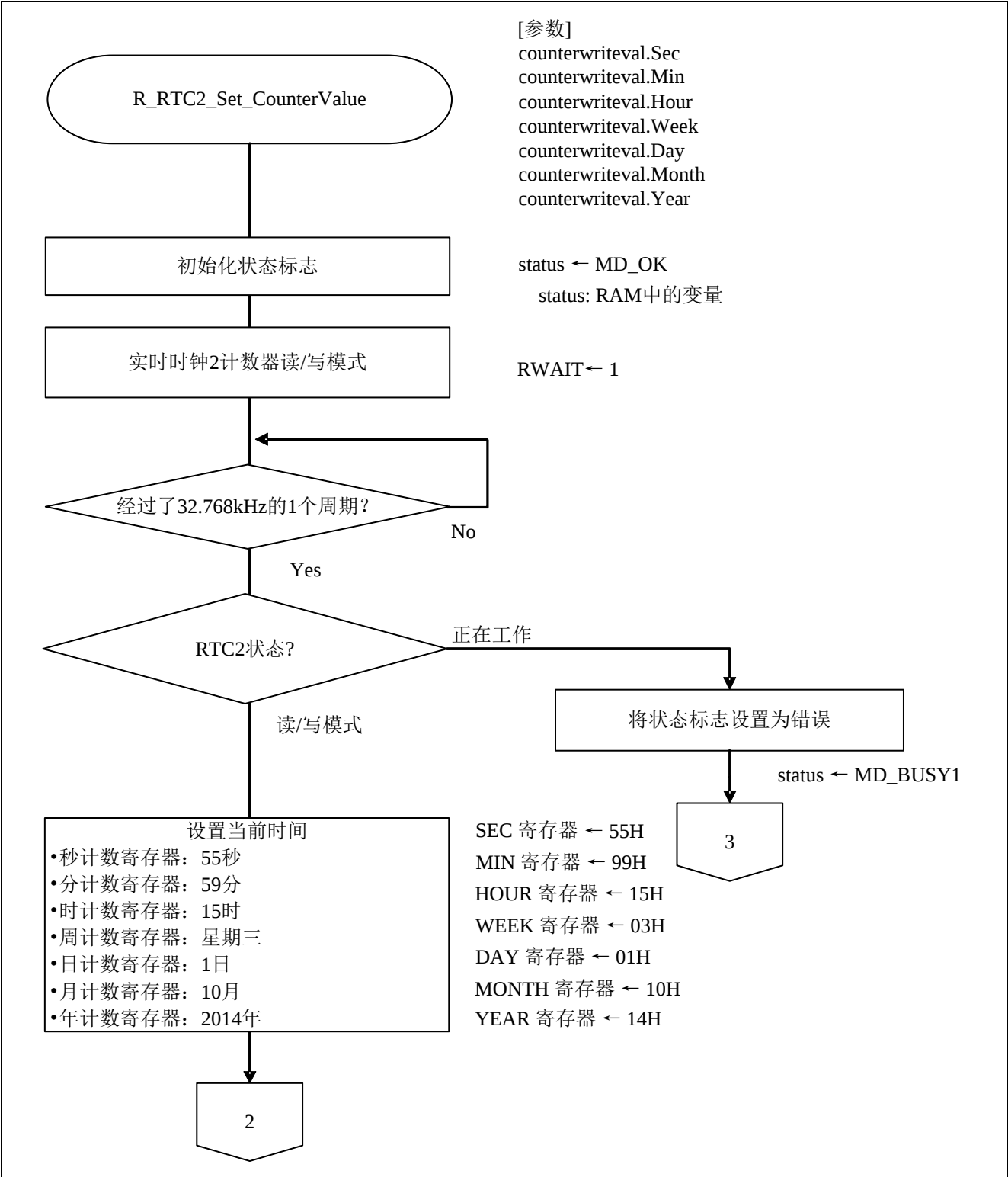
图 4.11 设置 RTC2 时间 (1/2)
