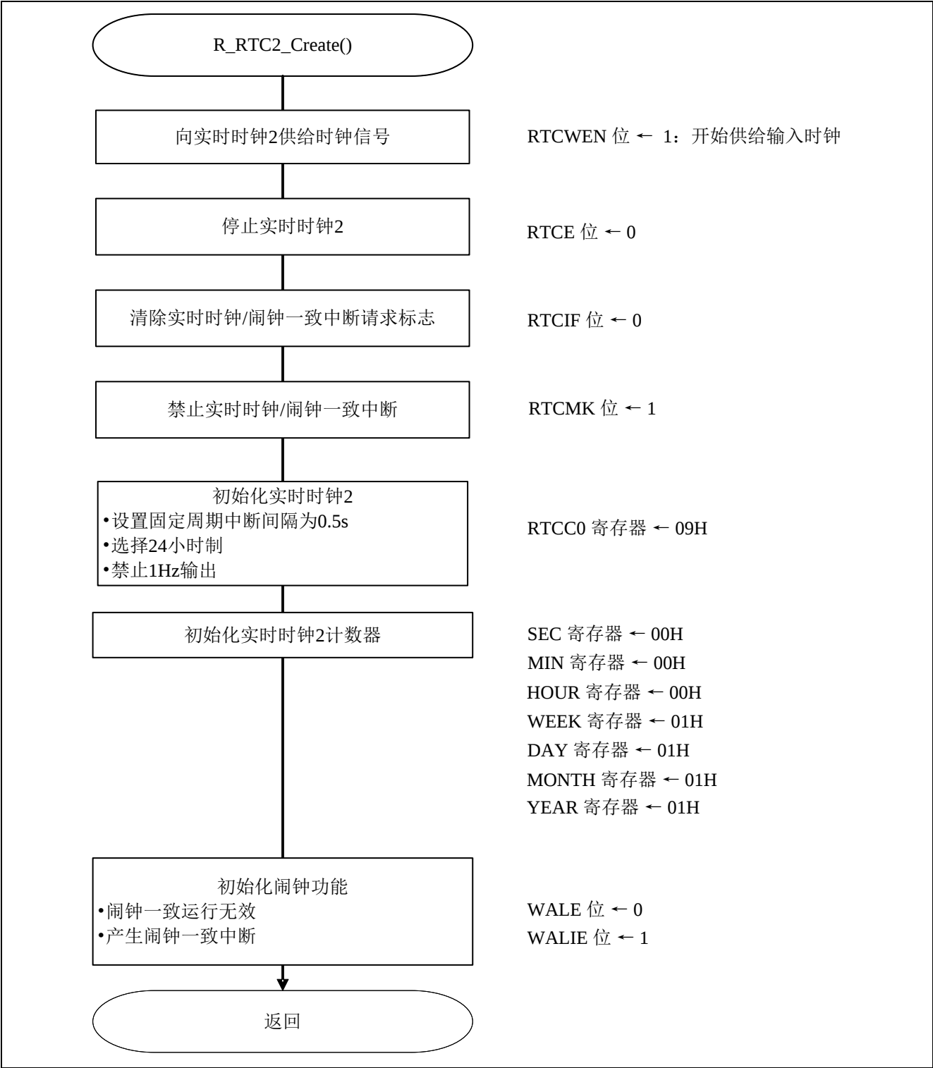
图 4.6 初始化 RTC2
