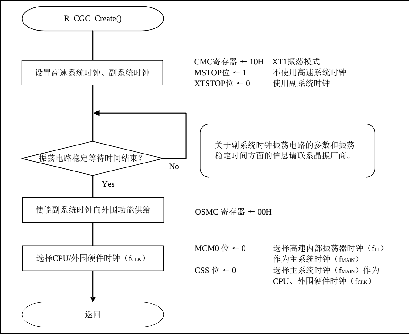
图 4.5 CPU 时钟设置
