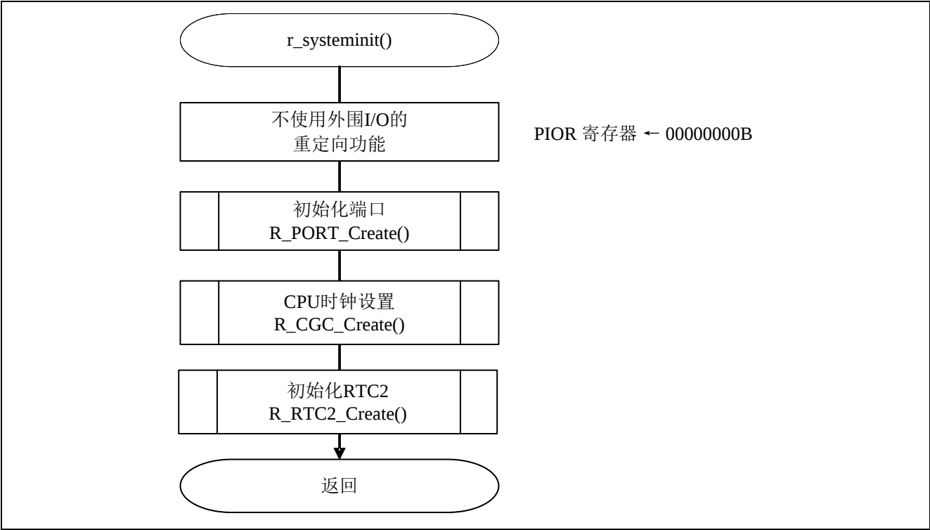
图 4.3 系统函数
