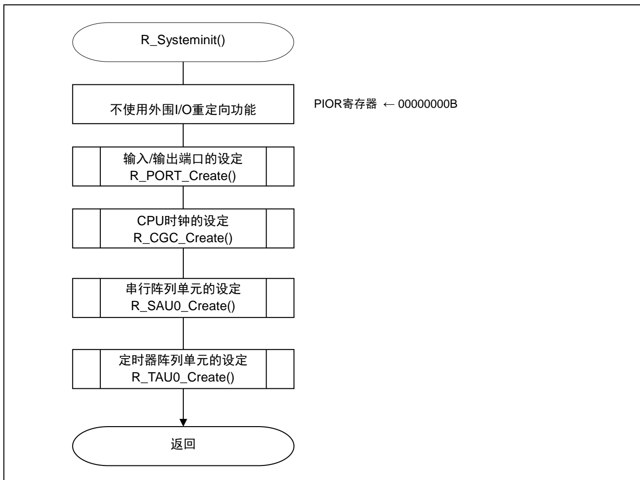
图 5.3 系统函数
