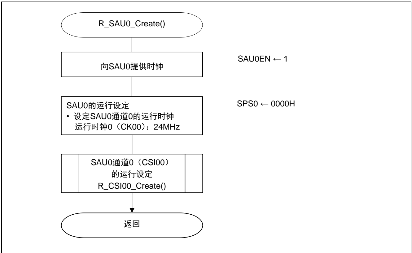
图 5.6 SAU0 的设置
