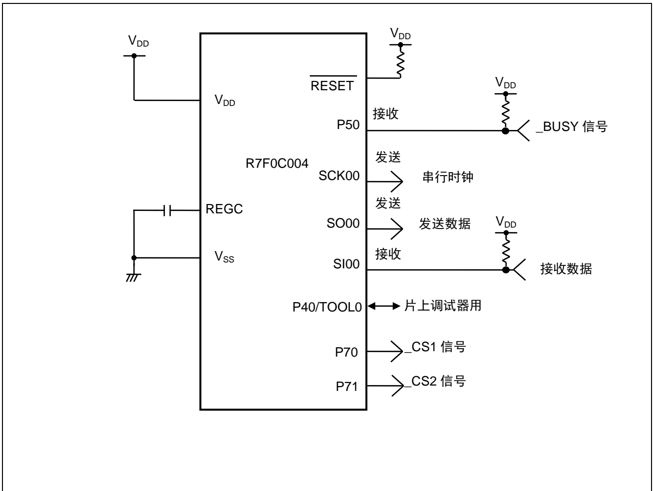
图 4.1 硬件配置
