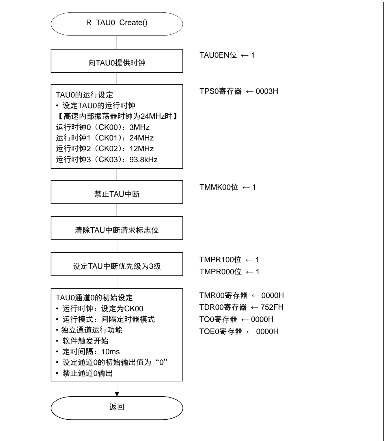
图 5.8 TAU0 的设定
