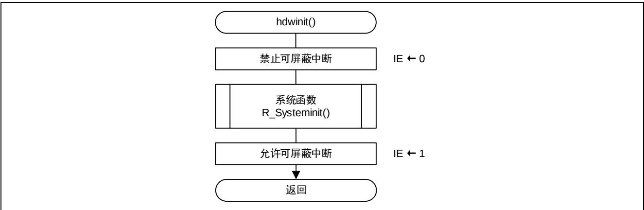
图 4.4 初始化函数
