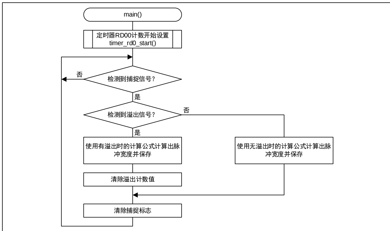
图 4.8 主函数处理
