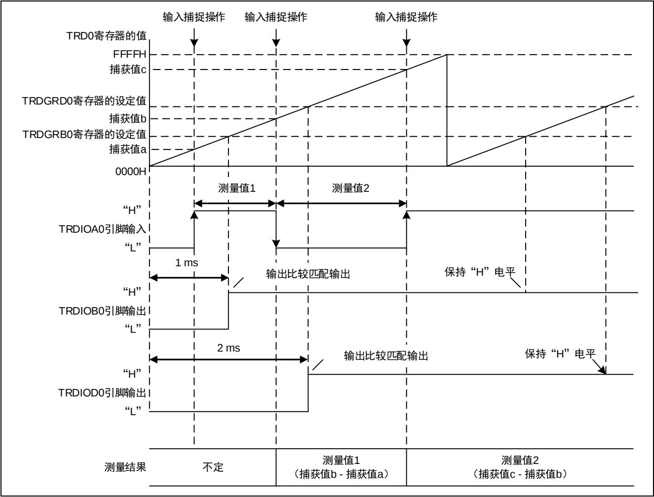
图 1.1 输出时序图
