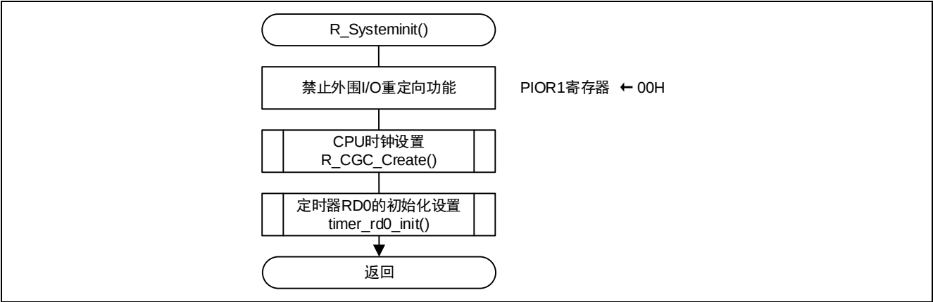
图 4.5 系统函数
