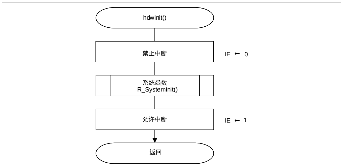
图 4.2 初始化函数
