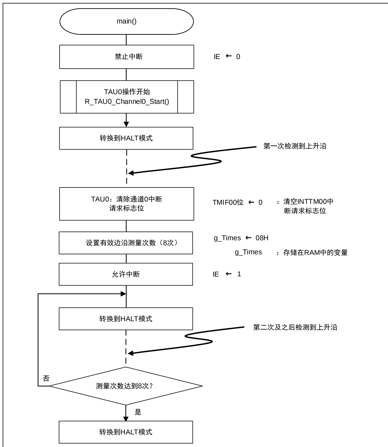
图 4.7 主函数处理
