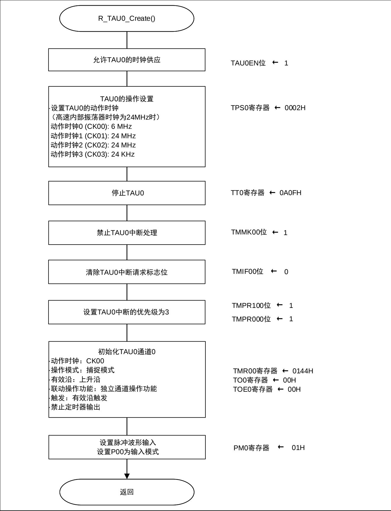
图 4.6 TAU0 初始化
