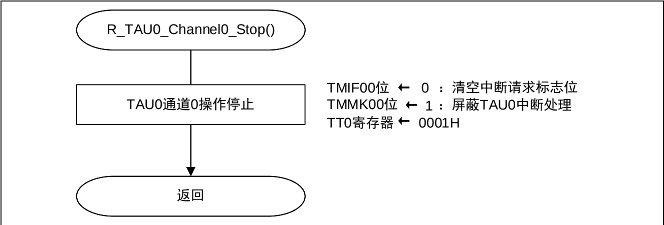
图 4.9 TAU0 操作停止
