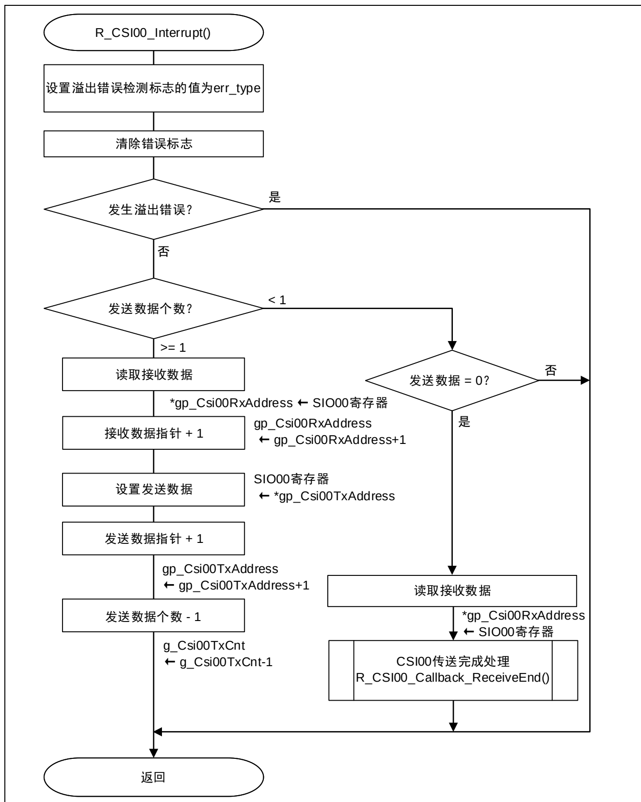
图 5.12 CSI00 传送结束中断处理
