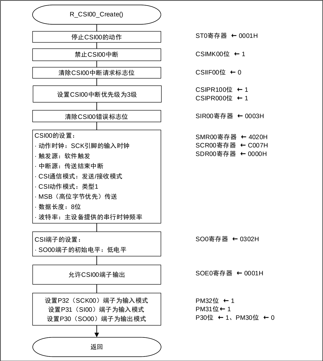
图 5.7 SAU0 通道 0（CSI00）的动作设置
