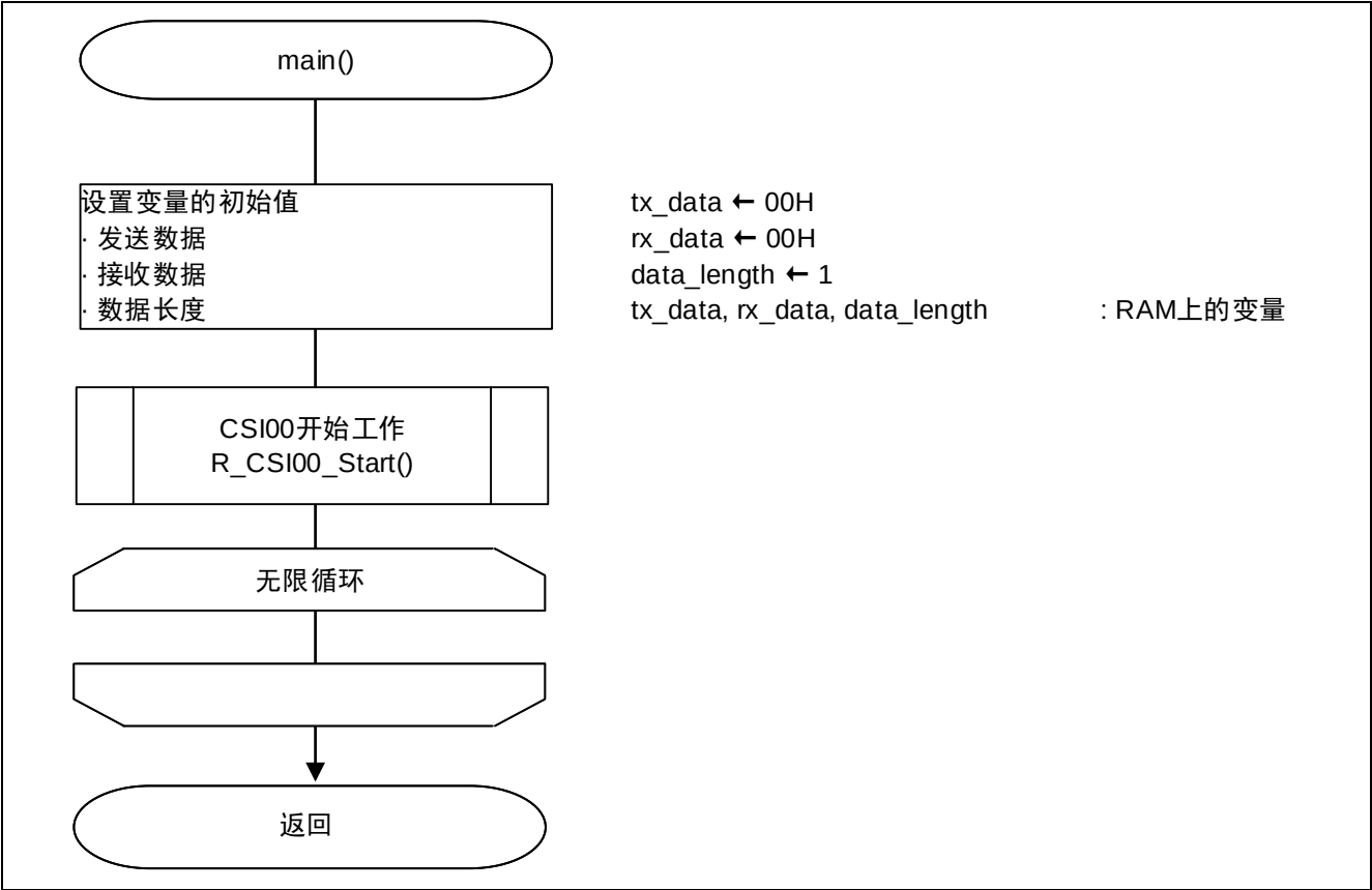
图 5.8 主函数处理
