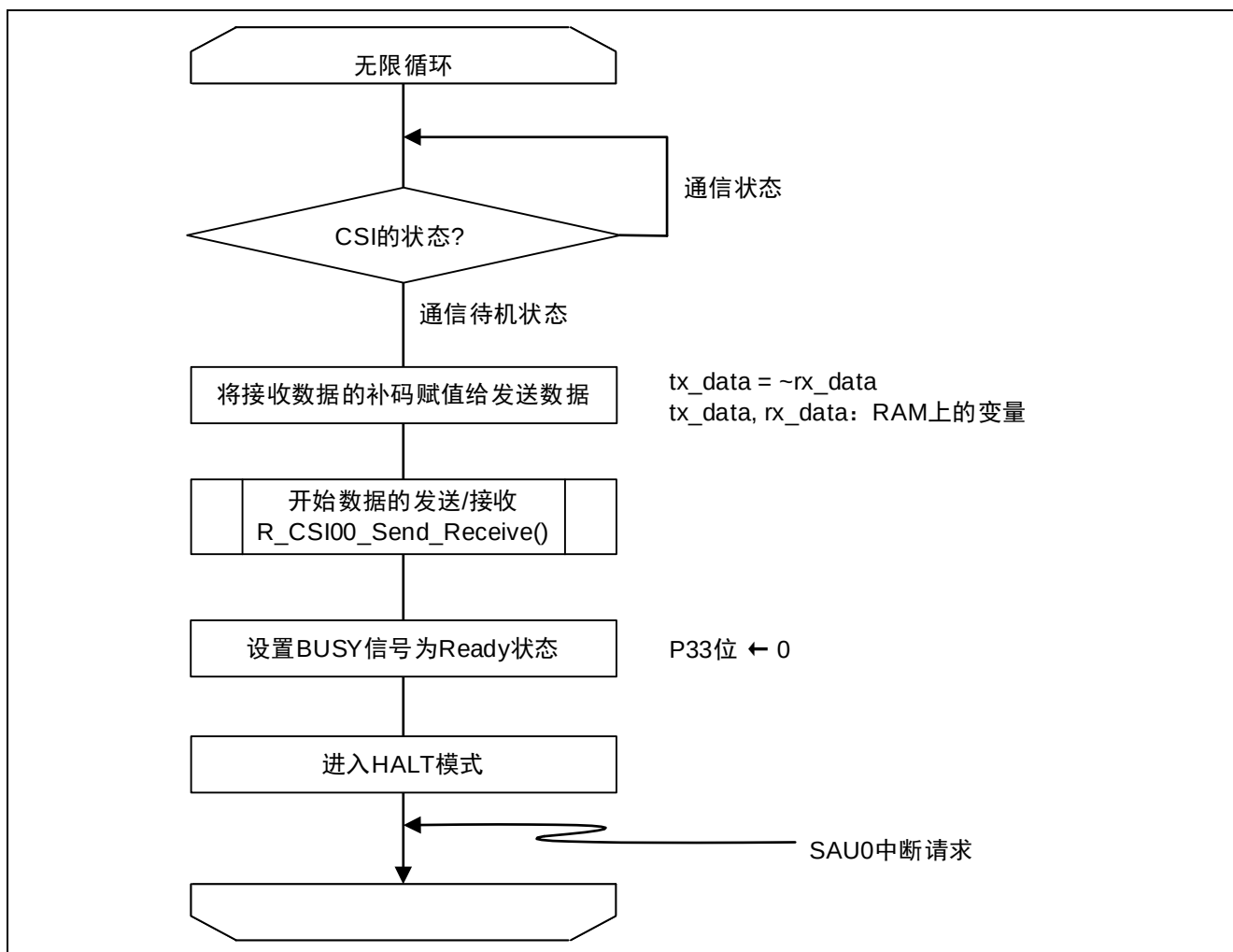
图 5.10 主函数处理中的无限循环
