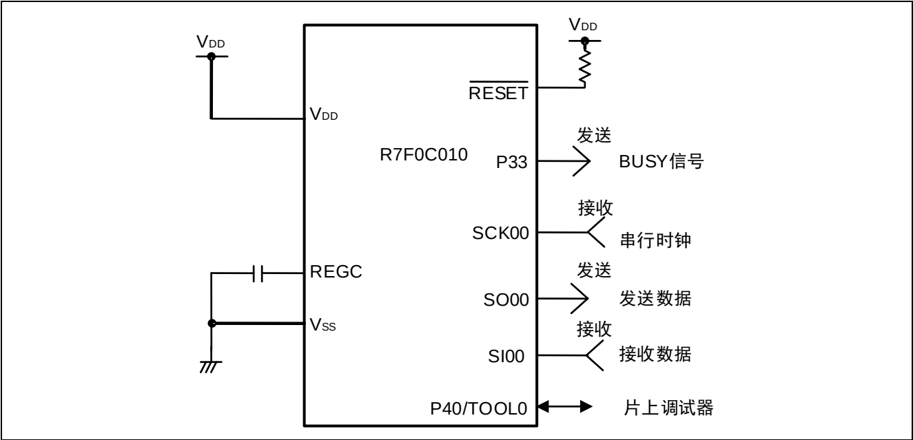
图 4.1 硬件配置
