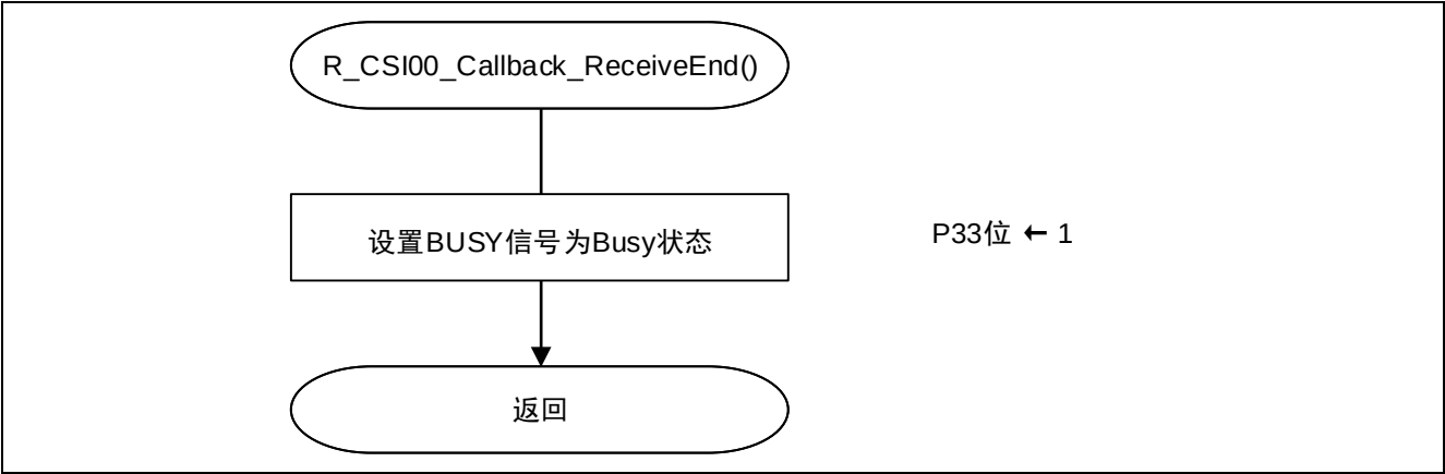
图 5.13 CSI00 传送完成处理
