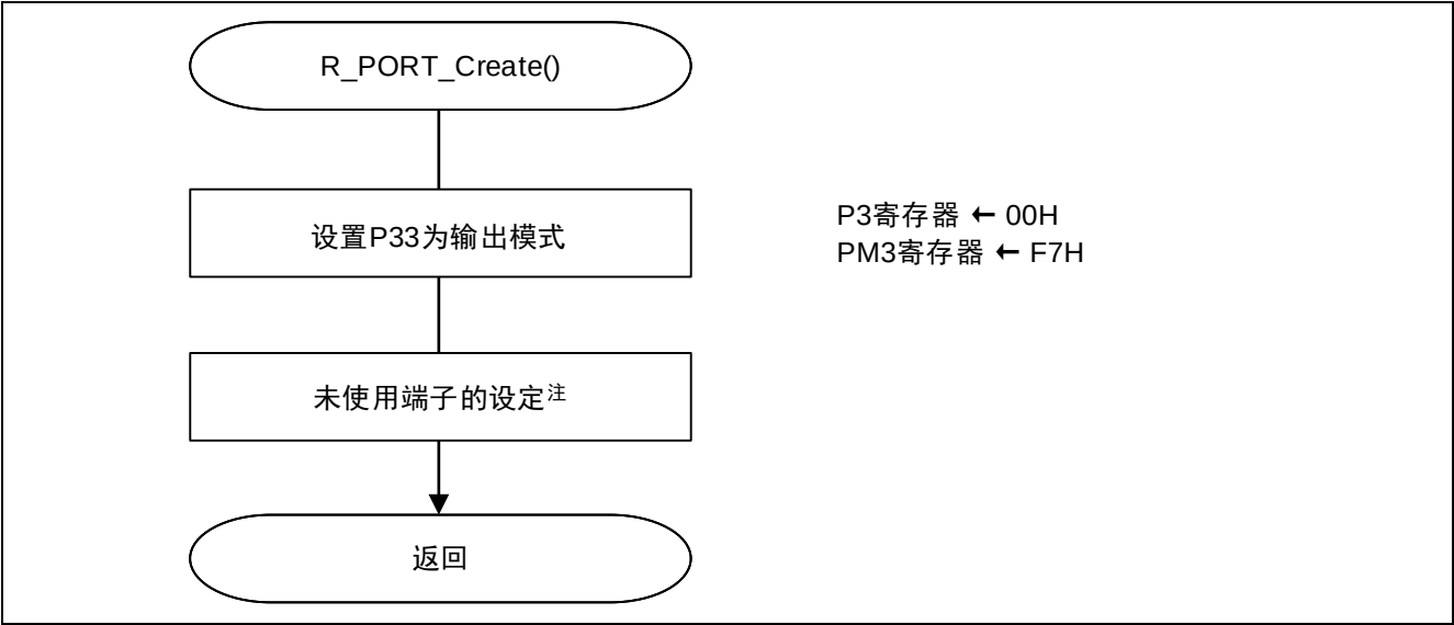
图 5.4 初始化端口
