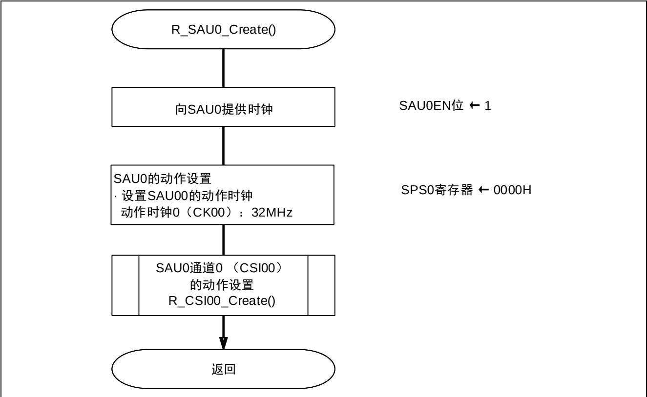
图 5.6 串行阵列单元设置
