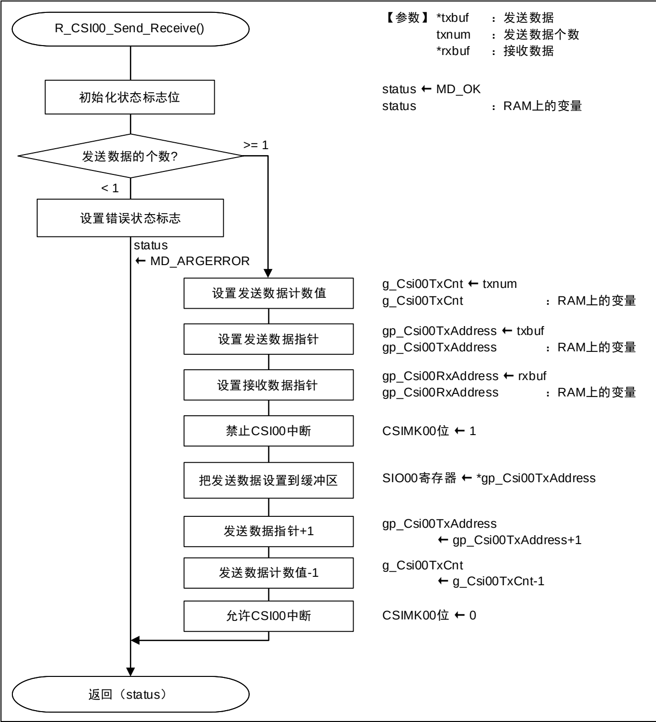
图 5.11 CSI00 开始数据发送/接收的处理
