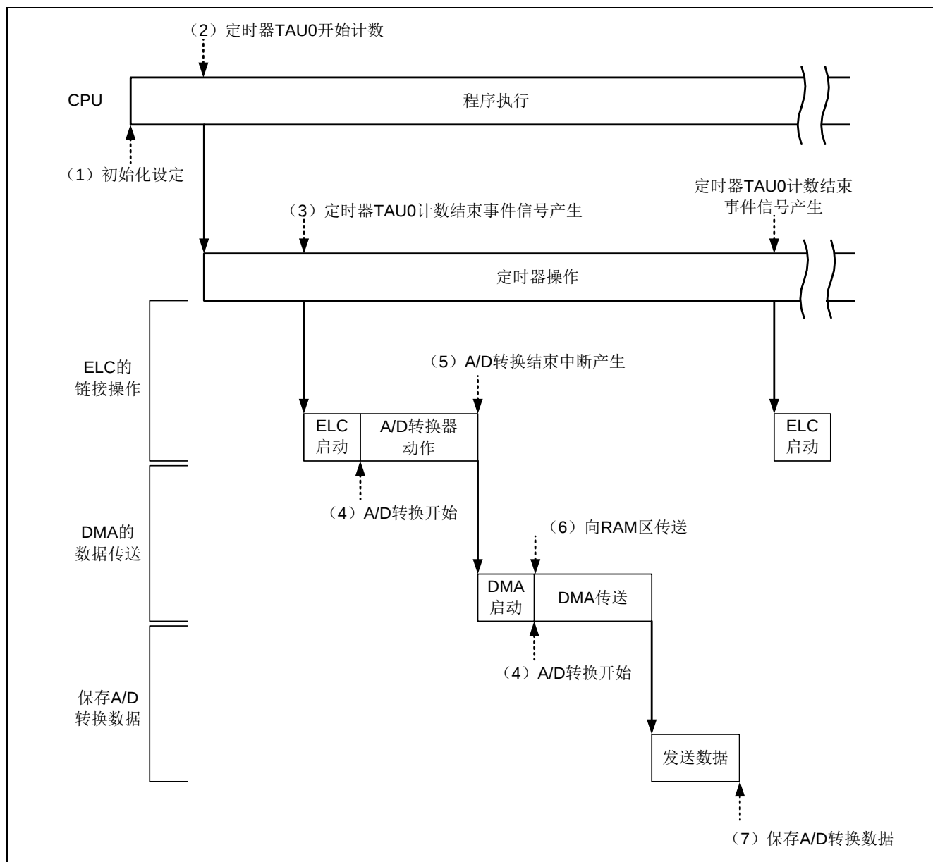
图 4.3 使用 ELC 和 DMA 进行数据保存
