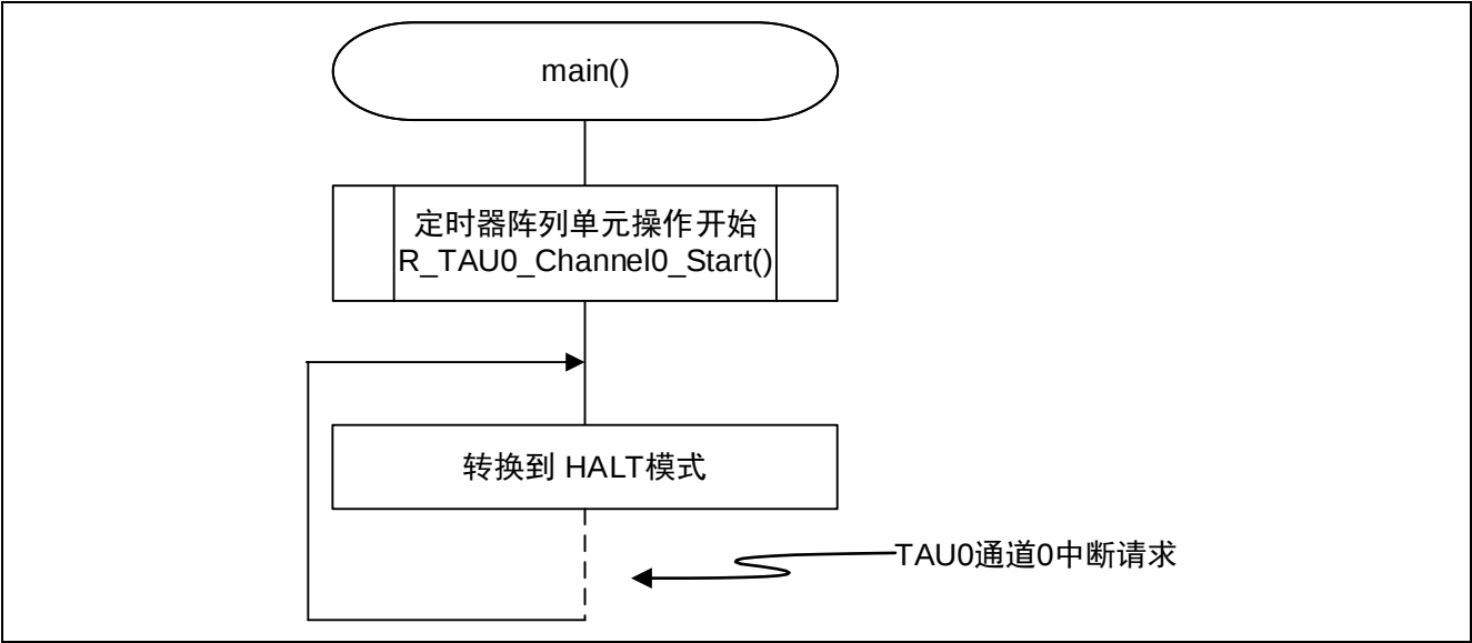
图 4.8 主函数处理
