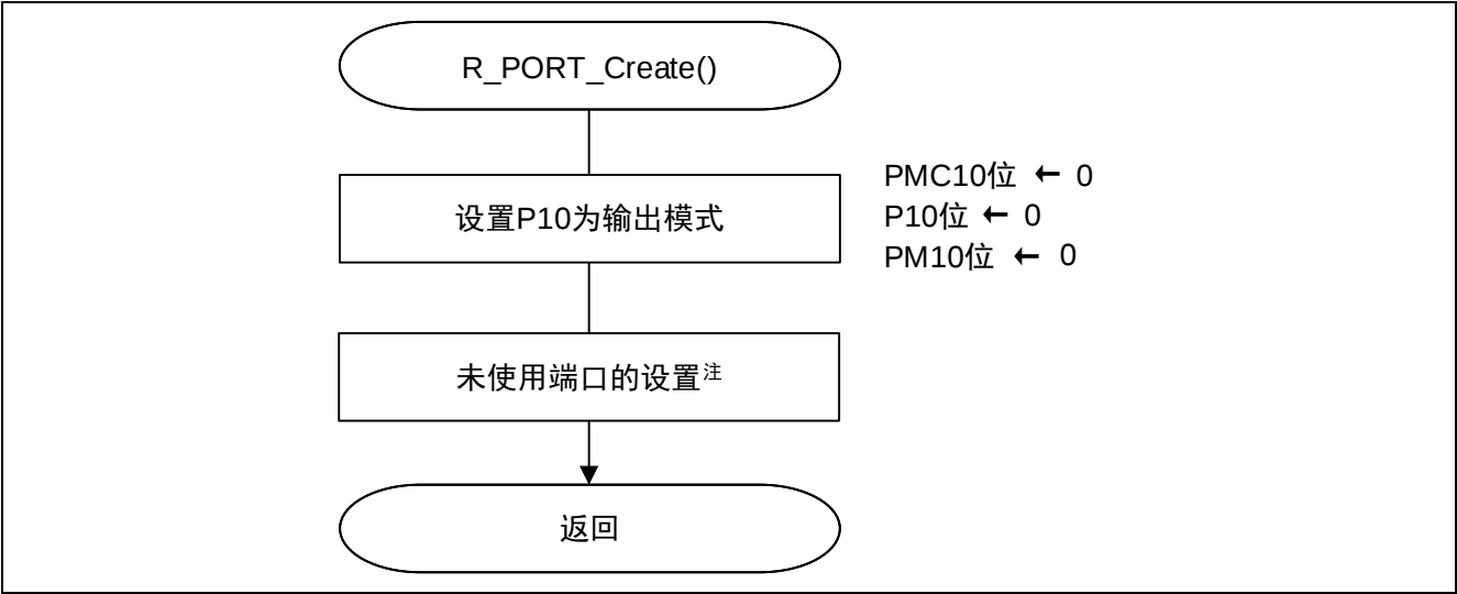
图 4.4 初始化端口
