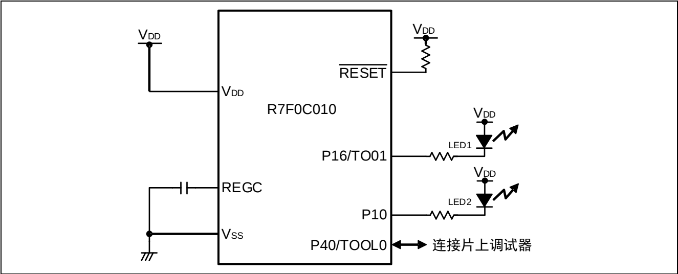
图 3.1 硬件配置
