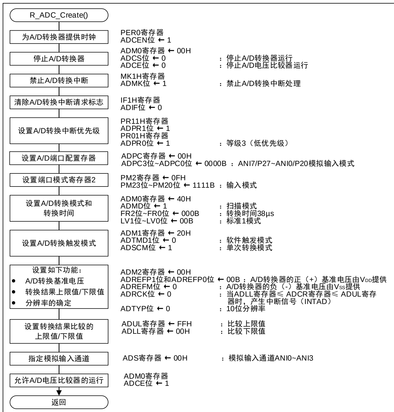
图 4.6 A/D 转换器初始化设置
