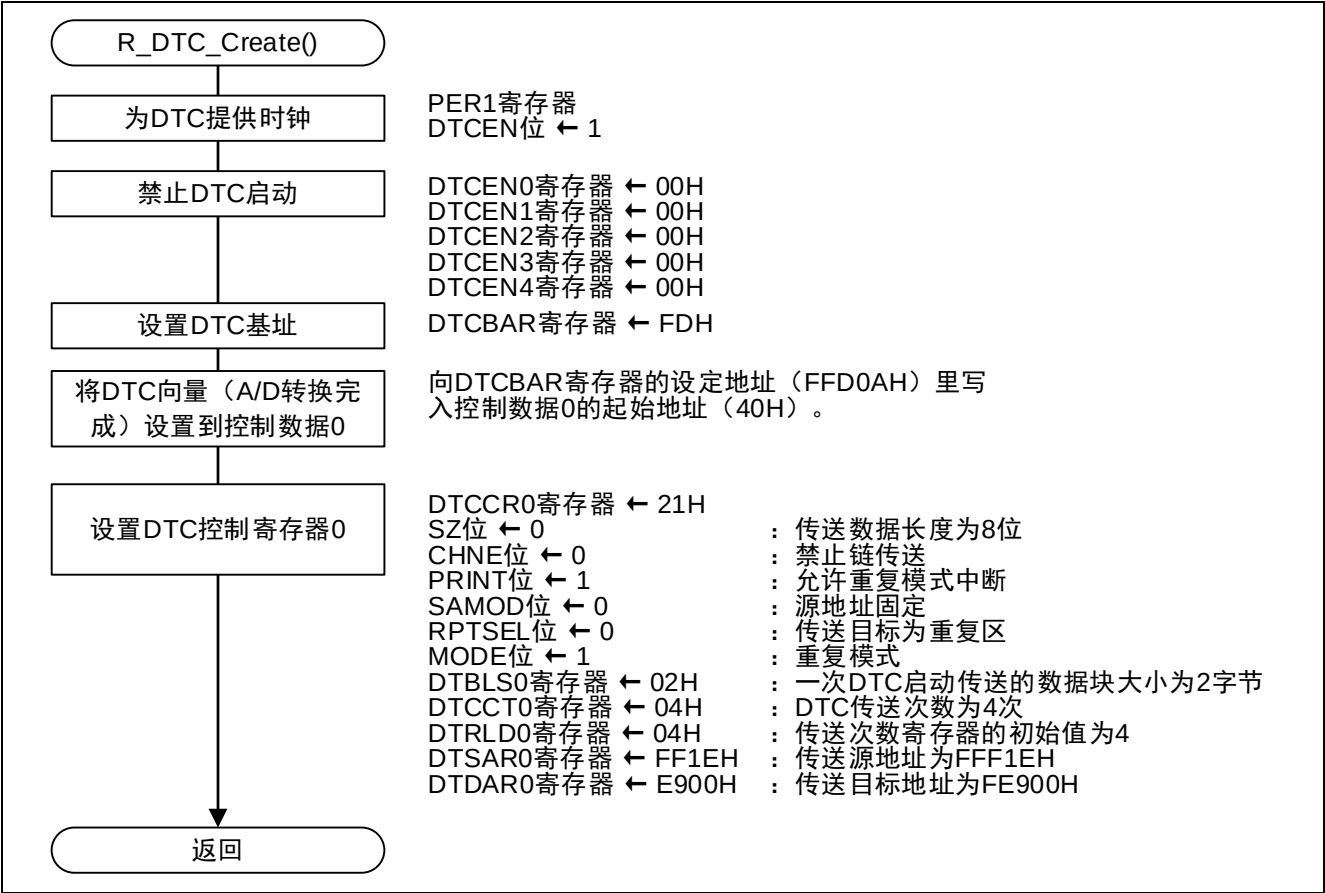
图 4.7 DTC 初始化设置
