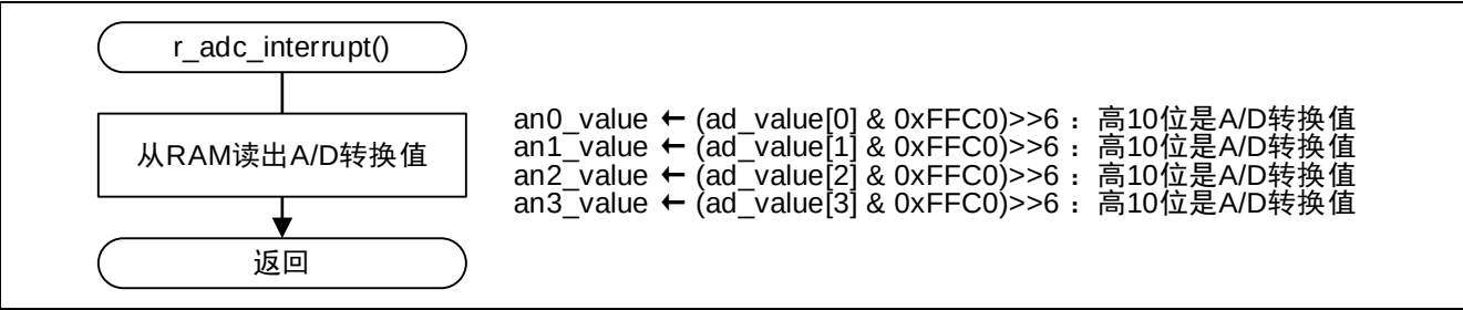
图 4.11 A/D 转换结束中断处理
