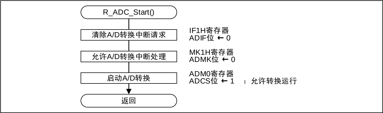
图 4.10 A/D 转换动作开始
