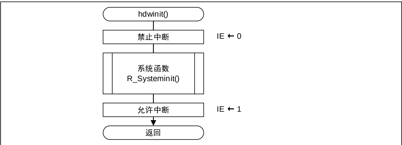
图 4.3 初始化函数
