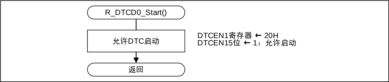
图 4.9 DTCD0 动作开始
