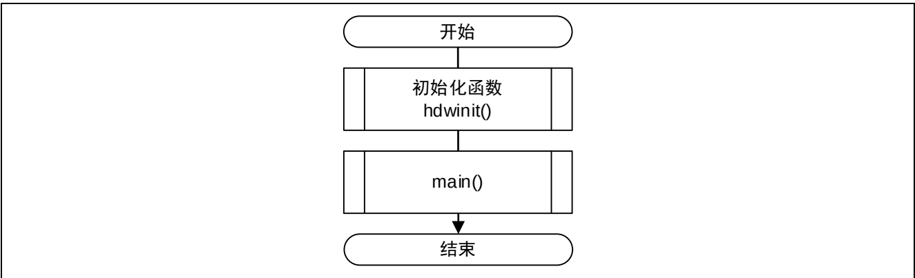
图 4.2 整体流程图
