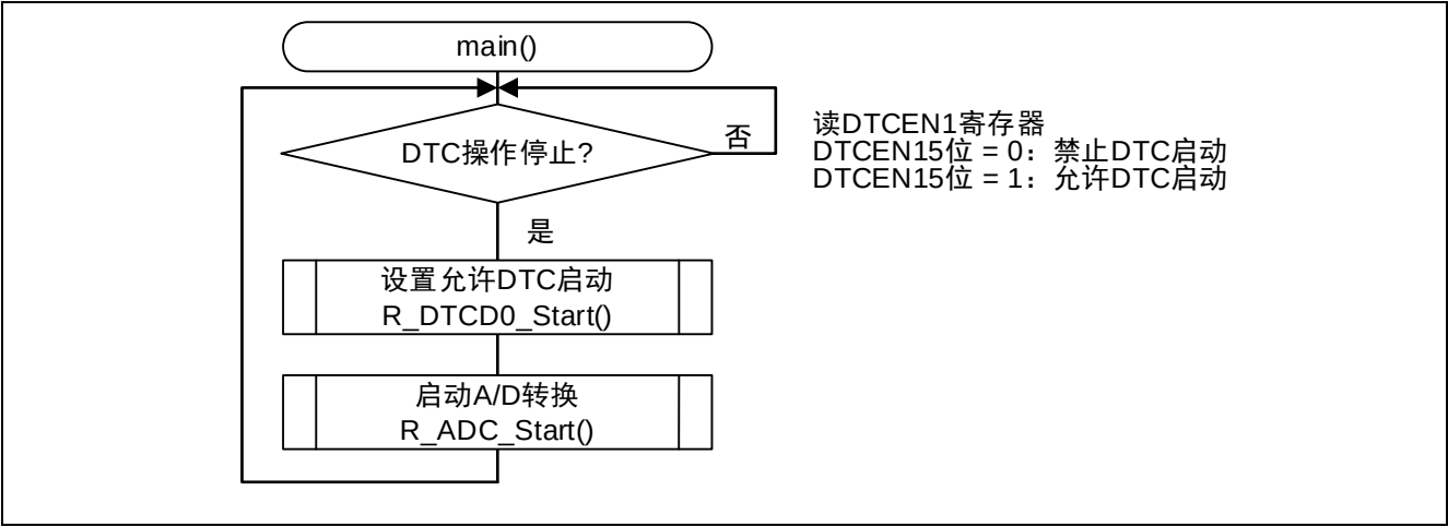
图 4.8 主函数处理
