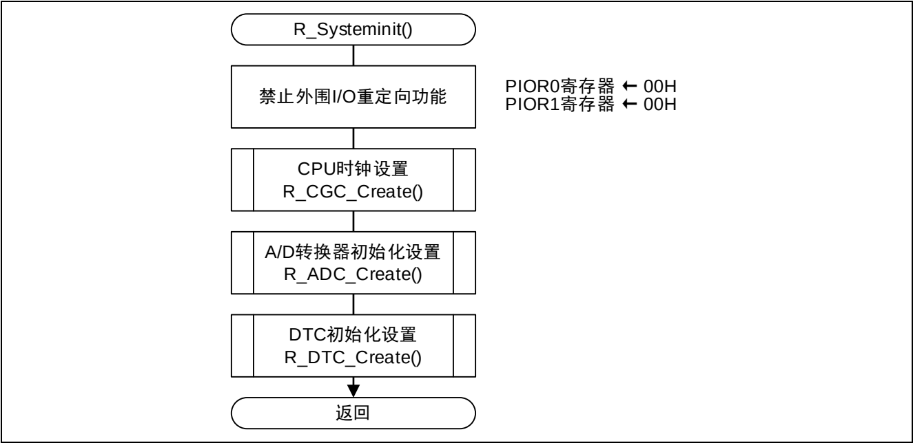
图 4.4 系统函数
