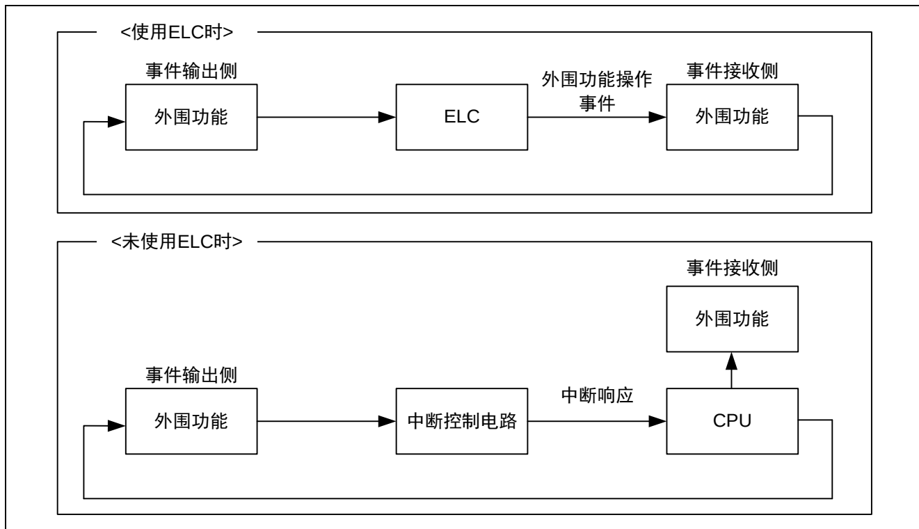
图 1.1 使用 ELC 和未使用 ELC 时的比较图
