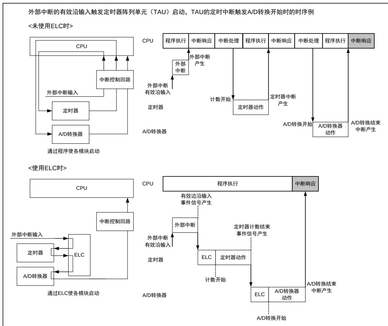
图 2.1 使用 ELC 时和未使用 ELC 时的处理比较图
