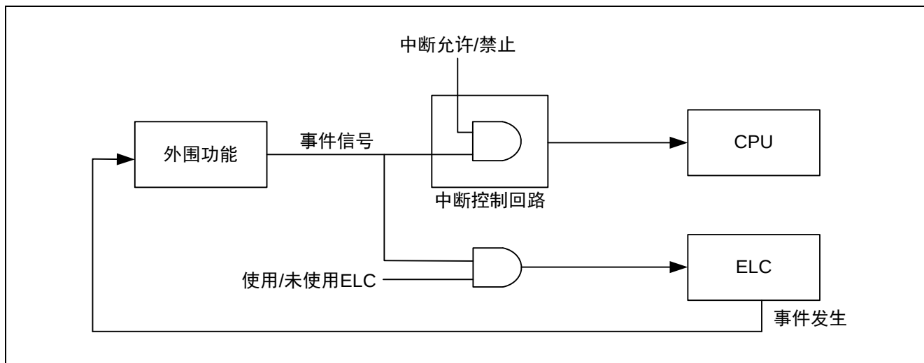
图 1.2 中断处理与 ELC 的关系
