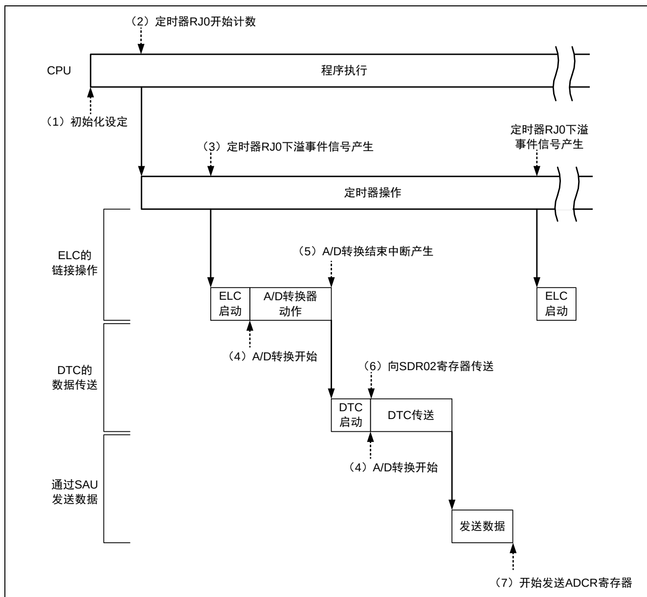
图 4.3 使用 ELC 和 DTC 进行数据发送
