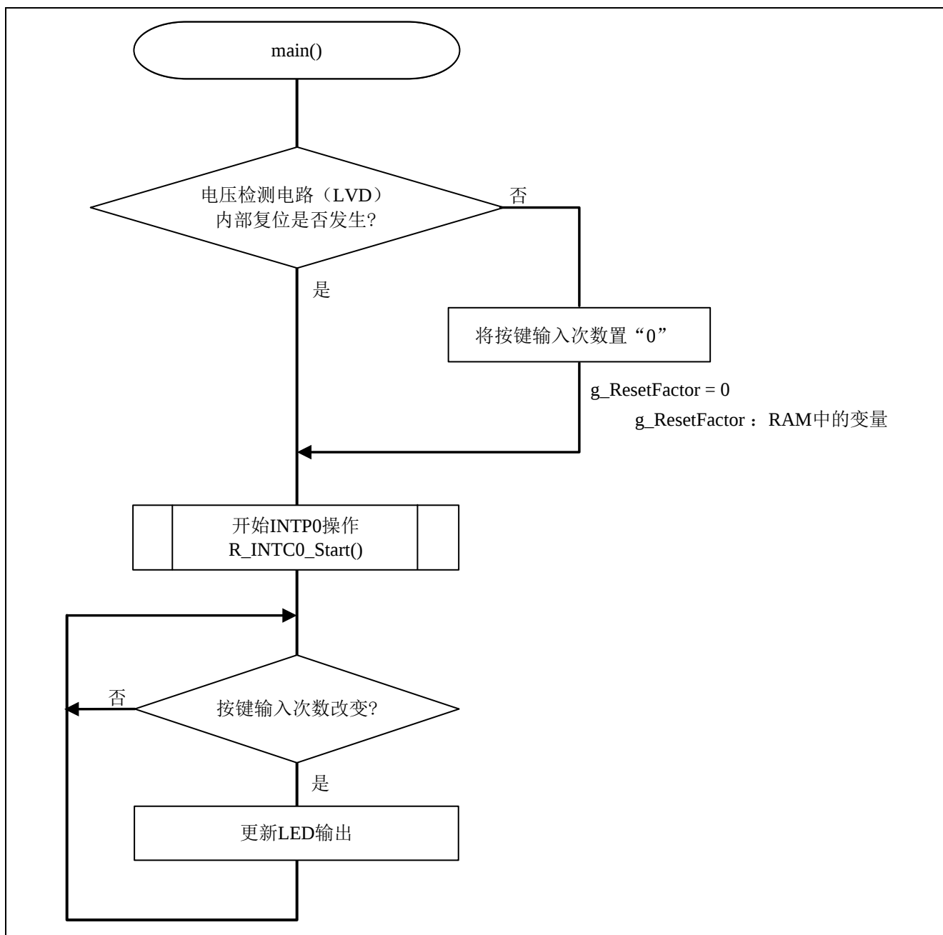
图 4.8 主函数处理
