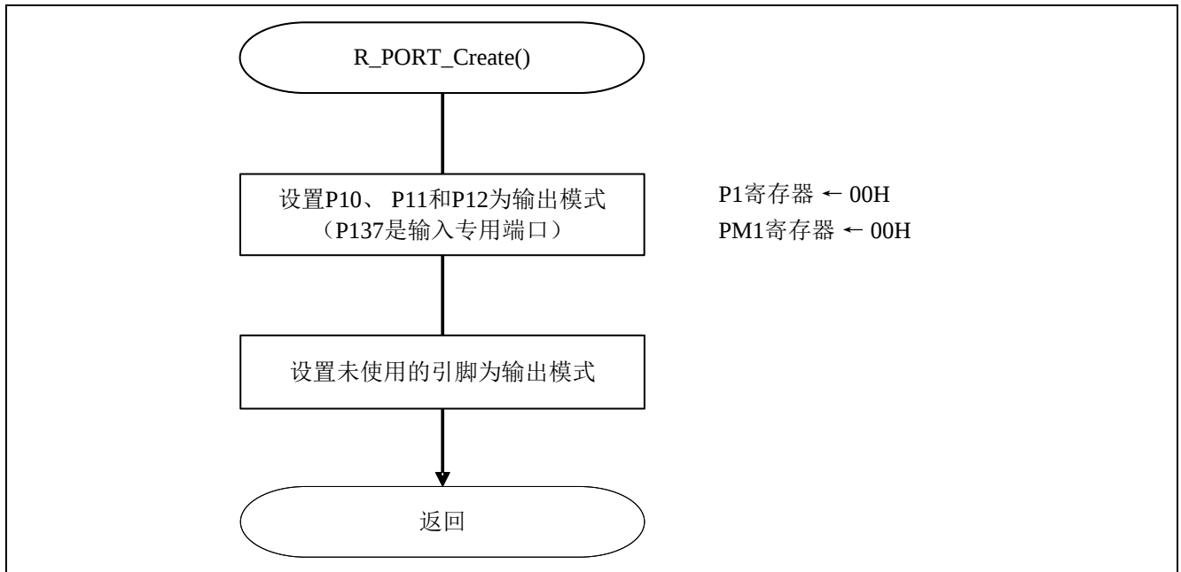
图 4.5 初始化端口
