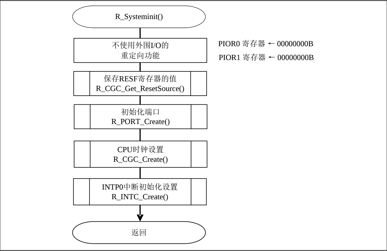
图 4.4 系统函数
