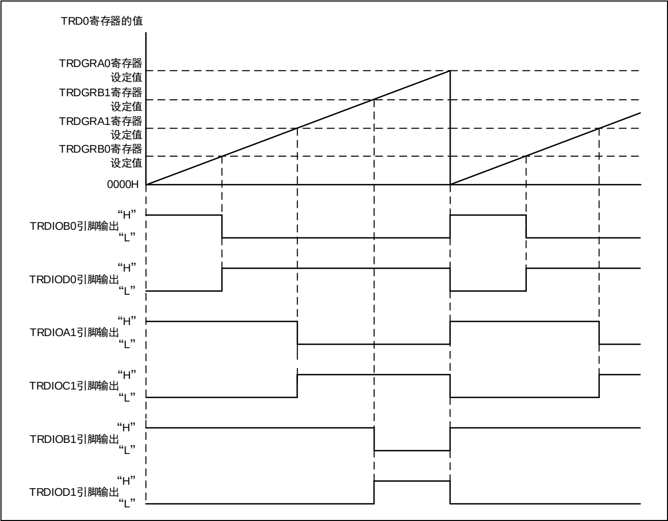
图 1.1 复位同步 PWM 的输出波形
