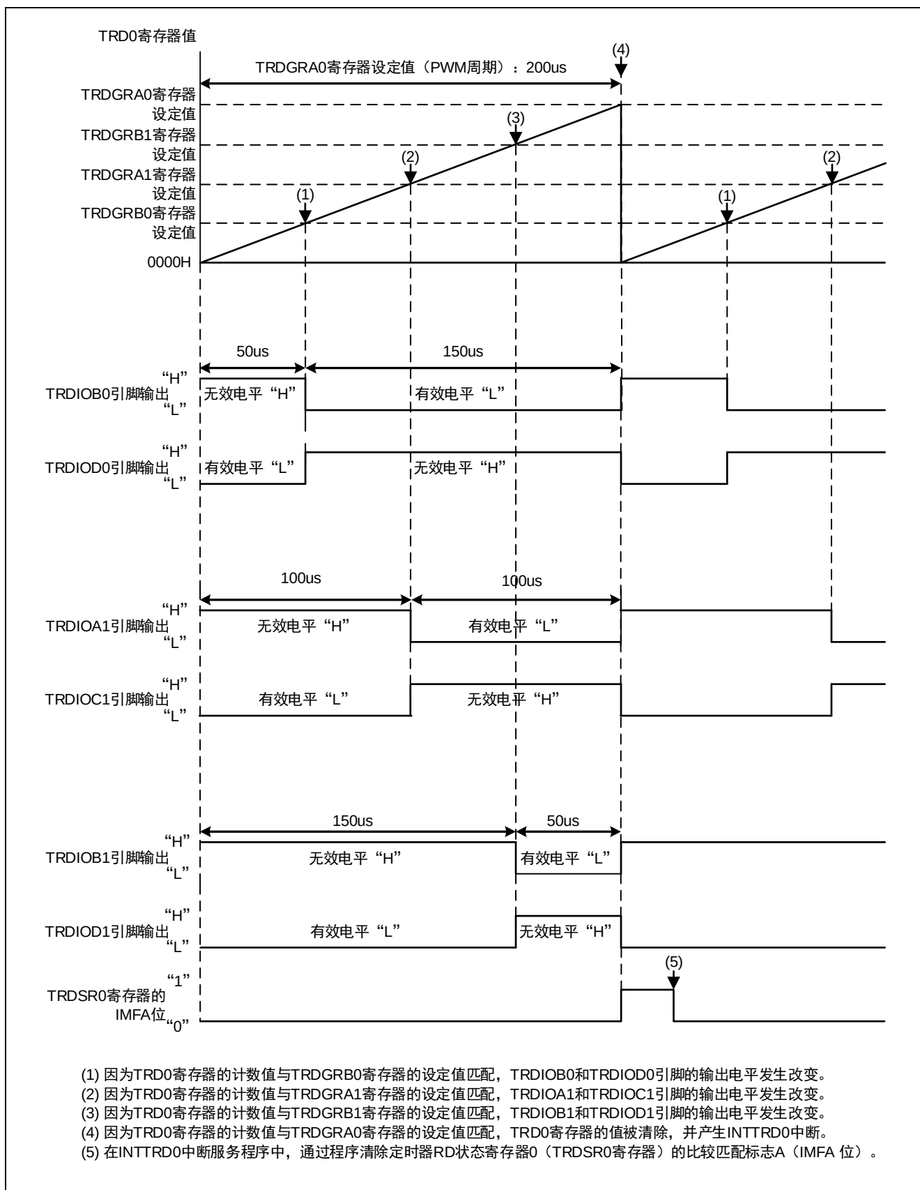
图 4.1 PWM 输出波形
