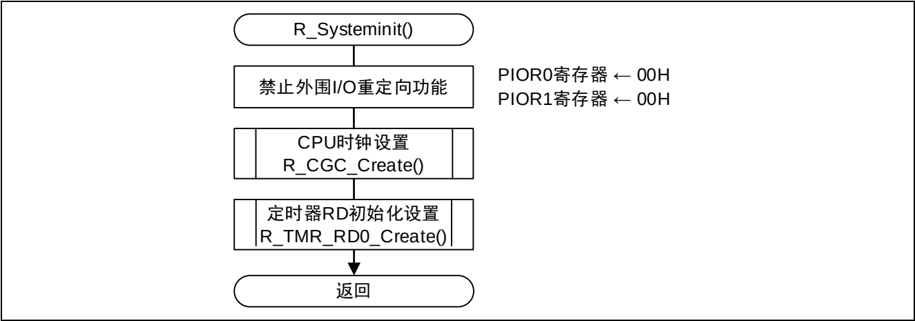
图 4.4 系统函数
