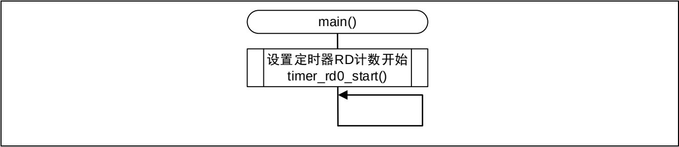
图 4.8 主函数处理
