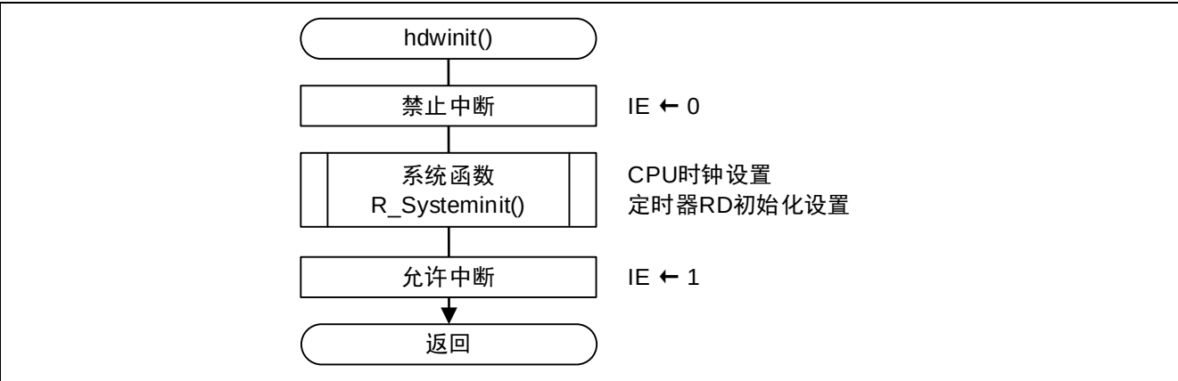
图 4.3 初始化函数
