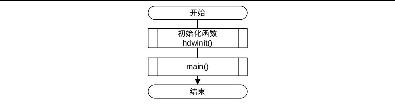
图 4.2 整体流程图
