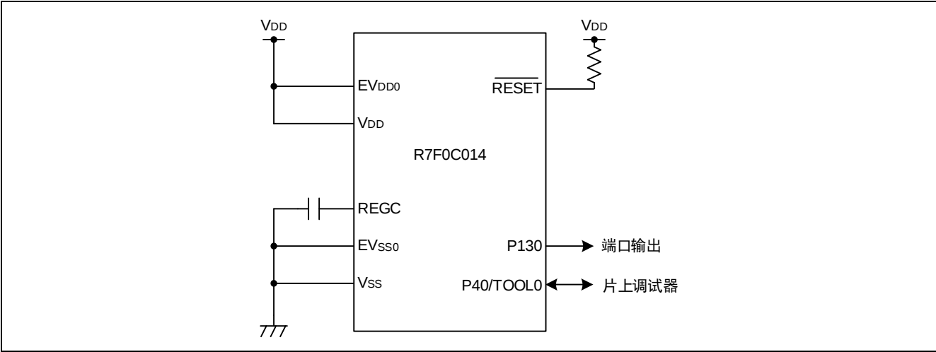
图 4.1 硬件配置
