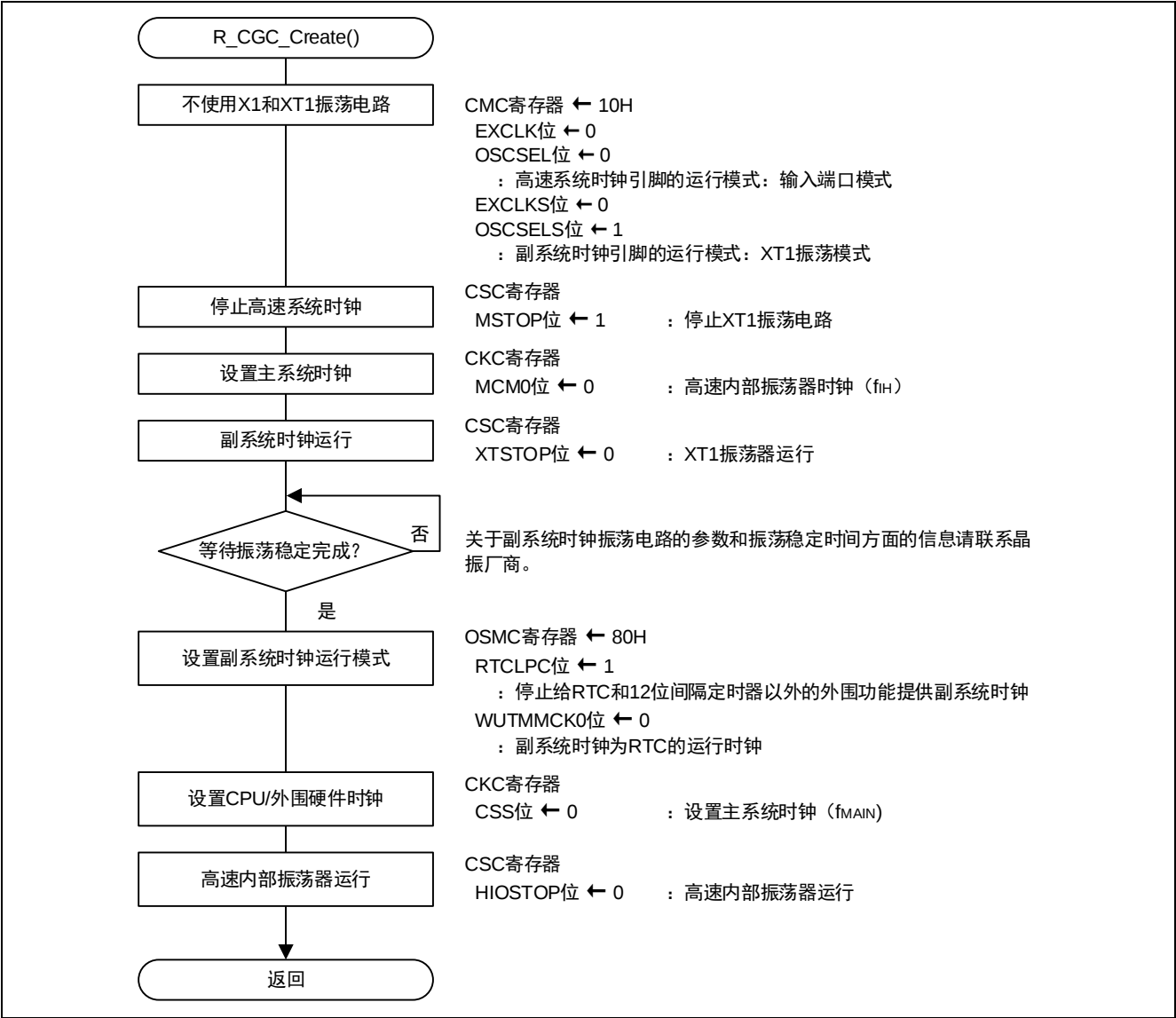
图 5.5 CPU 时钟设置
