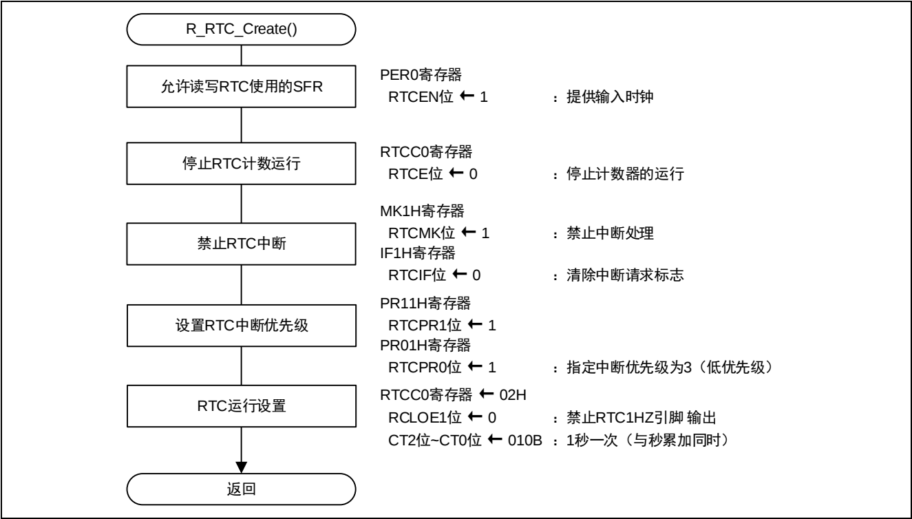
图 5.7 RTC 初始化设置
