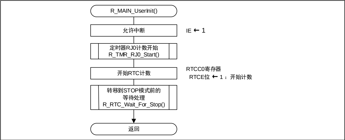
图 5.11 主函数初始化
