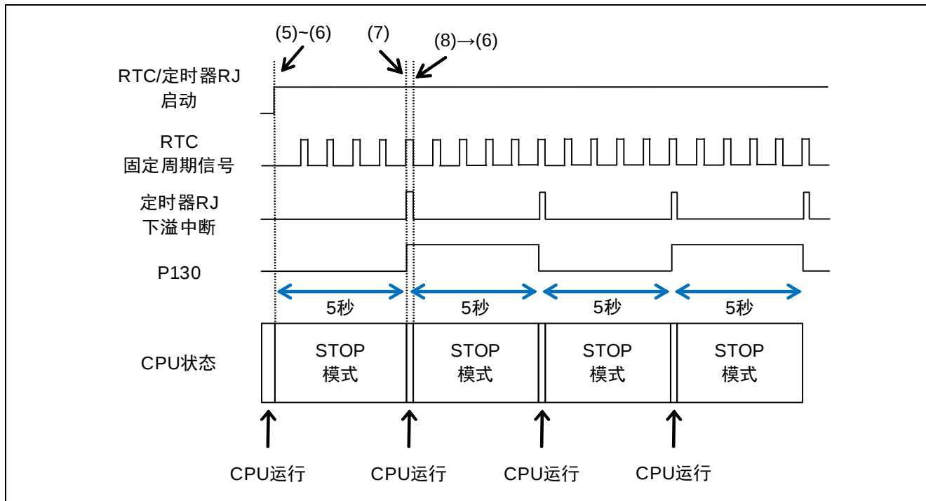
图 5.1 时序图
