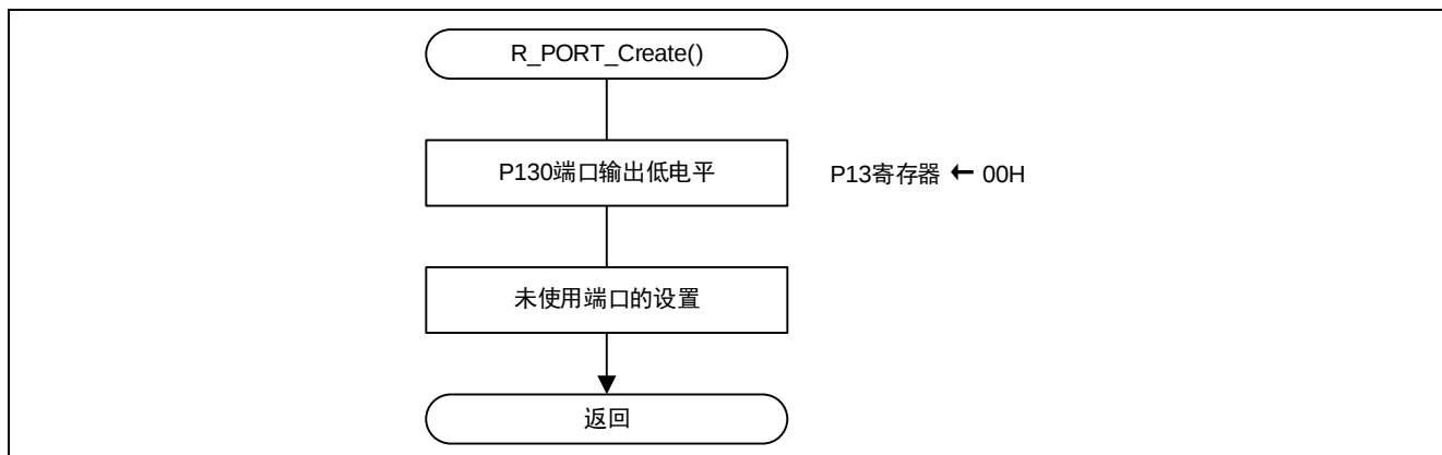
图 5.6 初始化端口
