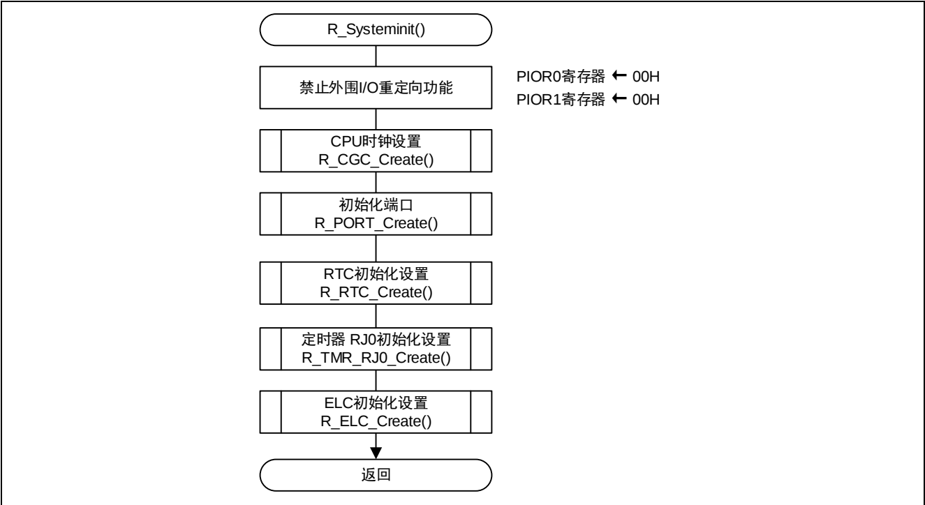
图 5.4 系统函数
