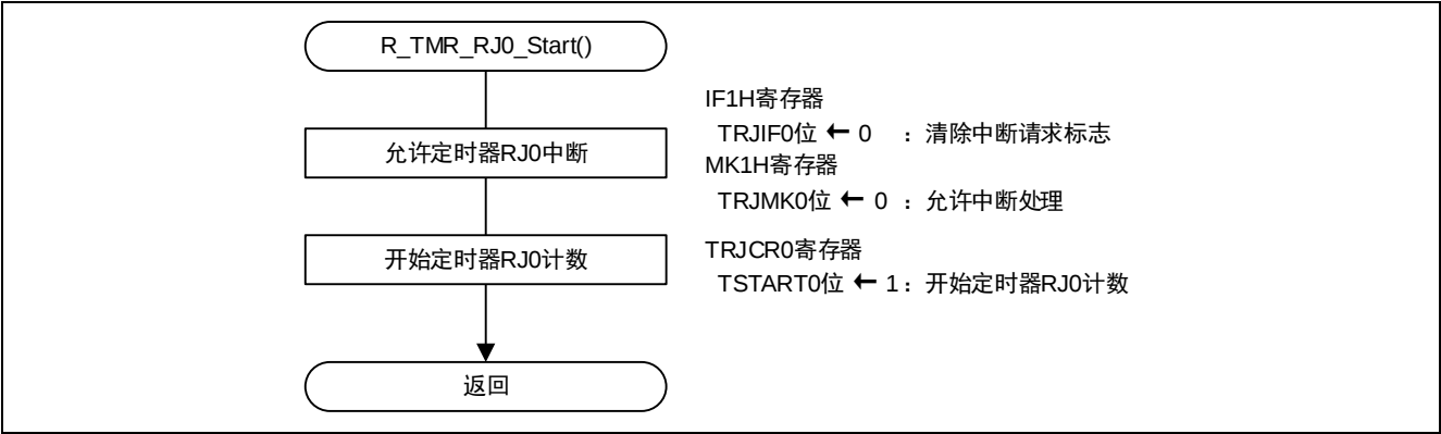
图 5.12 定时器 RJ0 计数开始
