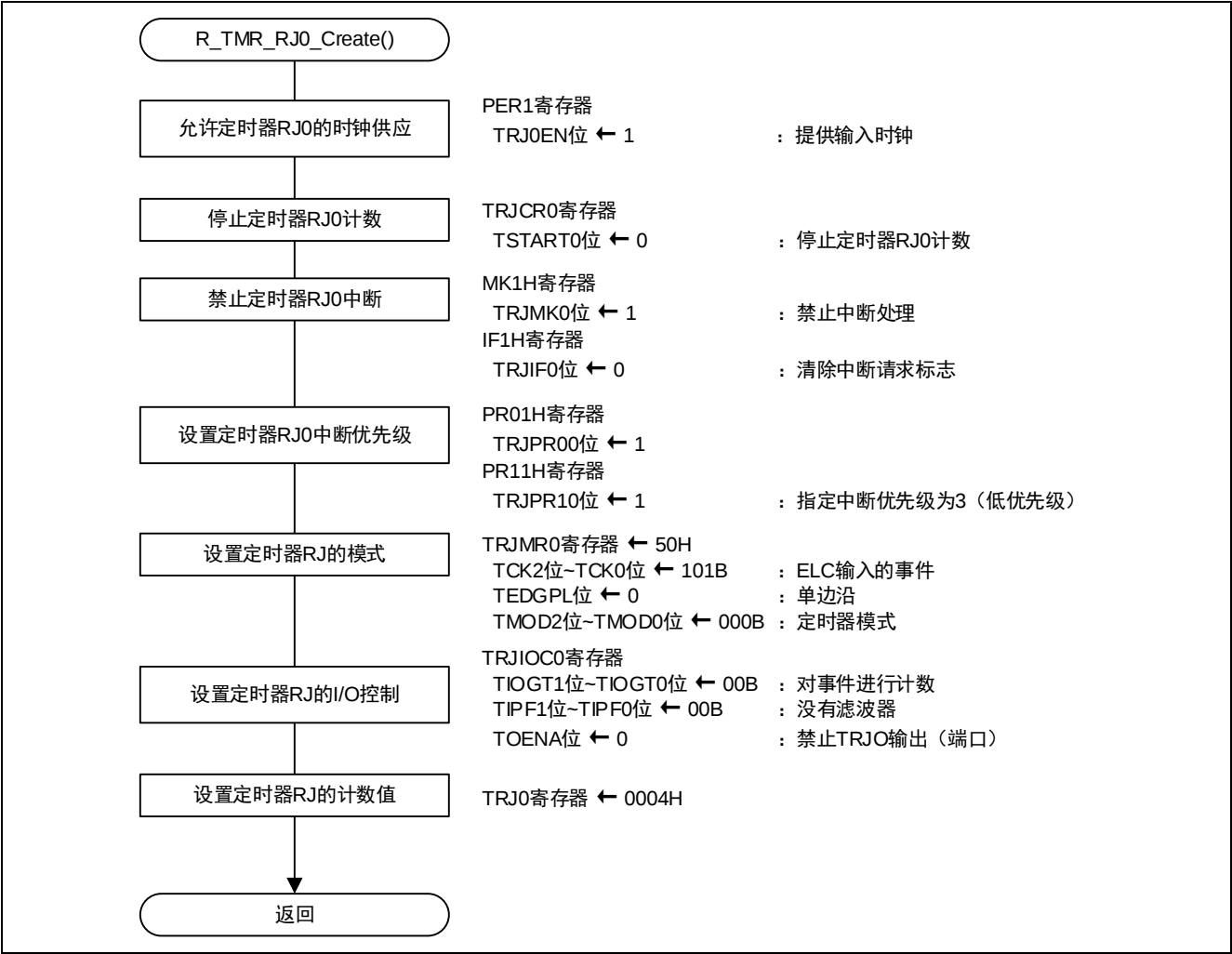
图 5.8 定时器 RJ0 初始化设置
