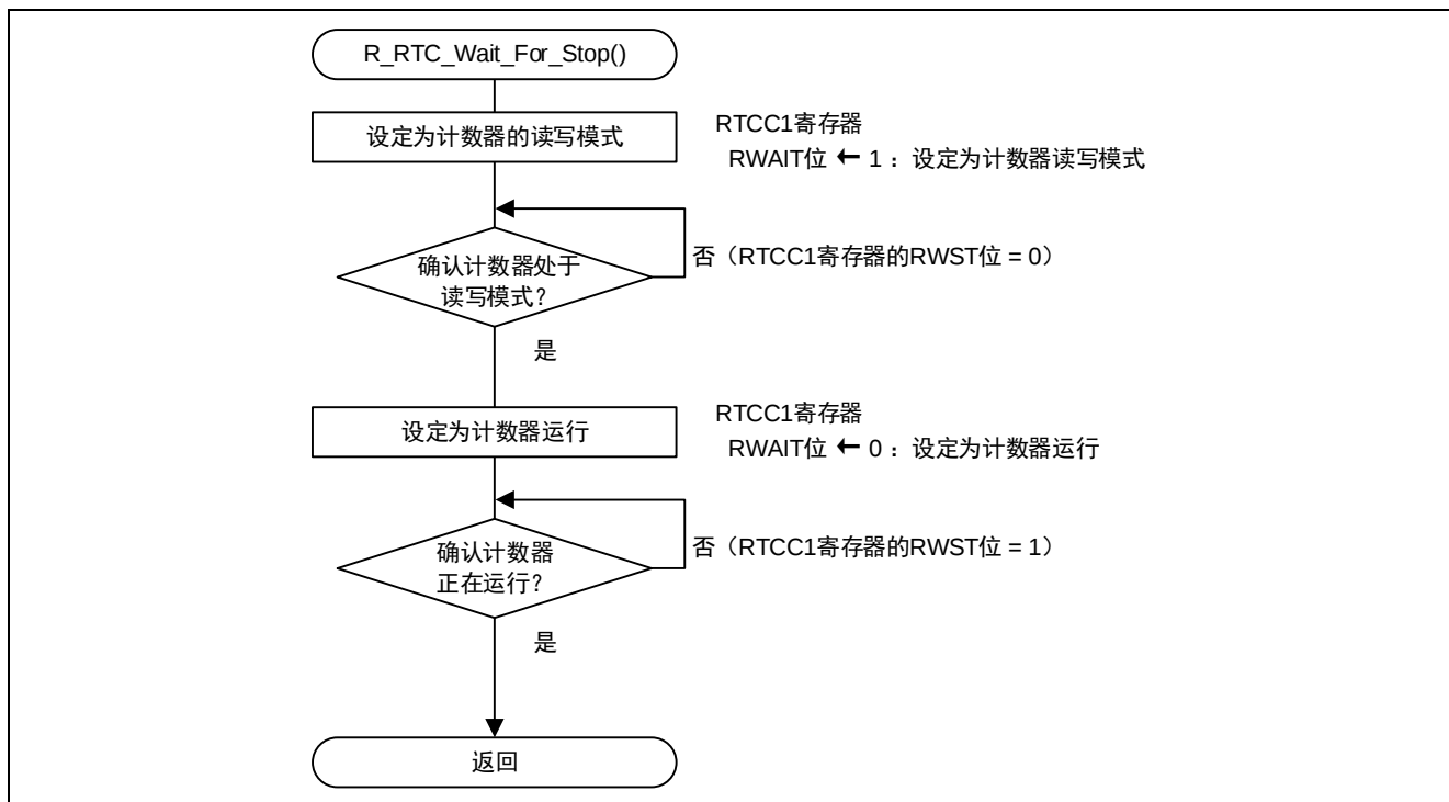
图 5.13 转移到 STOP 模式前的等待处理
