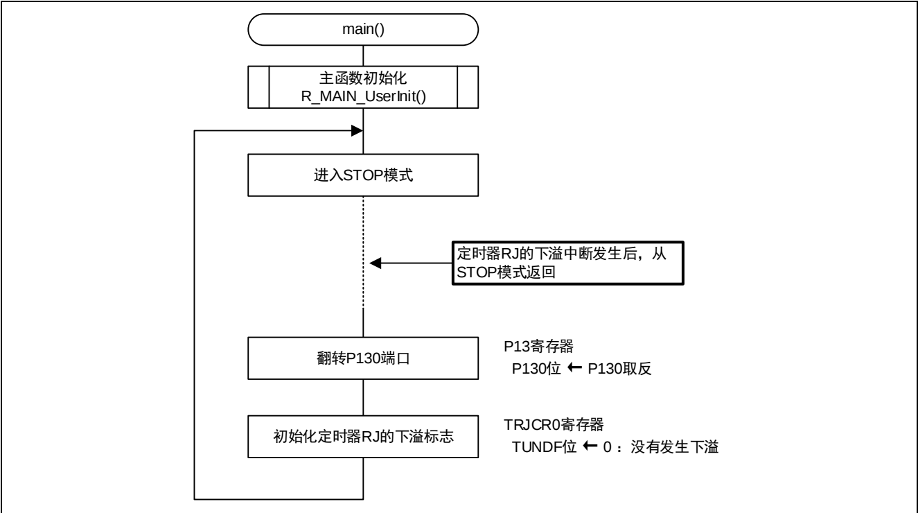
图 5.10 主函数处理
