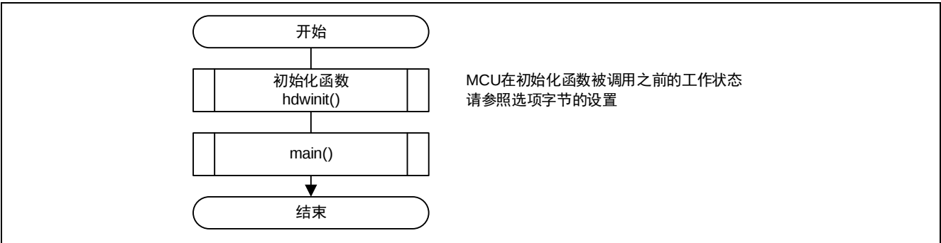
图 5.2 整体流程图
