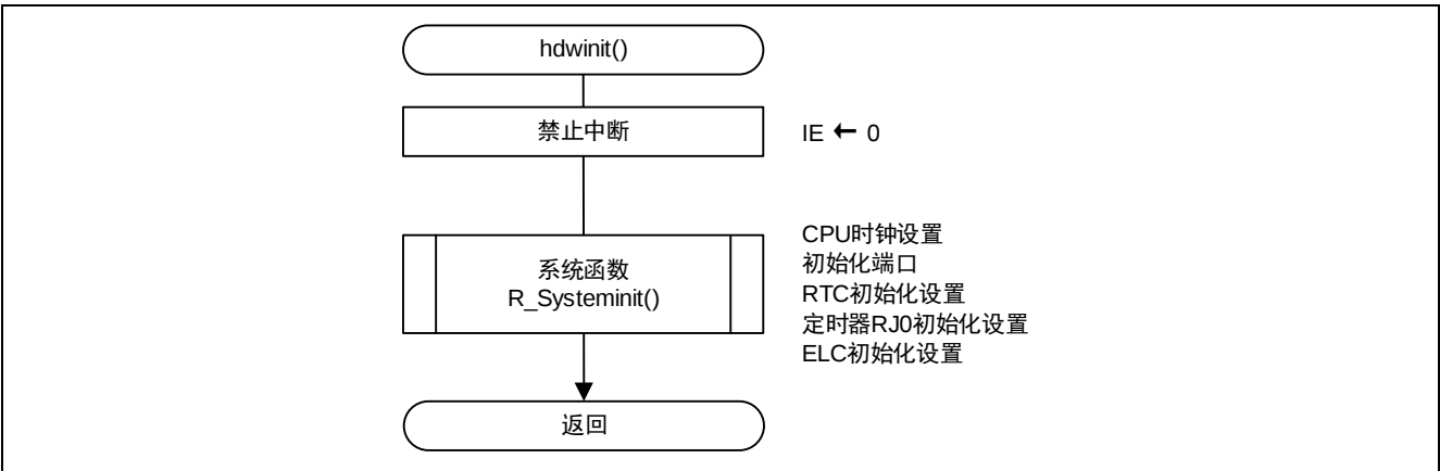
图 5.3 初始化函数
