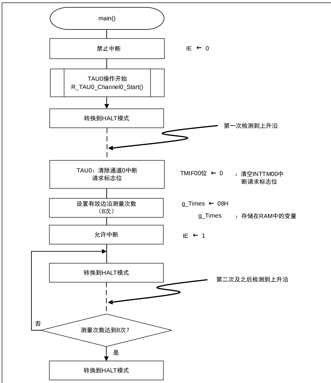
图 4.6 主函数处理
