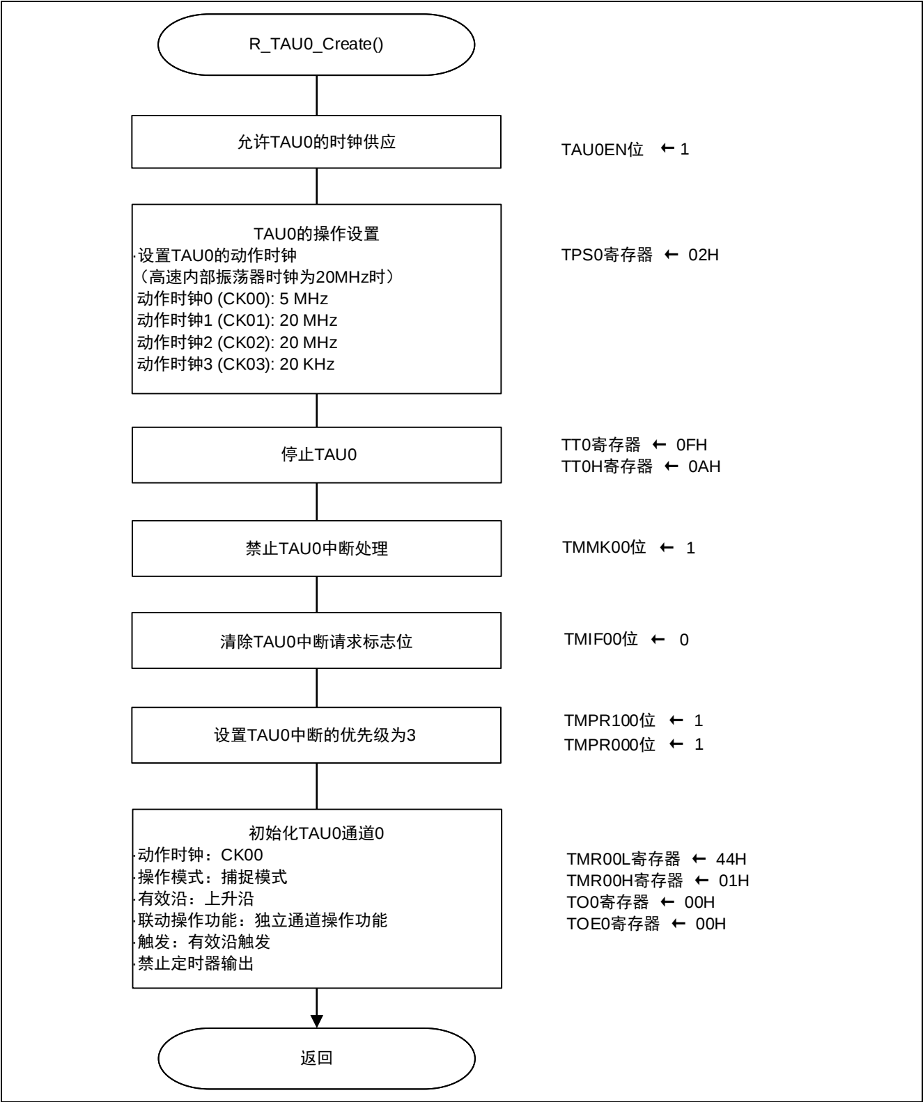
图 4.5 TAU0 初始化
