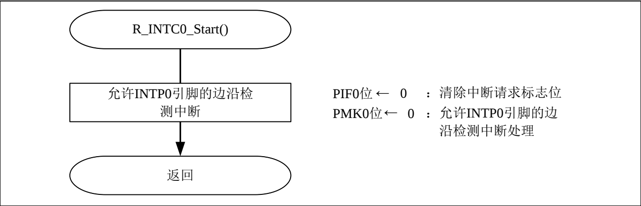
图 4.8 INTP0 操作开始
