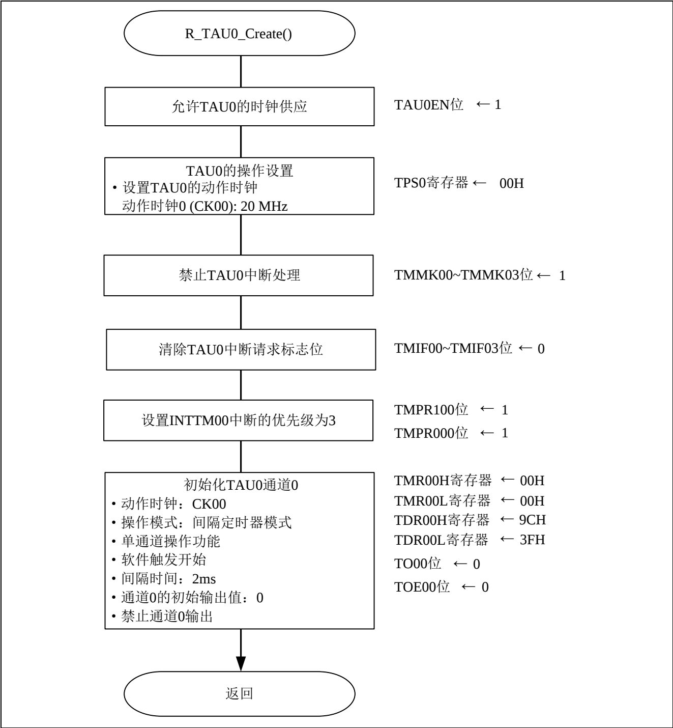
图 4.5 定时器阵列单元初始化
