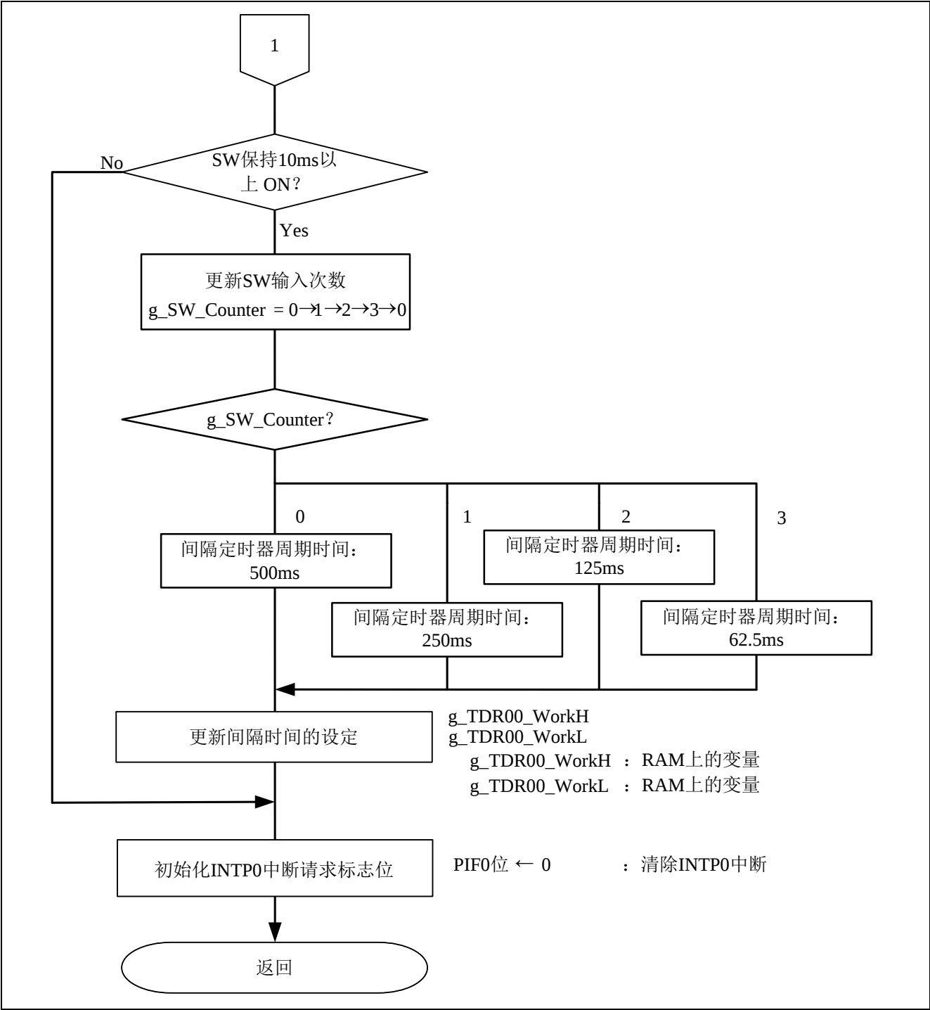
图 4.13 INTPO 中断处理 (2/2)
