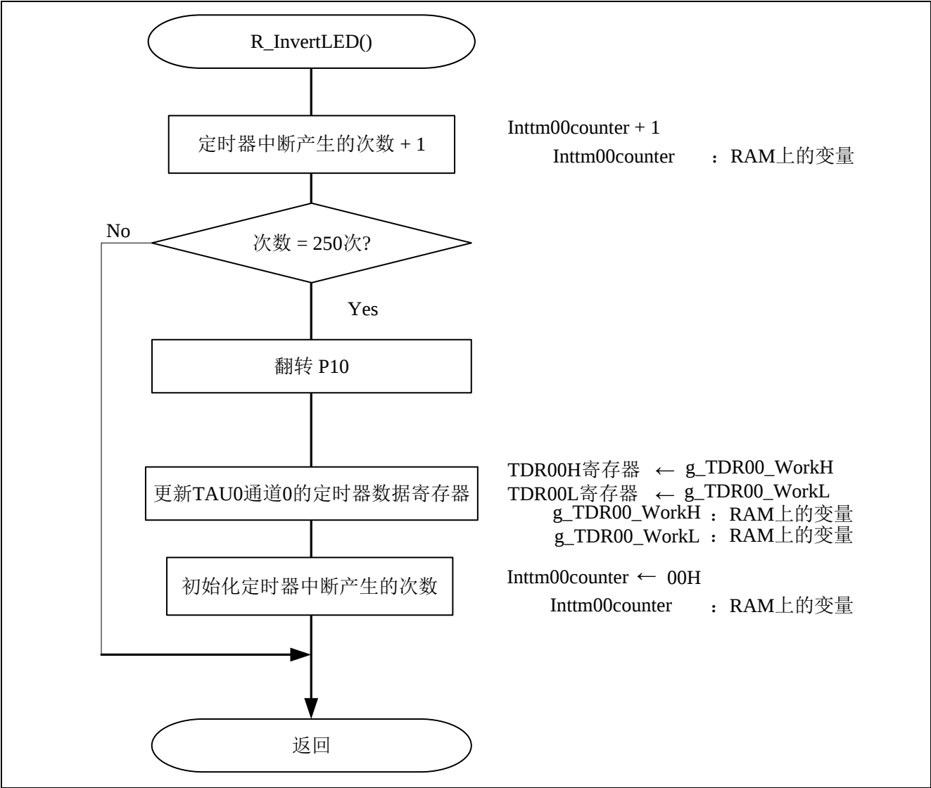
图 4.11 LED 开/关处理
