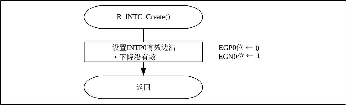
图 4.6 INTP0 初始化
