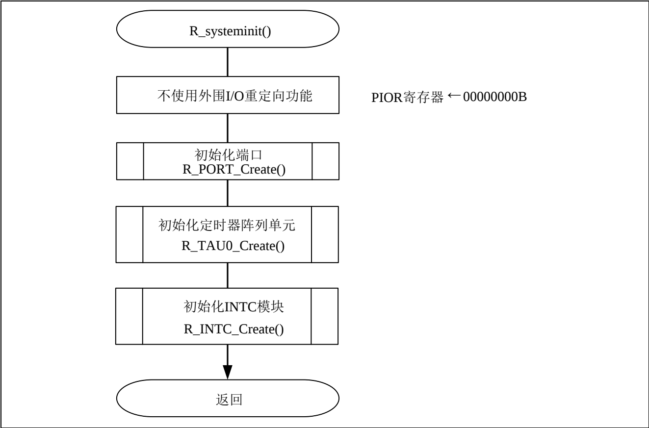
图 4.3 系统函数
