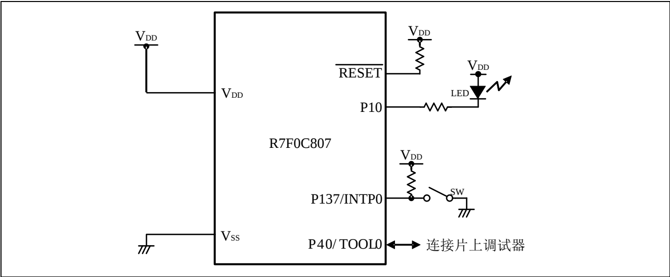
图 4.1 硬件配置
