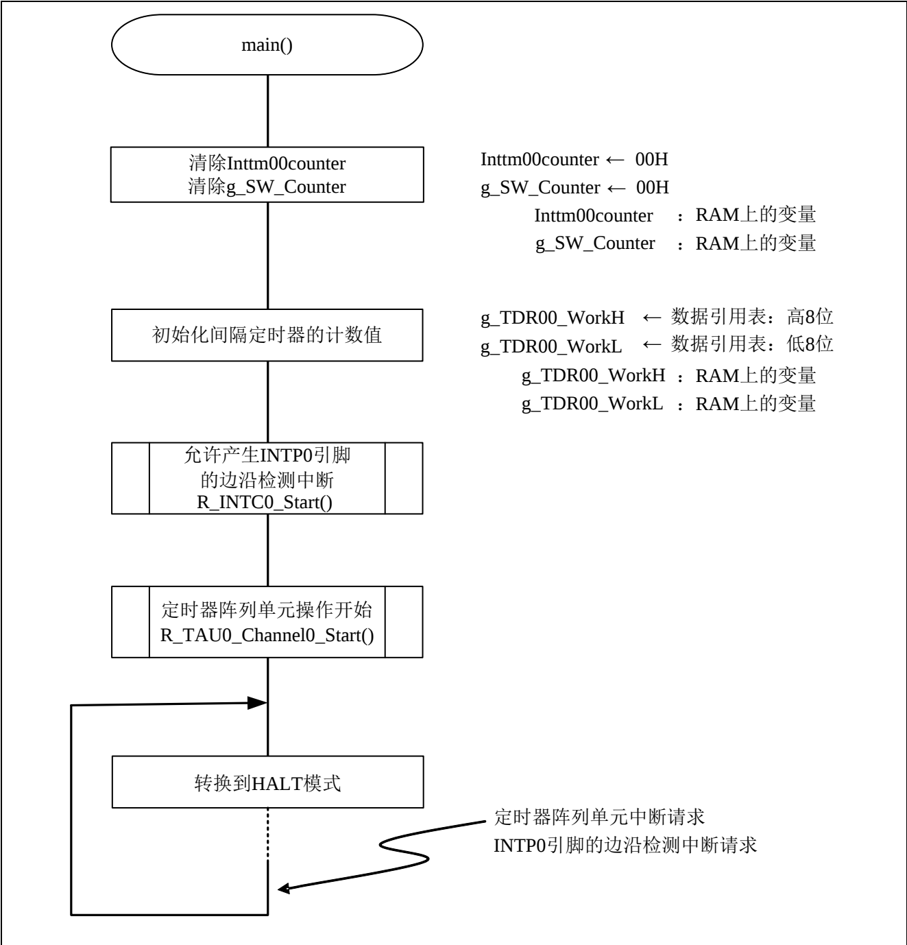
图 4.7 主函数处理
