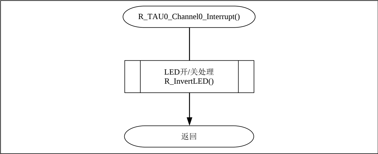
图 4.10 TAU0 通道 0 定时器中断处理
