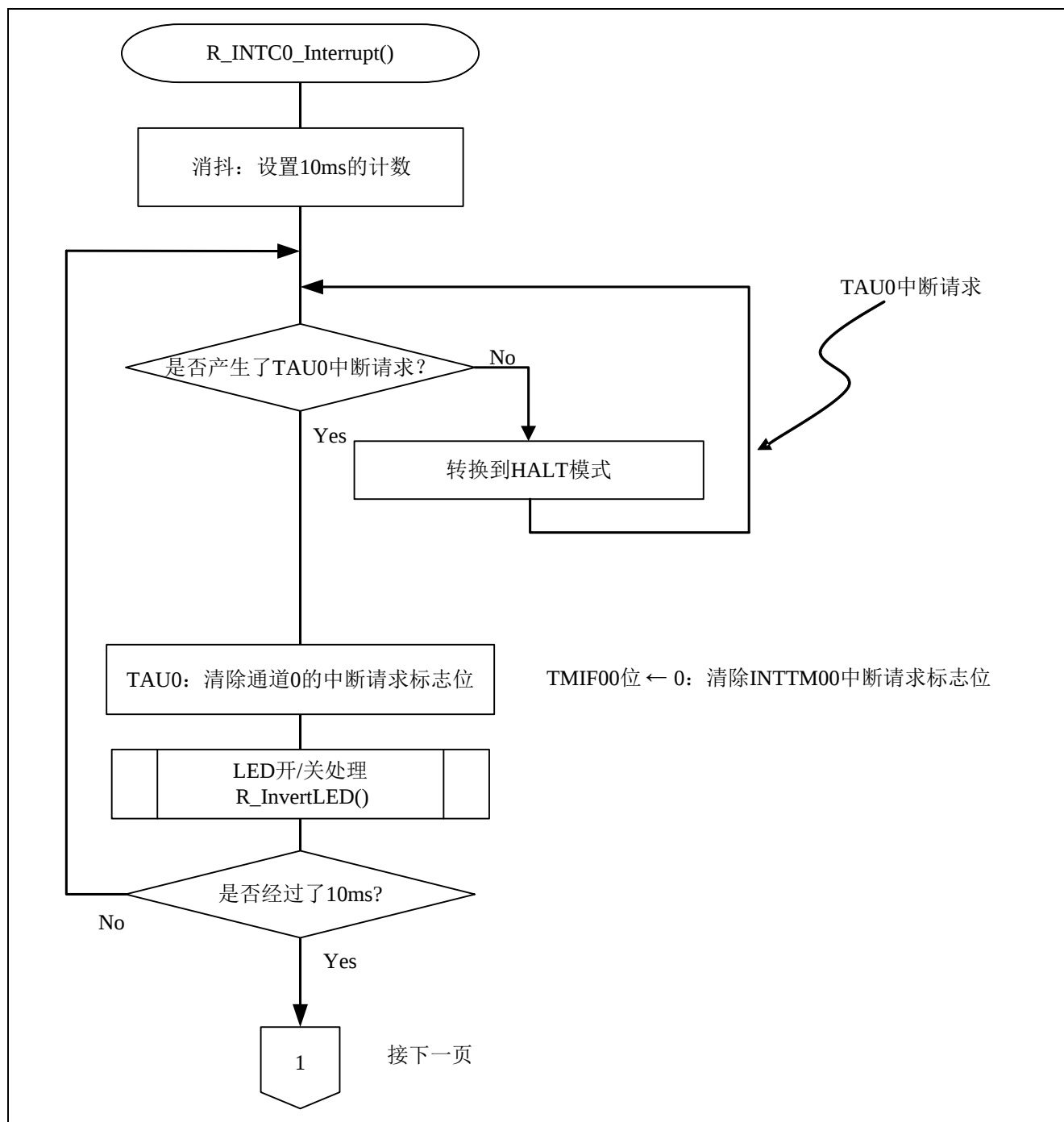
图 4.12 INTP0 中断处理（1/2）
