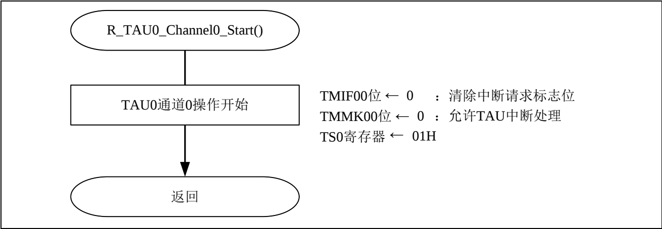
图 4.9 TAU0 通道 0 操作开始
