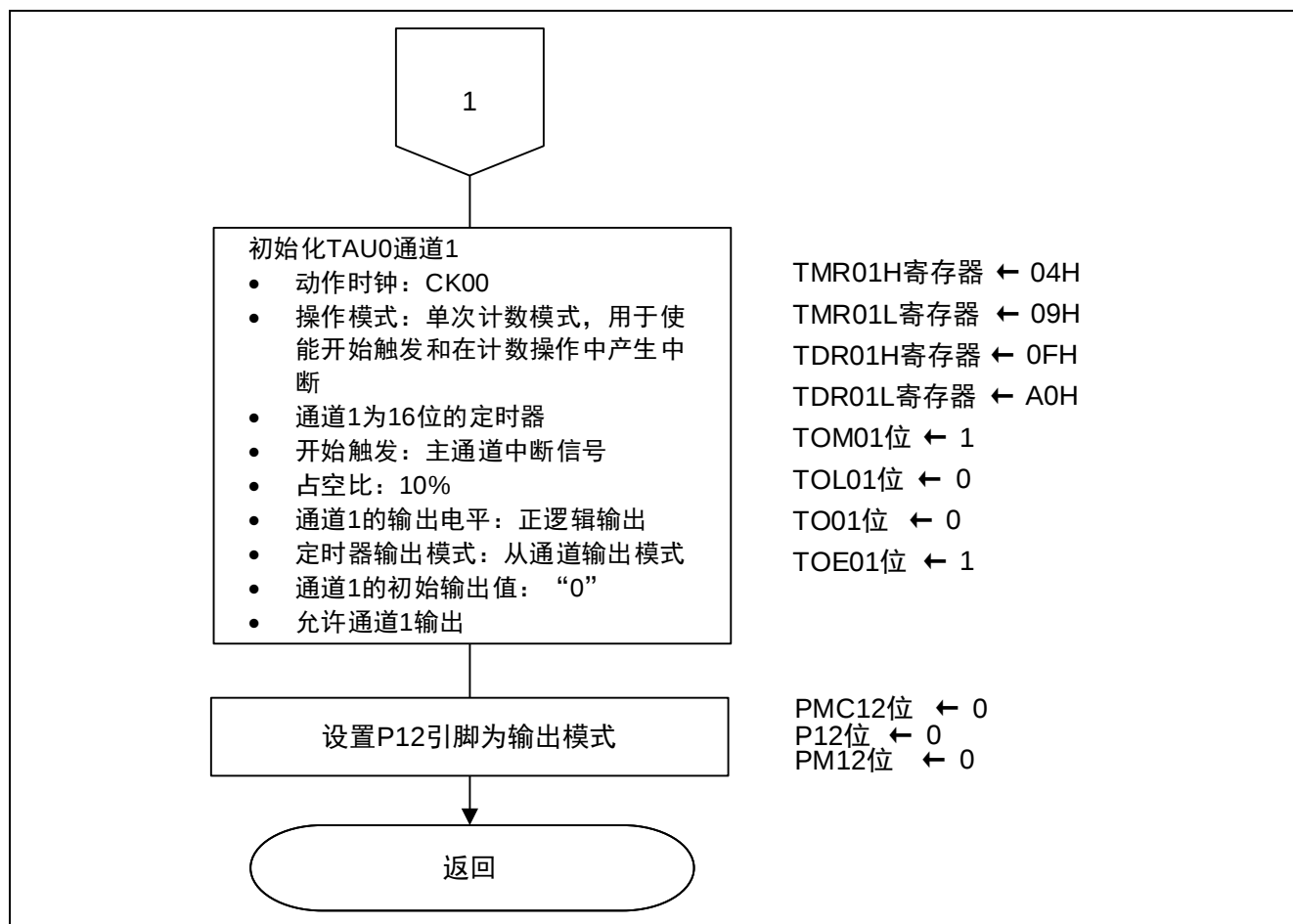
图 4.6 TAU0 初始化设置（2/2）
