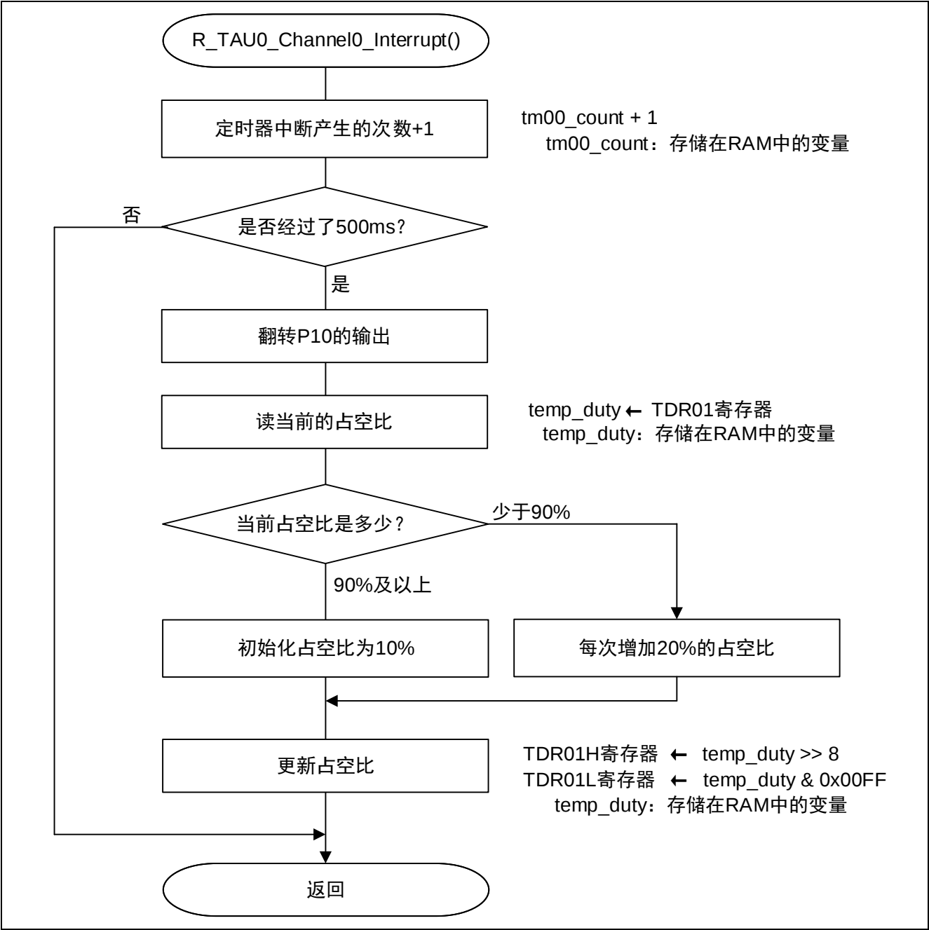
图 4.9 TAU0 通道 0 中断处理
