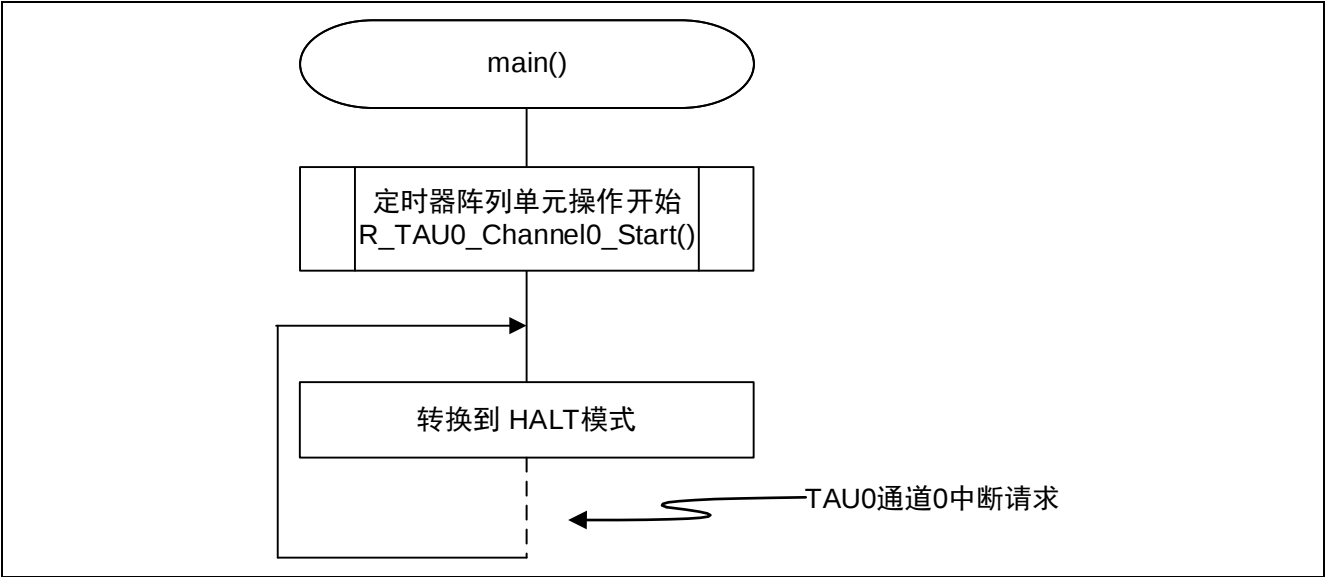
图 4.7 主函数处理
