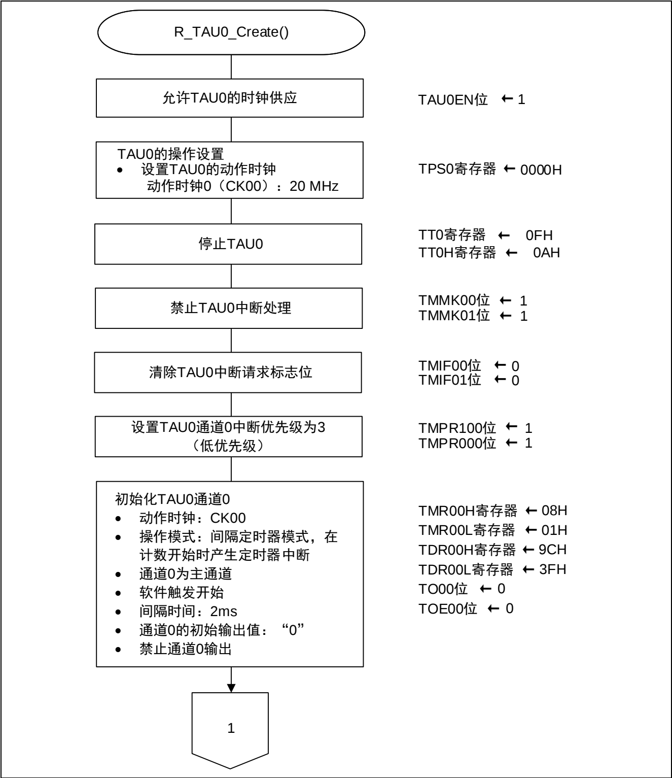
图 4.5 TAU0 初始化设置（1/2）
