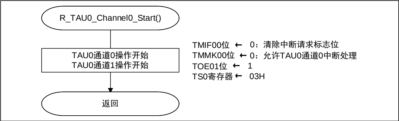
图 4.8 TAU0 操作开始
