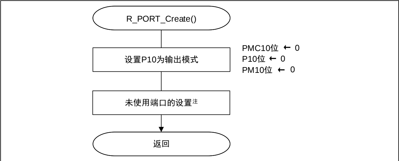
图 4.4 初始化端口
