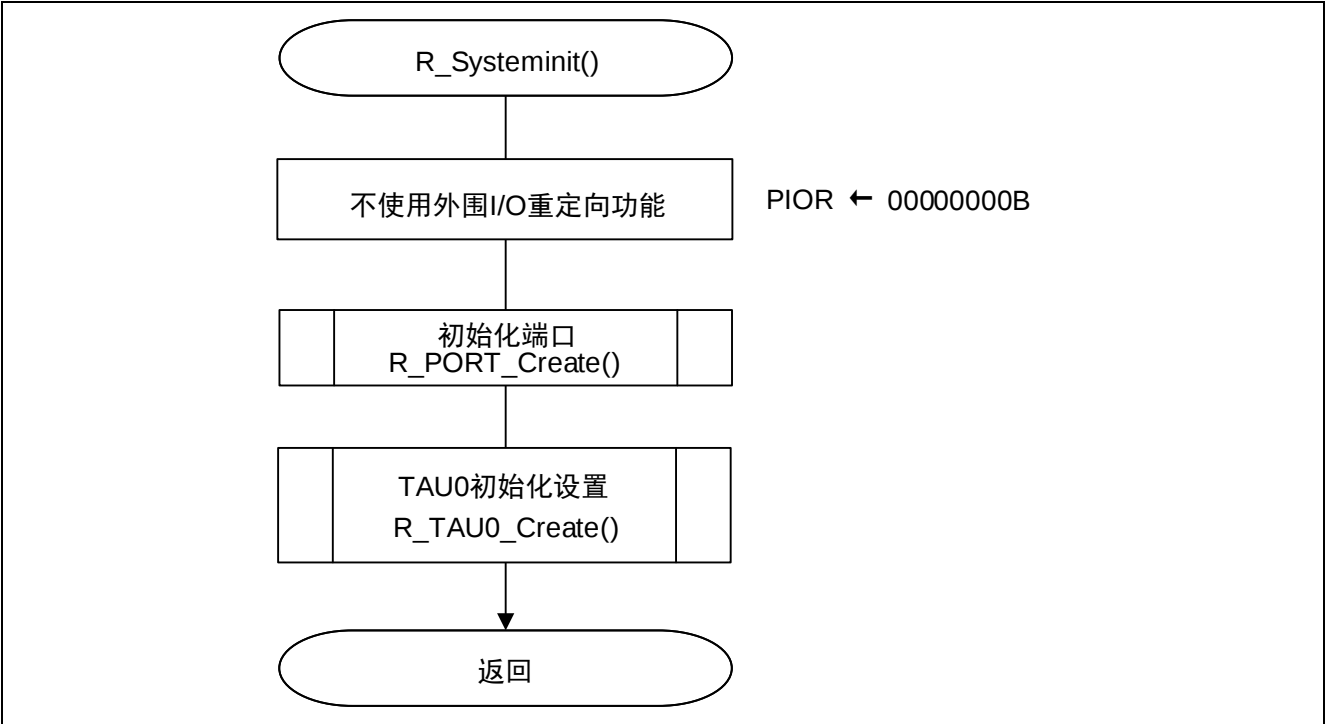
图 4.3 系统函数
