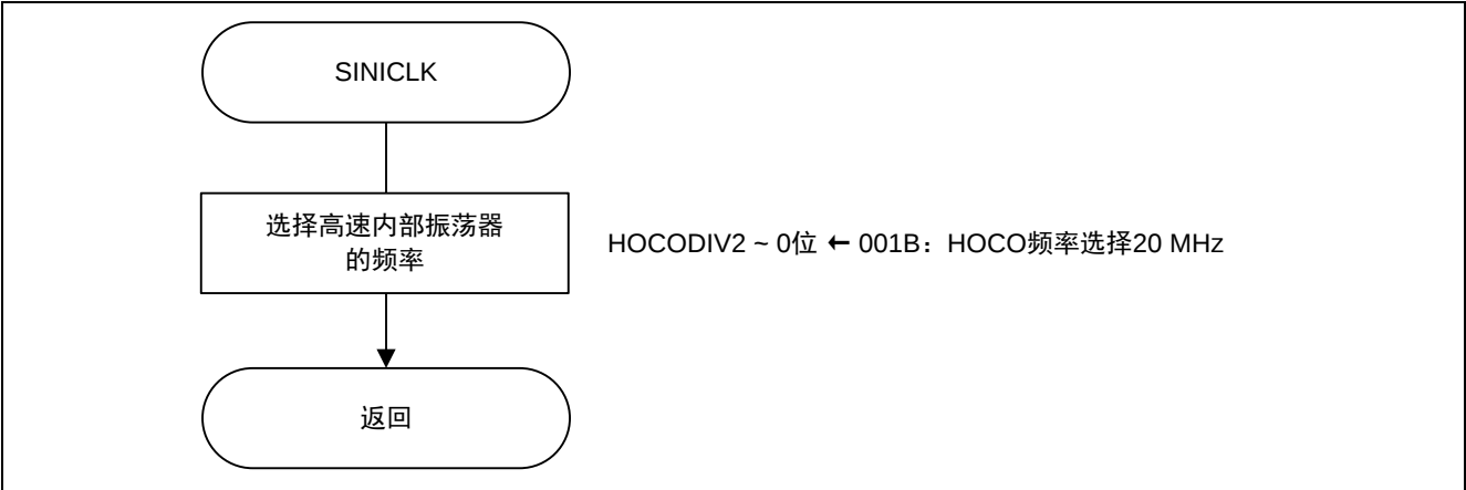
图 4.4 设置时钟发生电路
