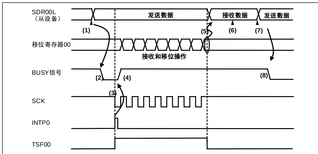
图 1.3 从设备通过 SCK 的检测控制 BUSY 信号的例子
