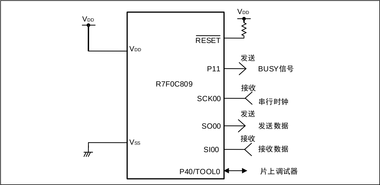
图 4.1 硬件配置
