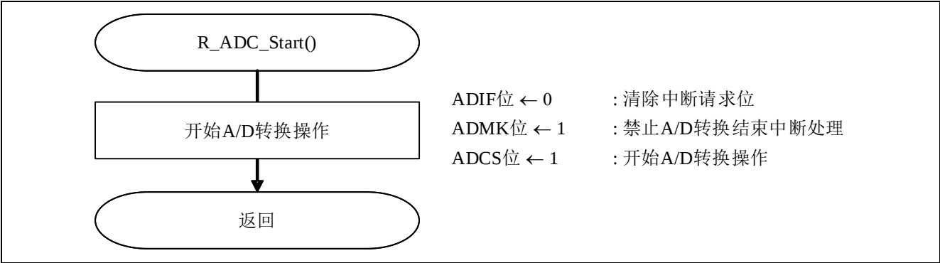
图 4.8 开始 A/D 转换
