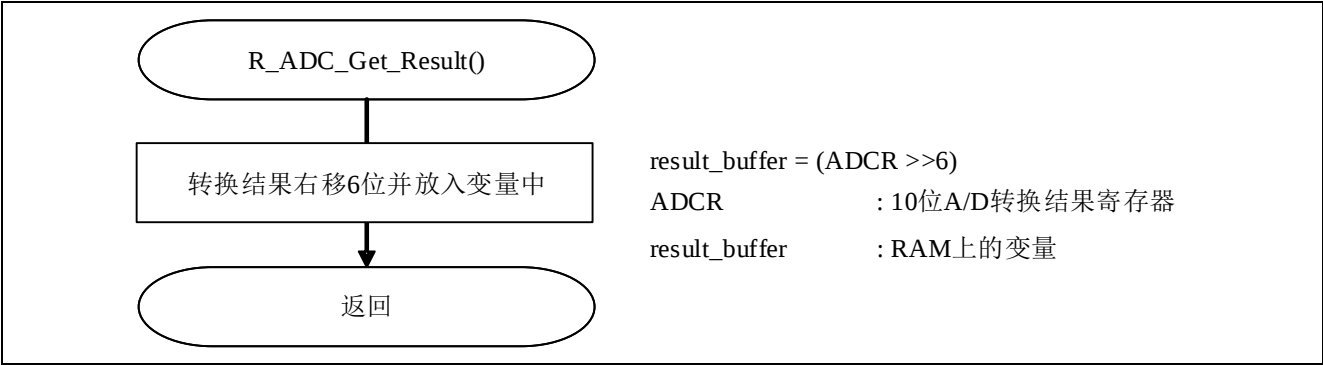
图 4.9 保存 A/D 转换结果
