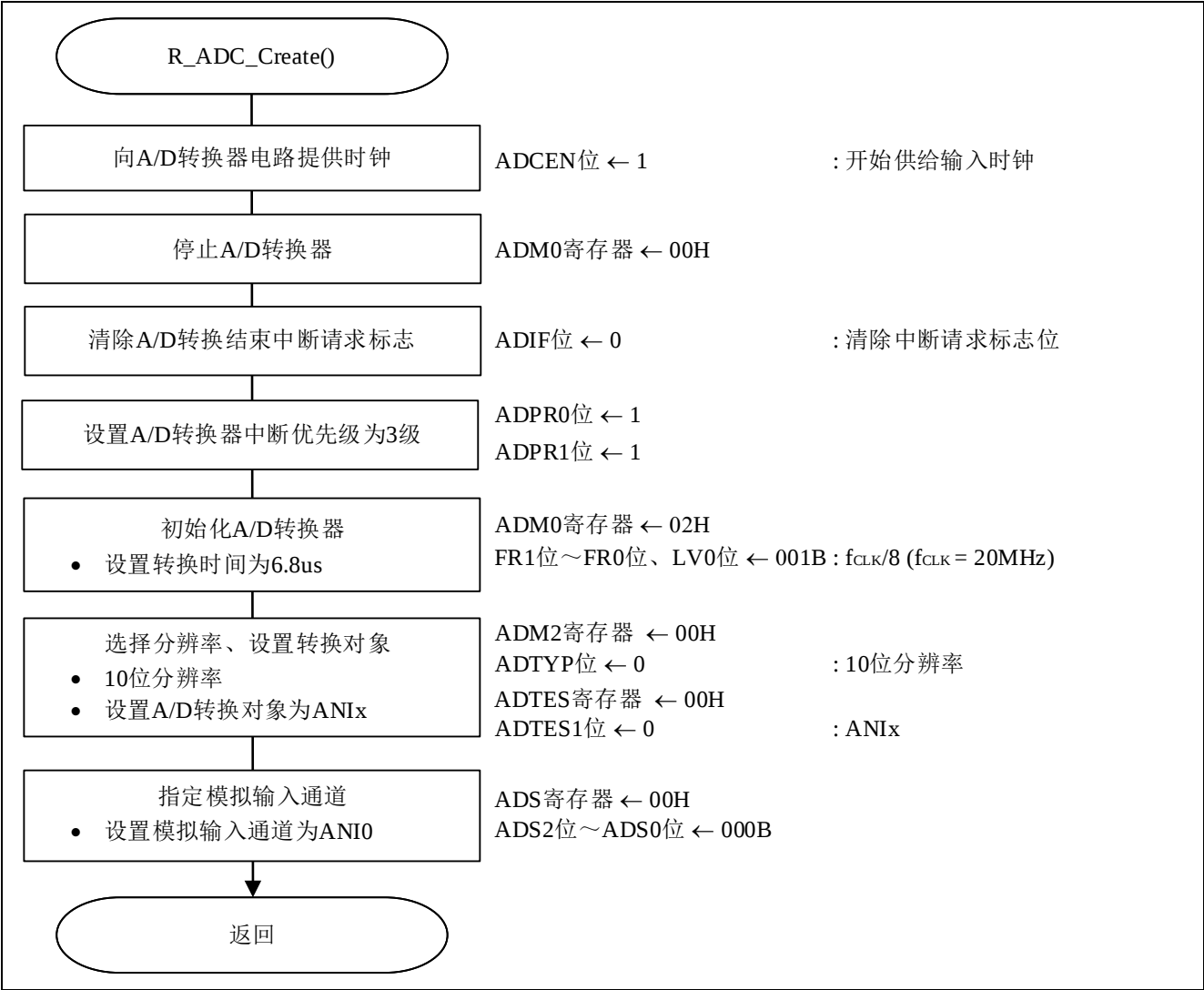
图 4.5 A/D 转换器的初始化设置
