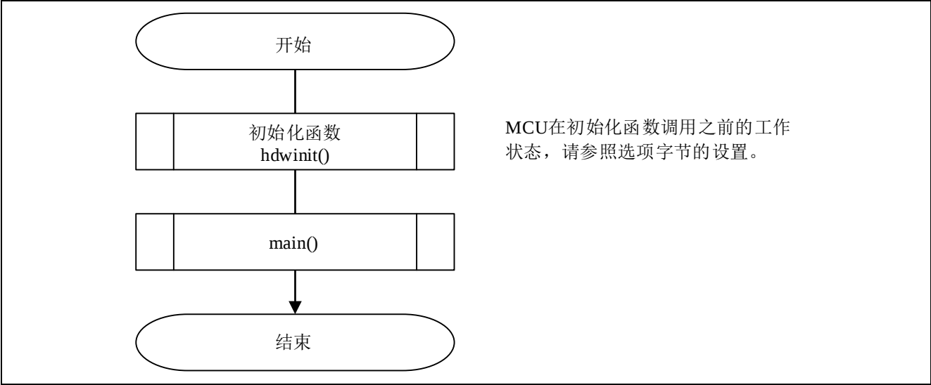
图 4.1 整体流程
