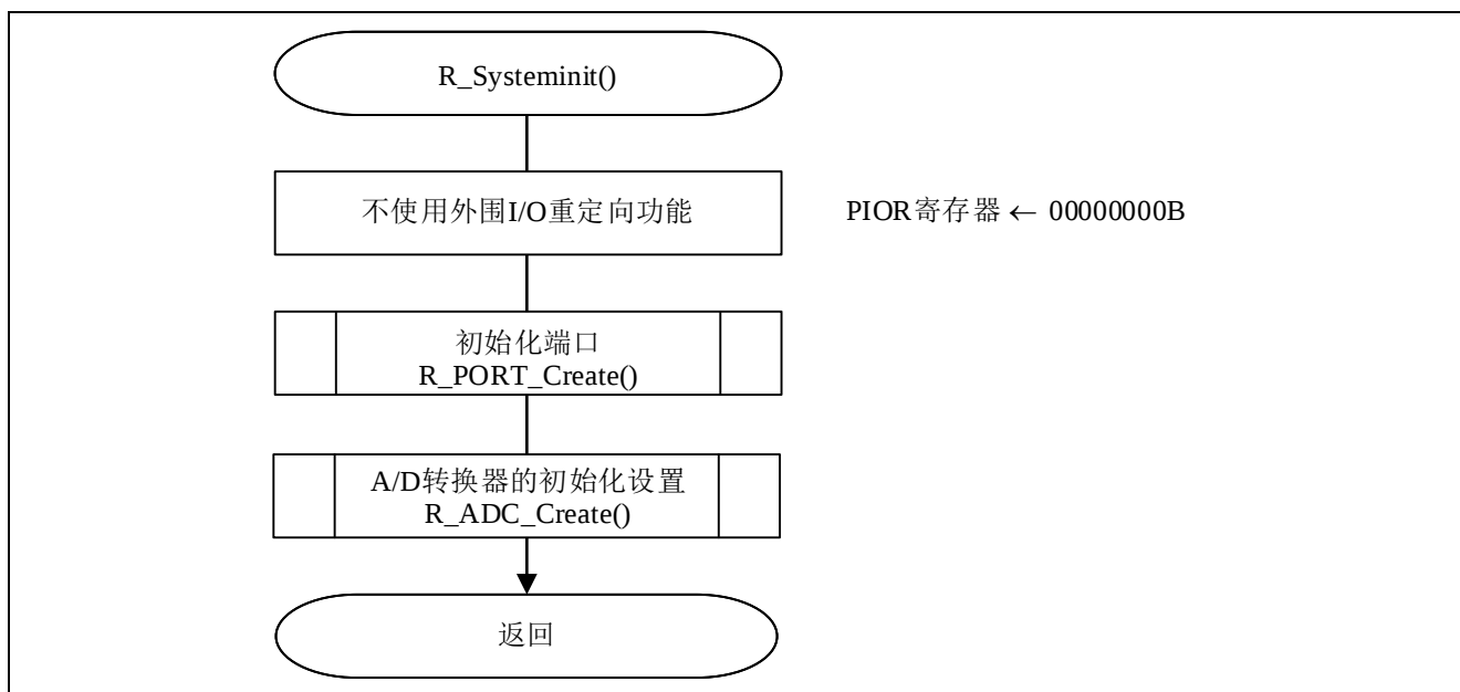
图 4.3 系统函数
