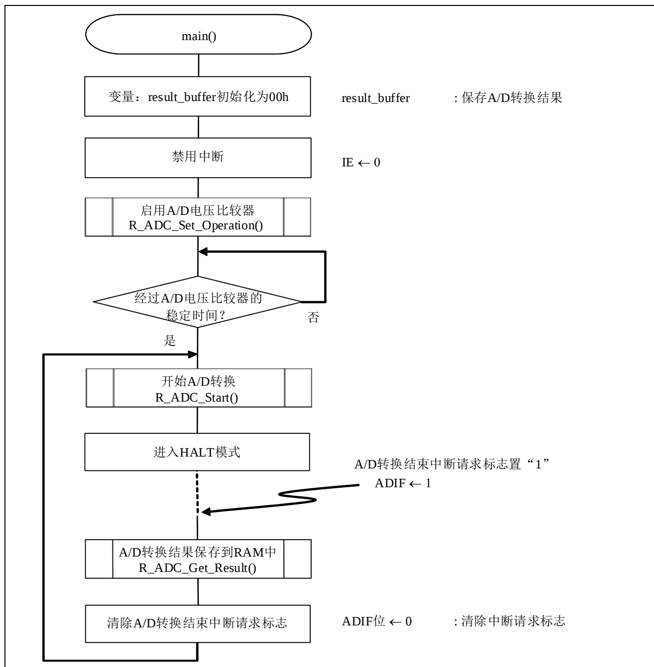
图 4.6 主函数处理
