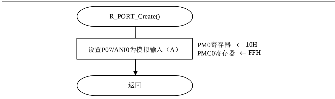
图 4.4 初始化端口
