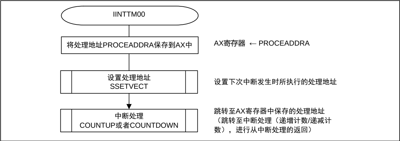
图 4.8 INTTM00 中断处理
