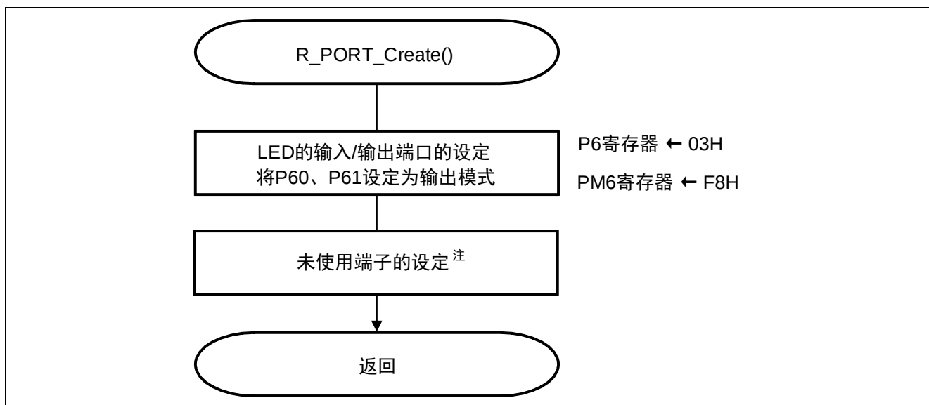
图 5.4 初始化端口
