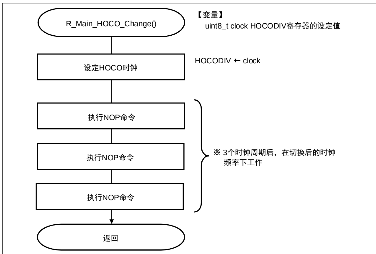
图 5.20 切换 HOCO 时钟
