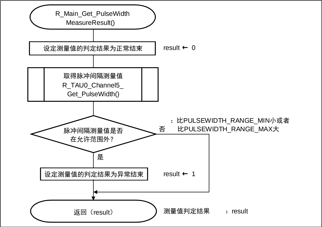
图 5.16 判断脉冲间隔测量结果
