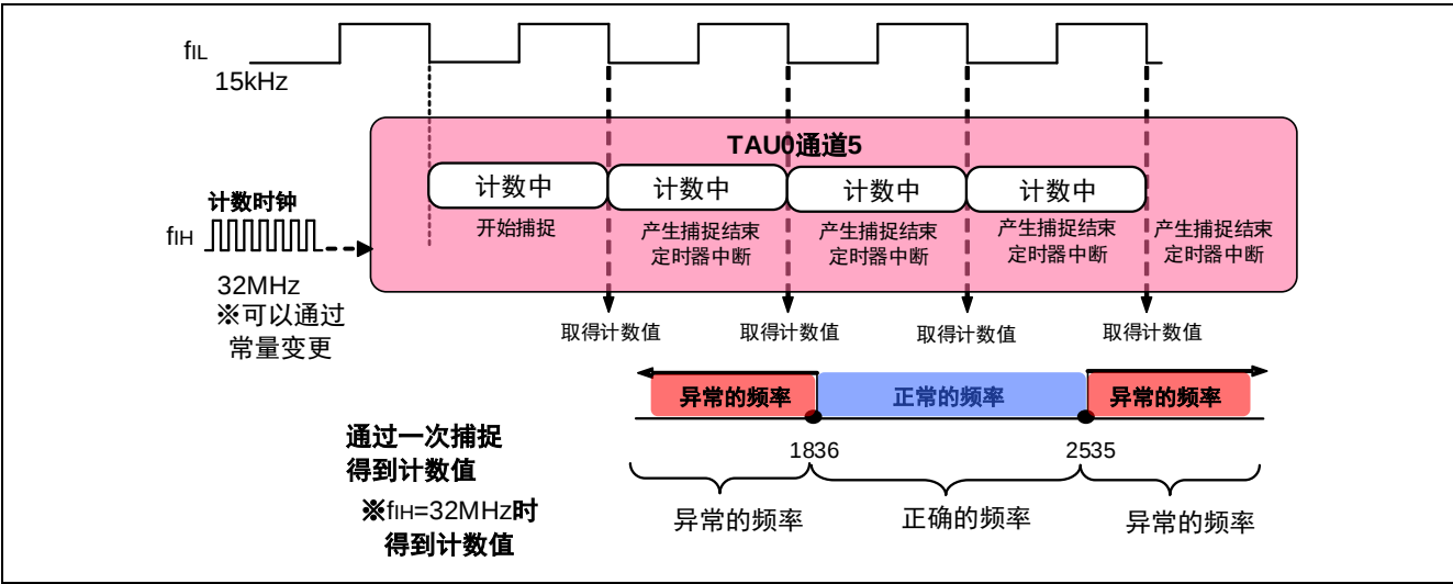
图 1.1 频率检出的动作概要
