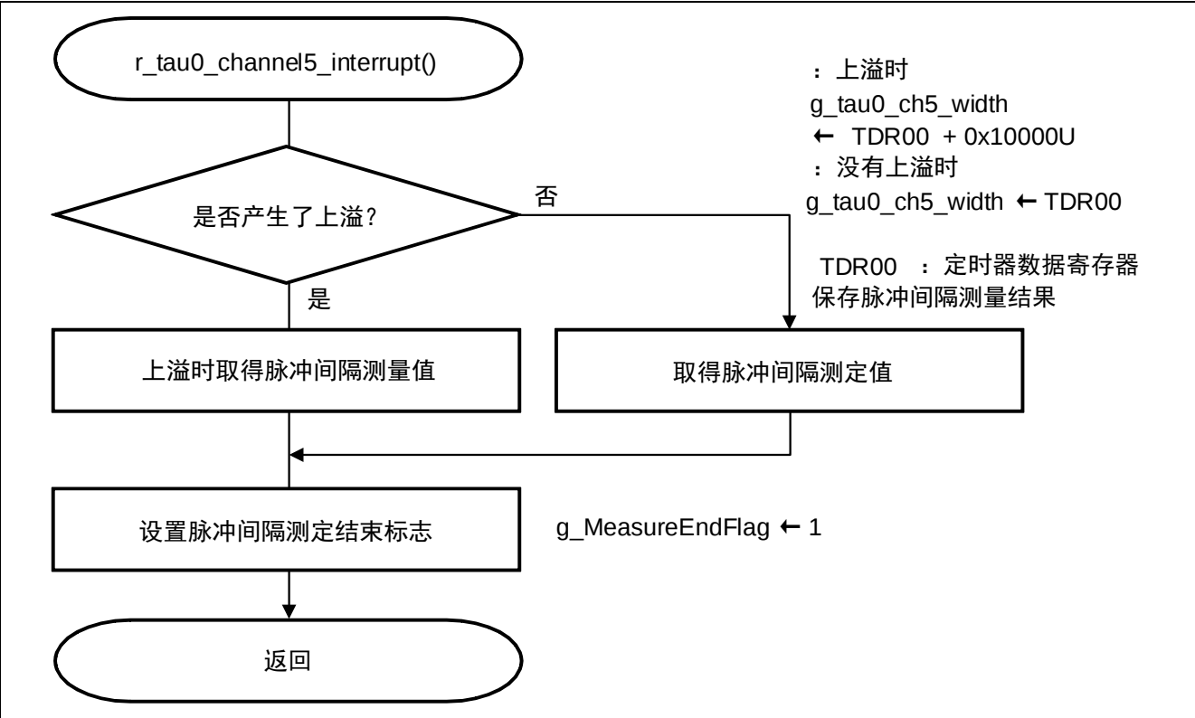
图 5.23 TAU0 通道 5 捕捉结束中断处理
