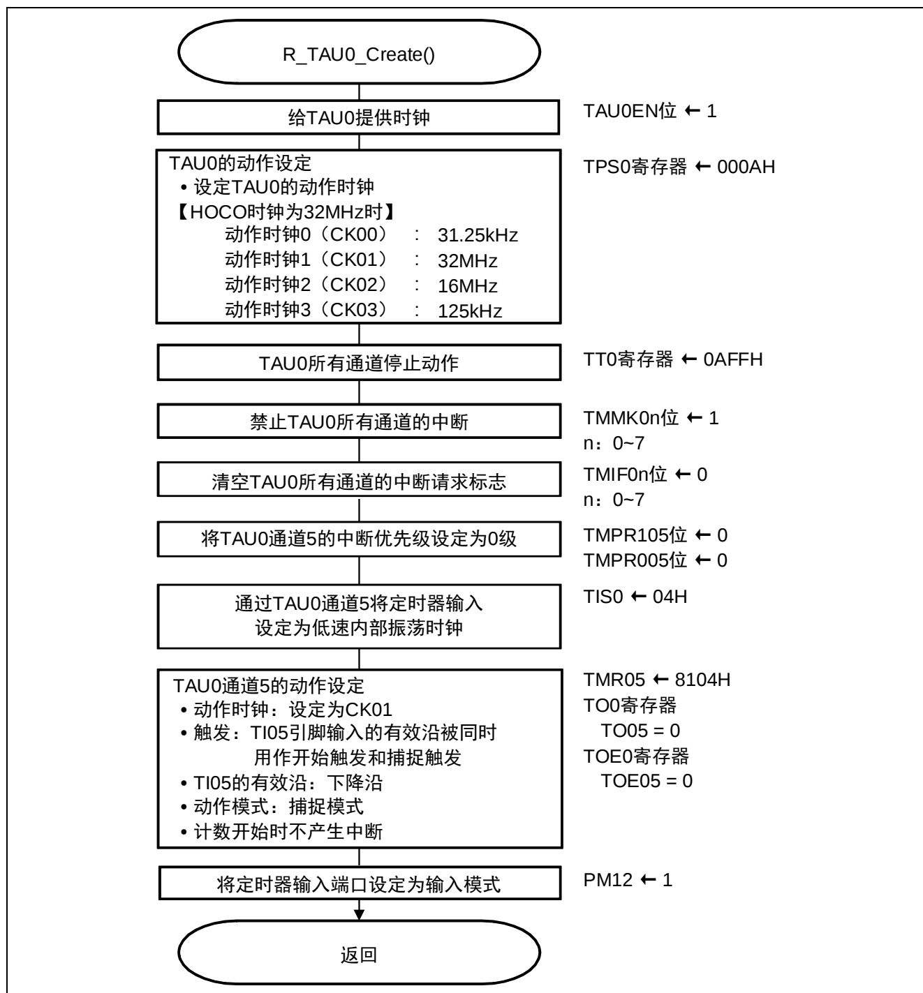
图 5.6 TAU0 的初始化设置
