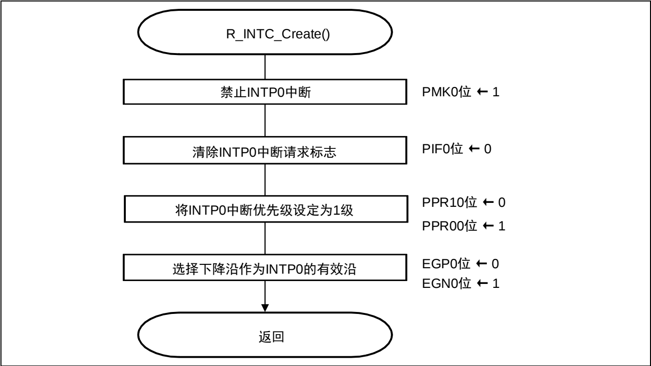
图 5.8 外部中断输入的初始化设置
