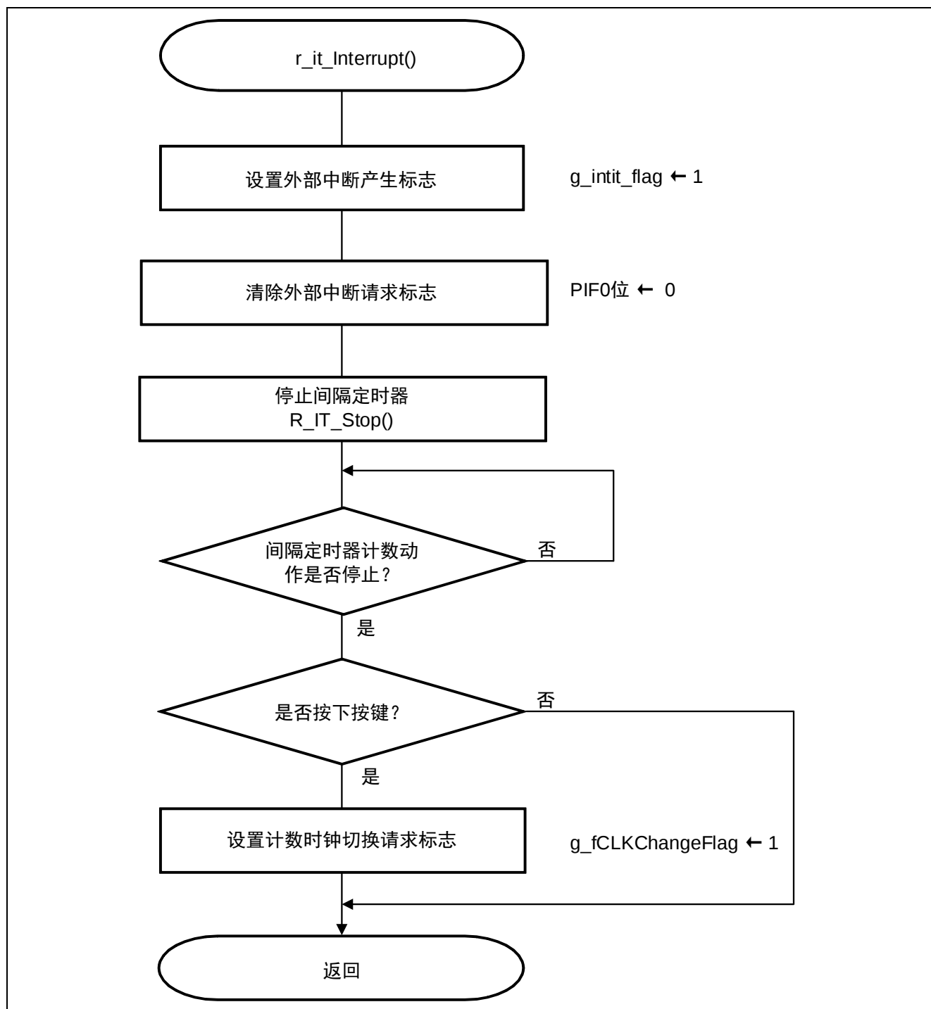
图 5.22 间隔定时器中断处理
