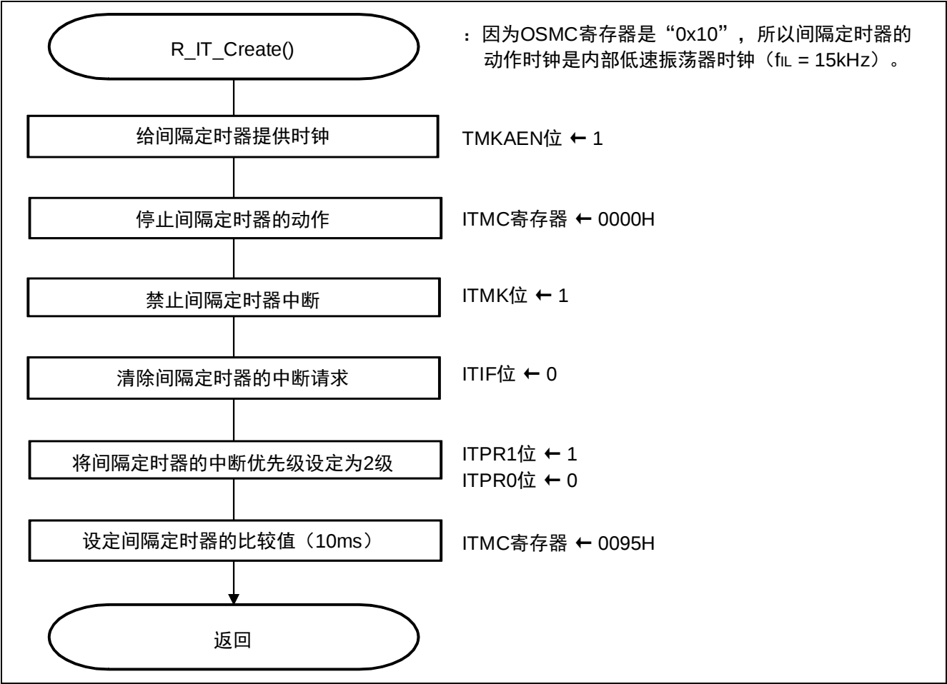
图 5.7 间隔定时器的初始化设置
