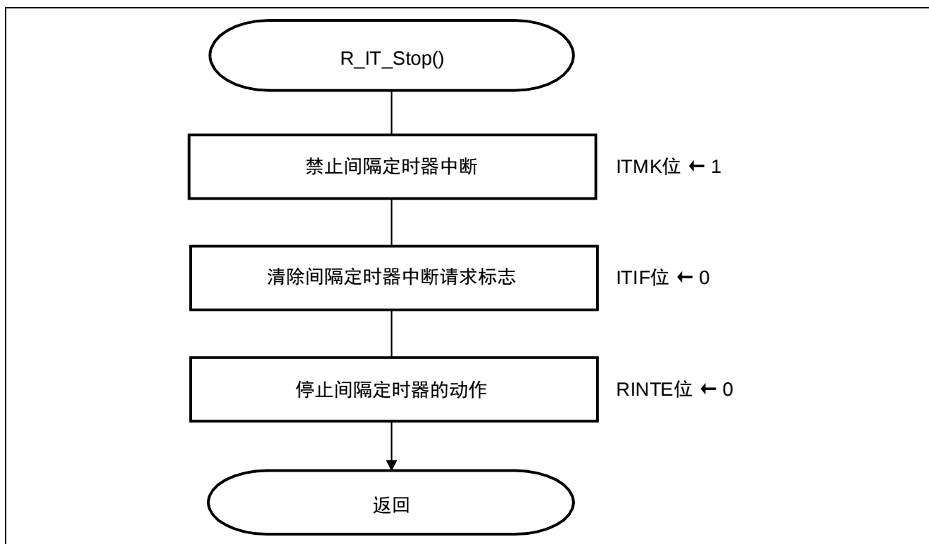
图 5.26 停止间隔定时器
