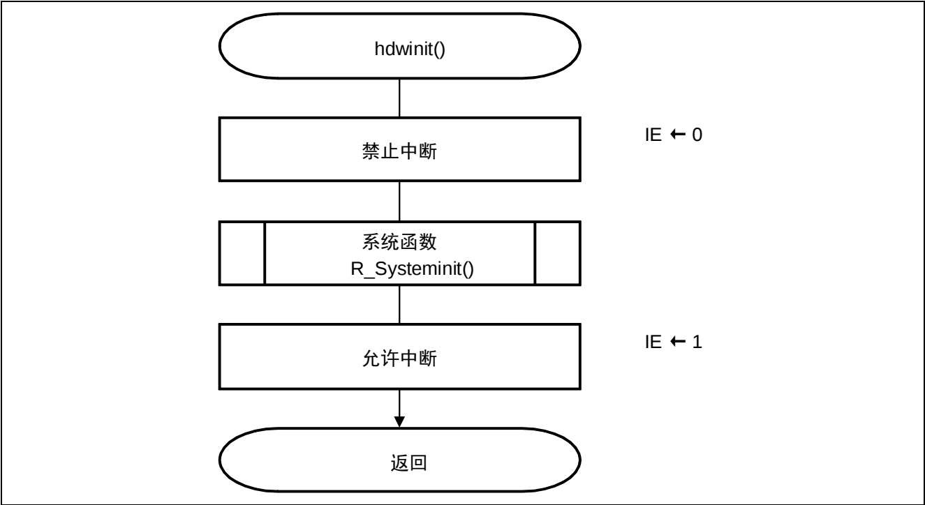
图 5.2 初始化函数
