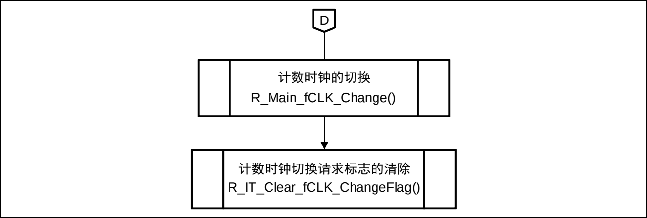
图 5.9 主函数处理（3/3）
