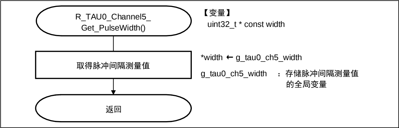
图 5.17 取得脉冲间隔测量值
