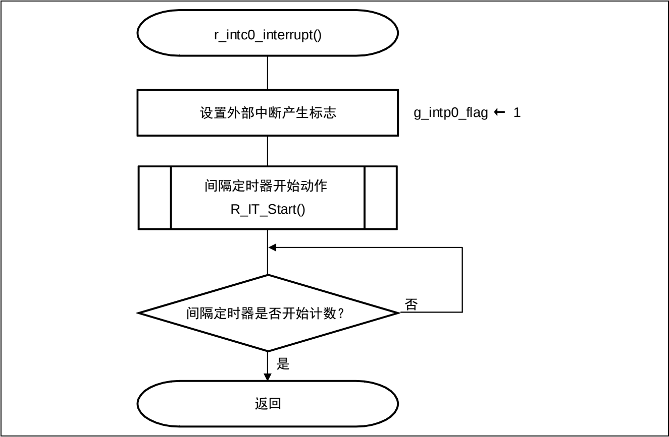
图 5.24 INTP0 外部中断处理
