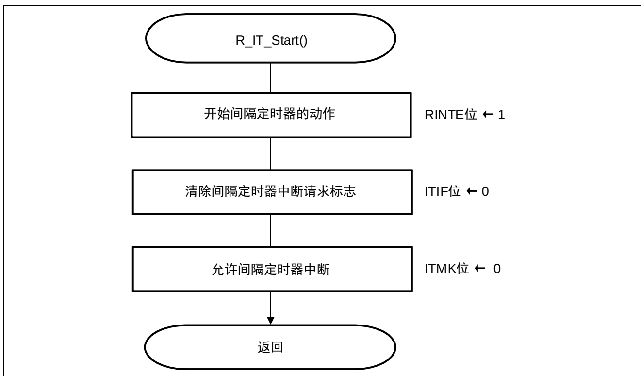
图 5.25 启动间隔定时器
