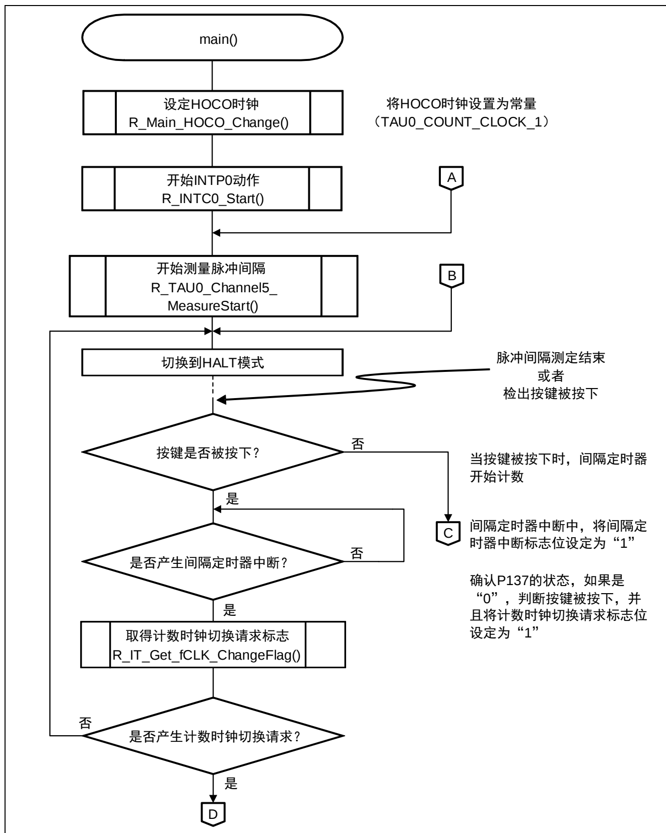
图 5.9 主函数处理 (1/3)
