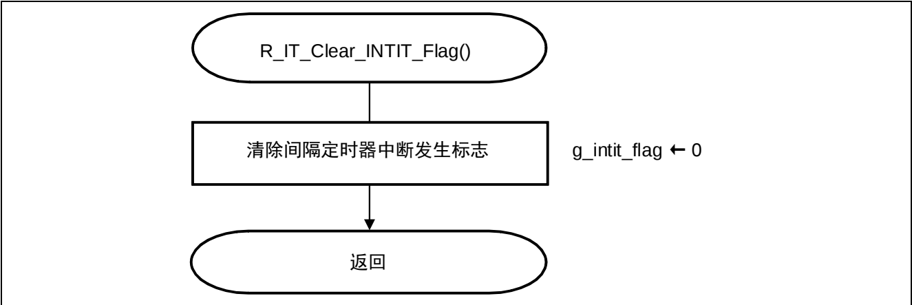
图 5.30 清除间隔定时器中断产生标志
