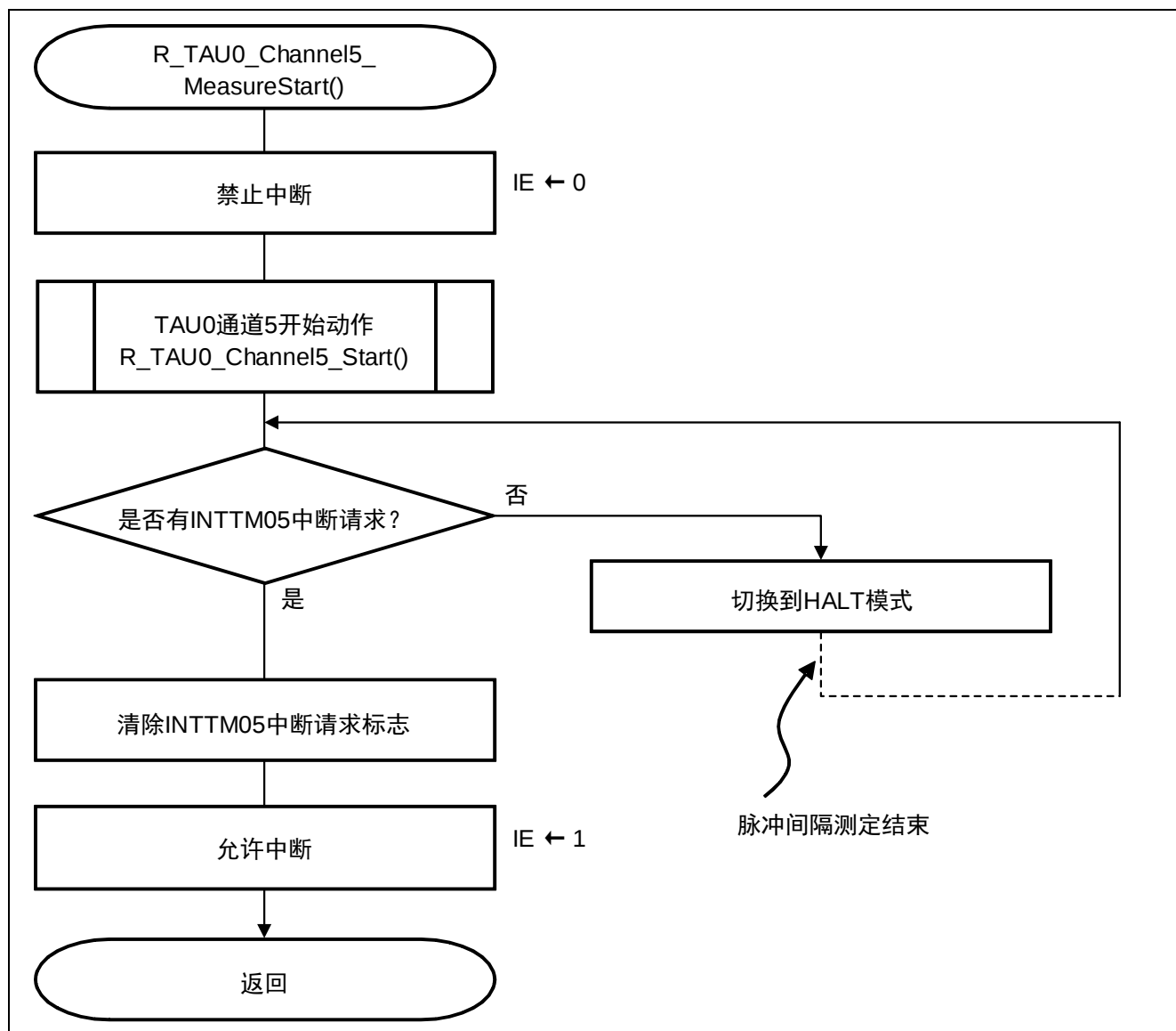
图 5.11 启用脉冲间隔测量
