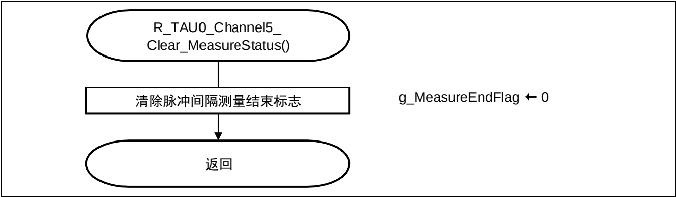
图 5.18 清除脉冲间隔测量结束标志
