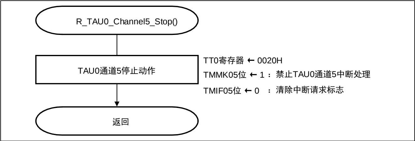
图 5.13 停止 TAU0 通道 5
