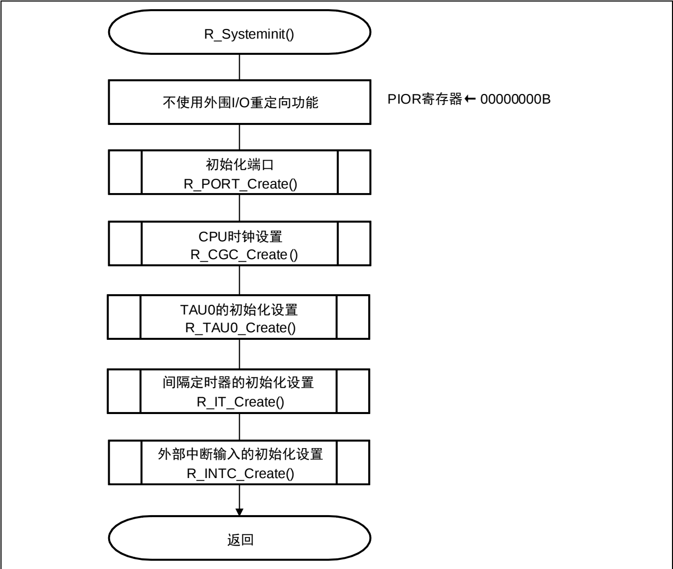
图 5.3 系统函数
