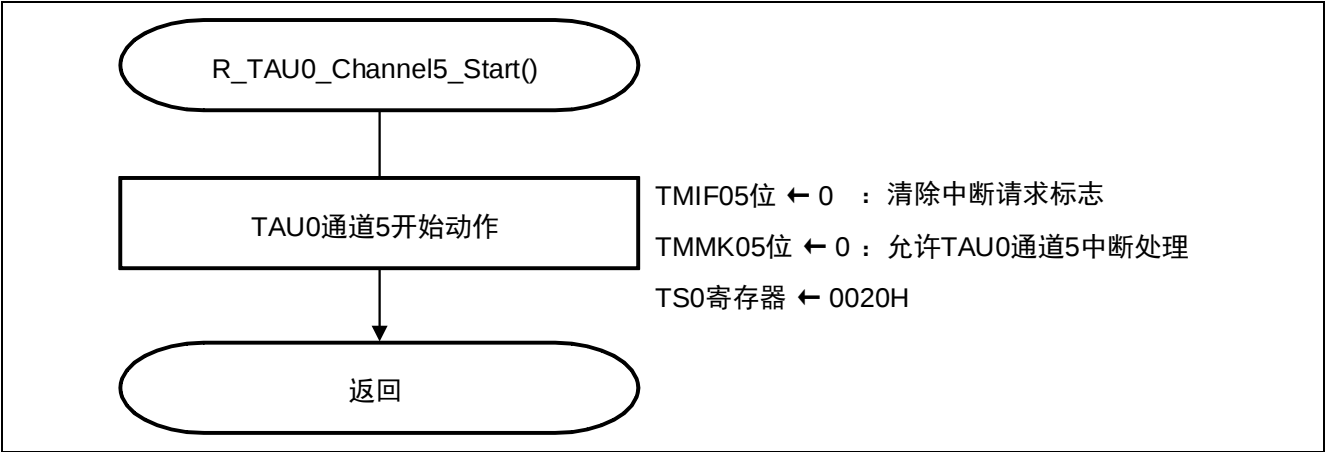
图 5.12 启用 TAU0 通道 5
