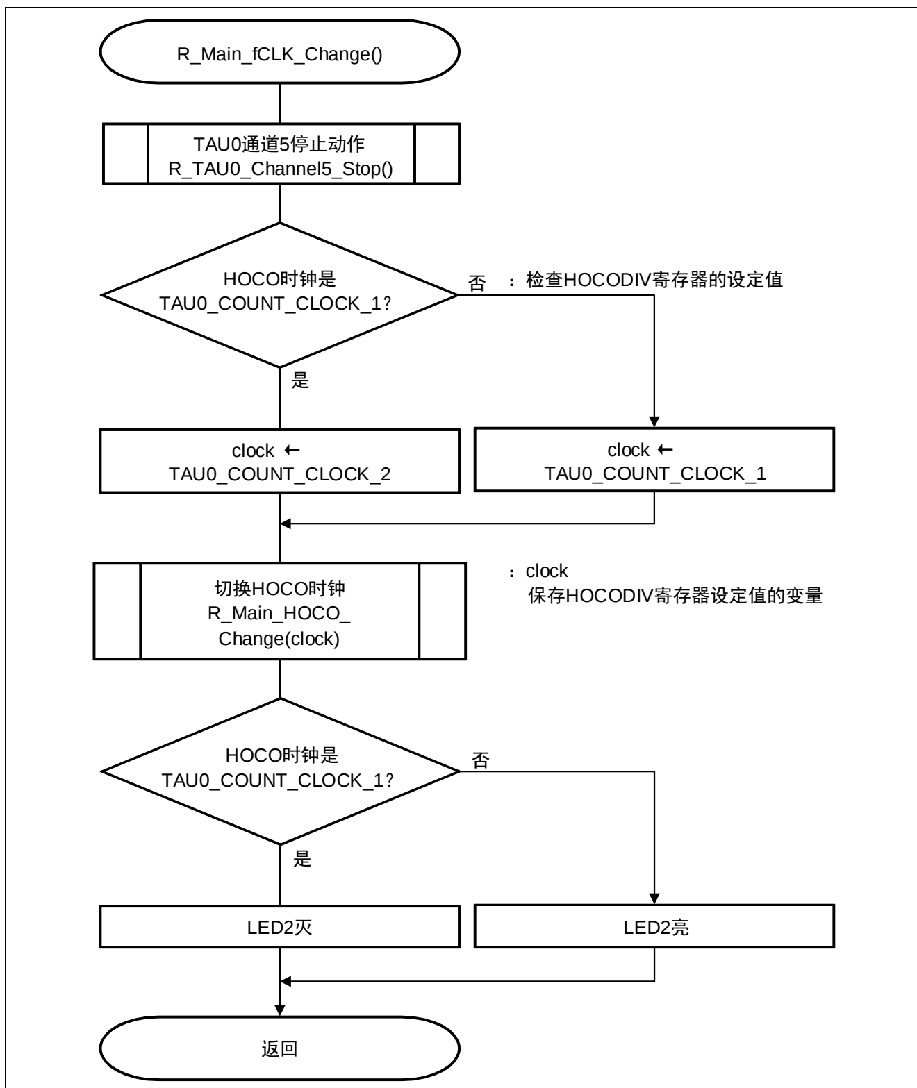
图 5.19 切换计数时钟
