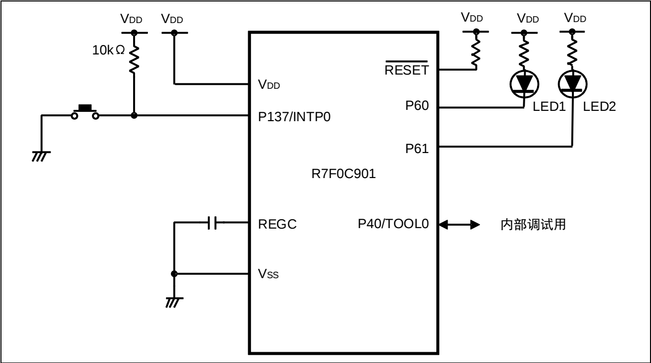
图 4.1 硬件配置
