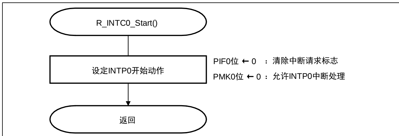
图 5.10 启用 INTP0 外部中断
