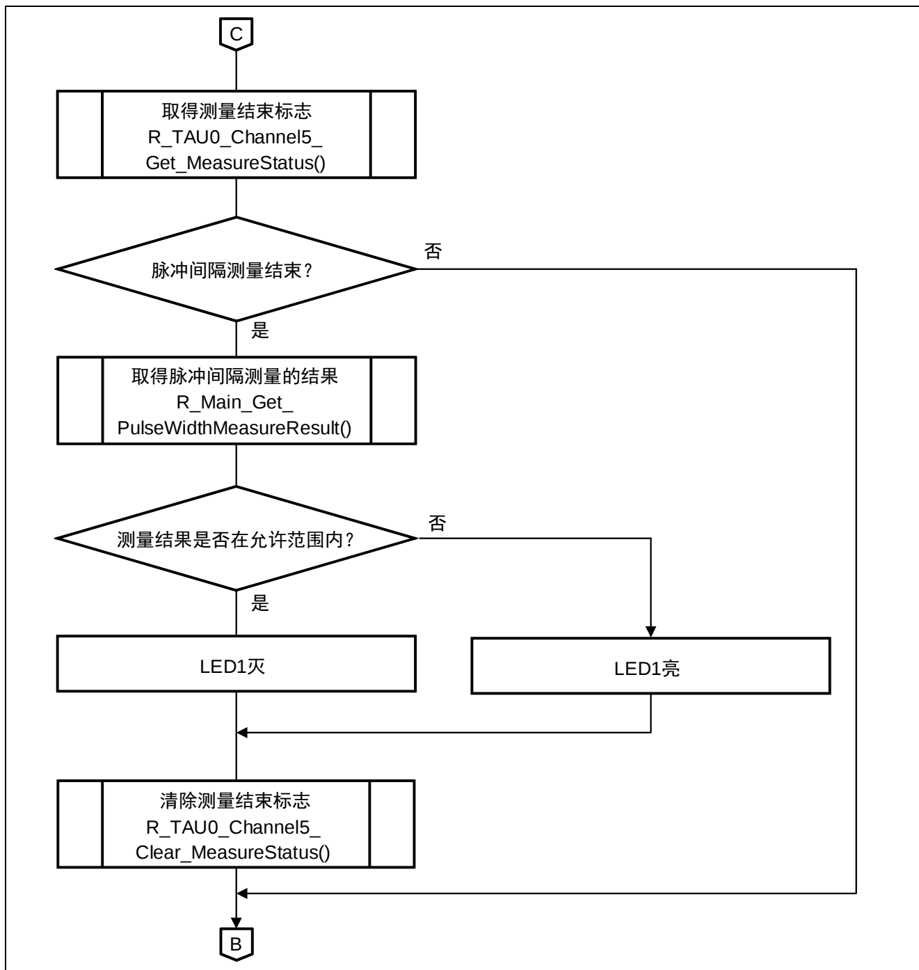
图 5.9 主函数处理（2/3）
