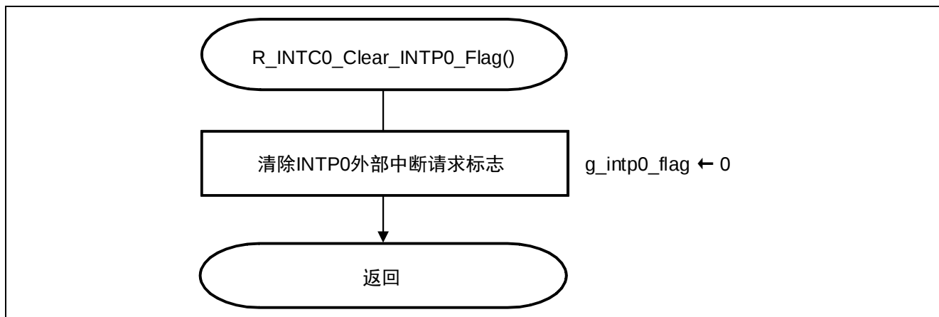
图 5.28 清除 INTP0 外部中断产生标志
