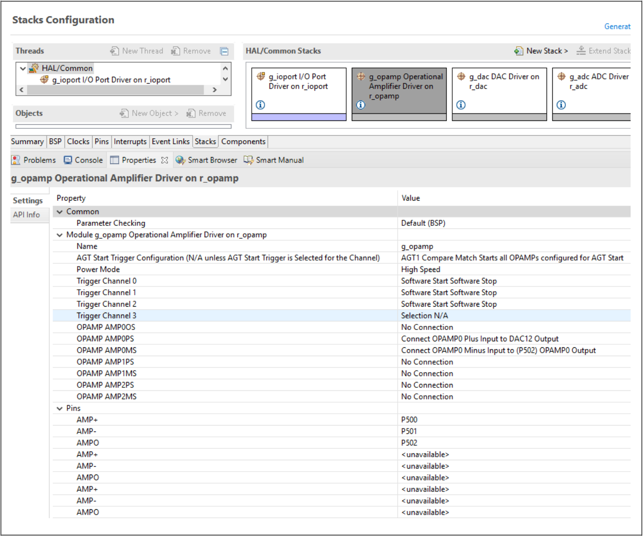
图31. 使用 Renesas FSP 配置器设置RA2A1 OPAMP的示例
