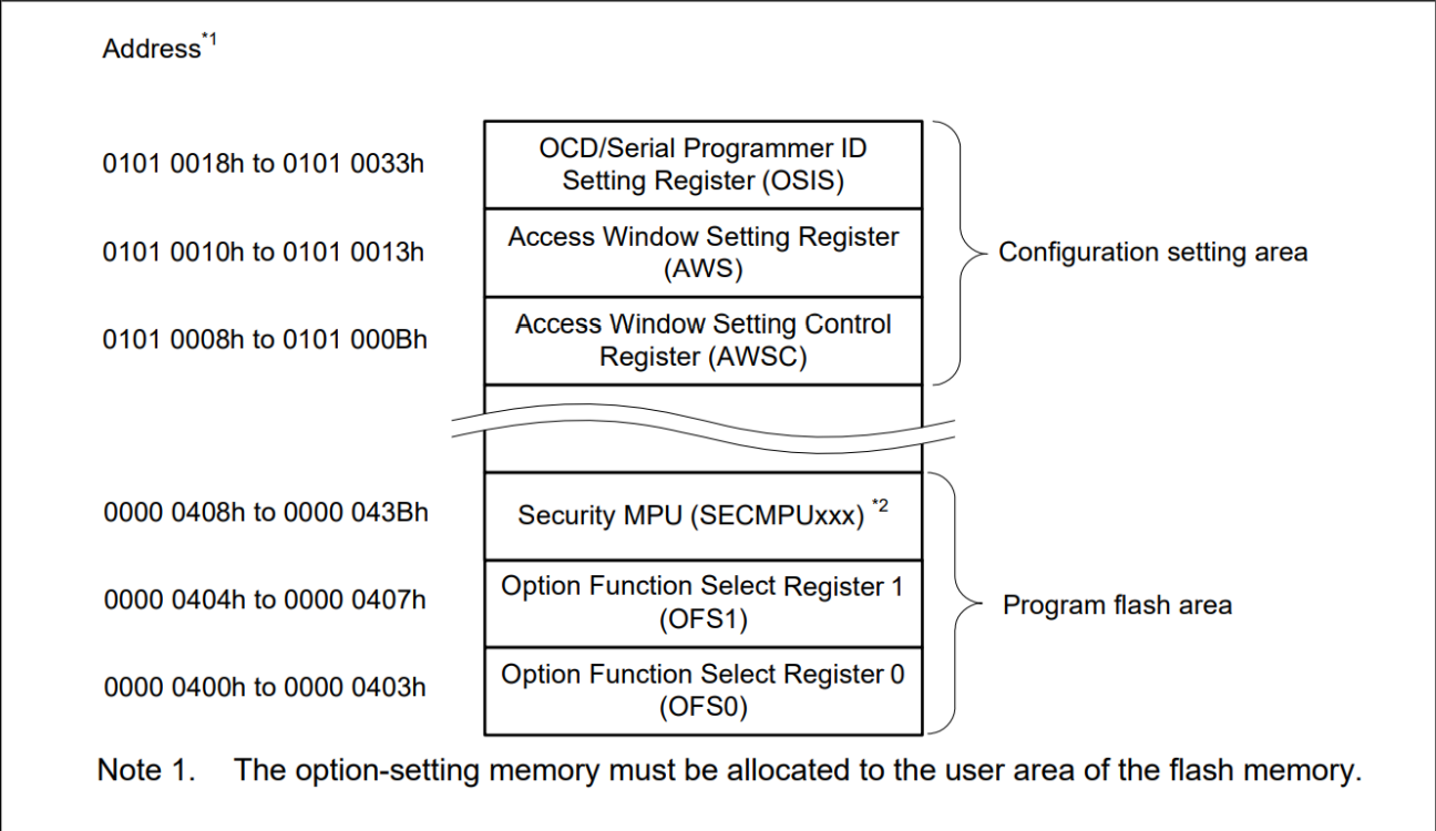
图6. RA2A1的选项功能选择寄存器
