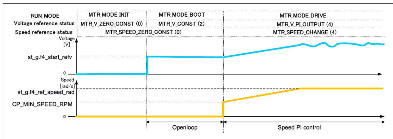
図 3-6 始動方法例
