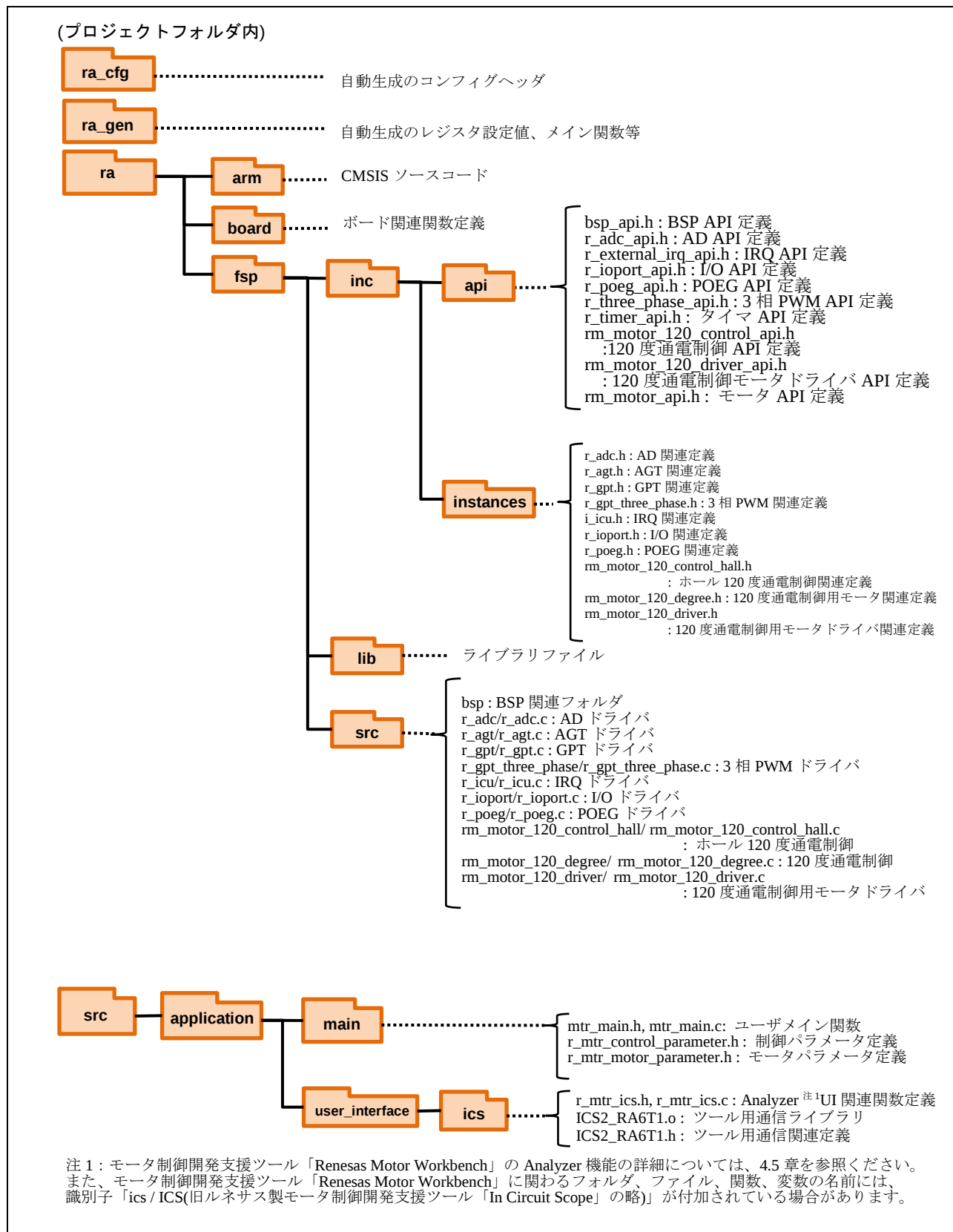
図 2-8 フォルダ・ファイル構成
