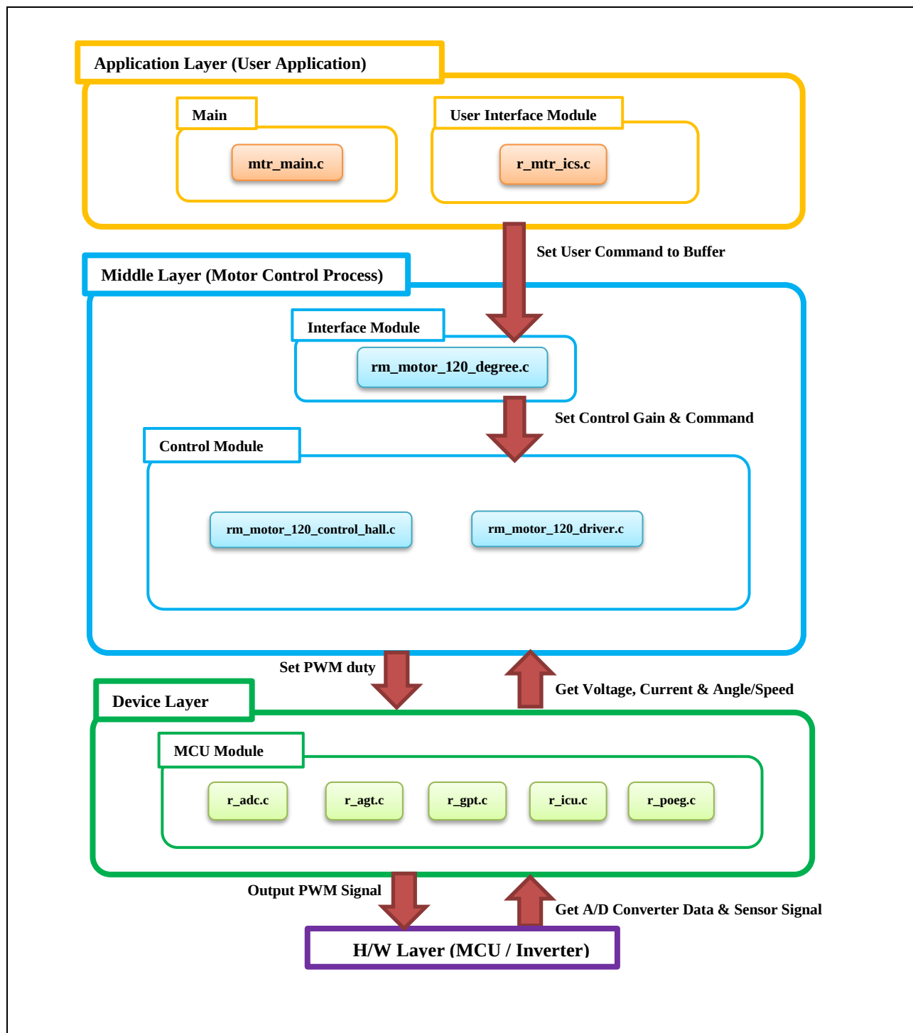
図 2-9 モジュール構成
