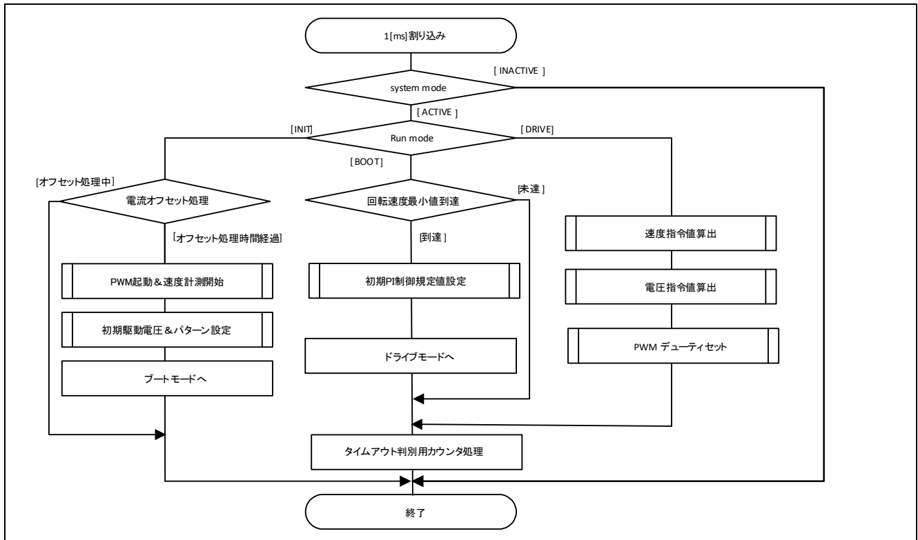
図 3-13 1 [ms]周期割り込み処理フローチャート
