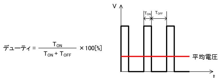
図 3-2 PWM 制御
