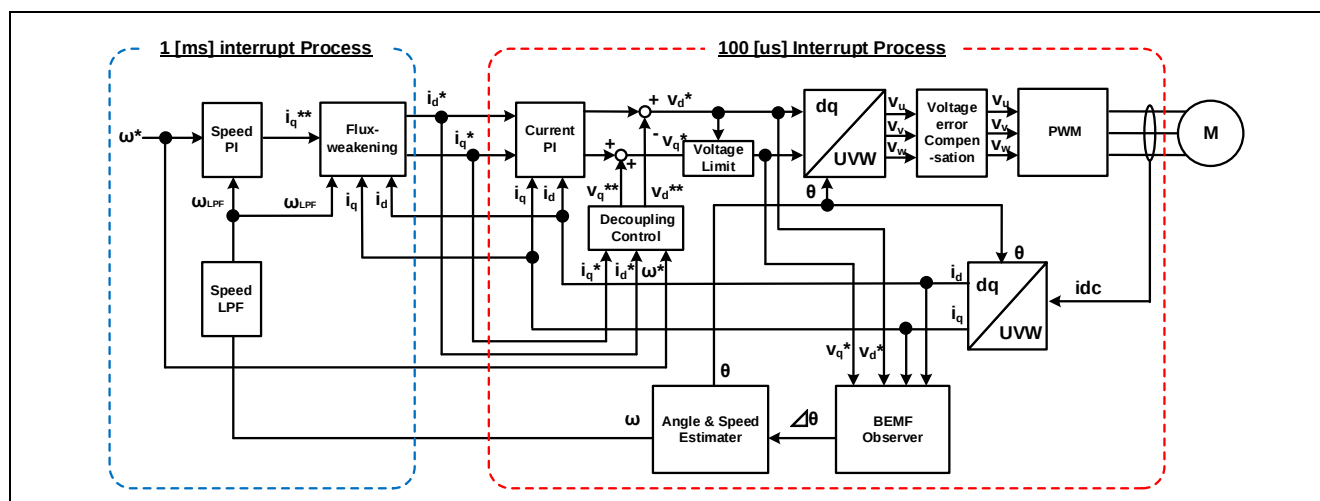
図 3-10 センサレスベクトル制御概略ブロック図(センサレス制御時)
