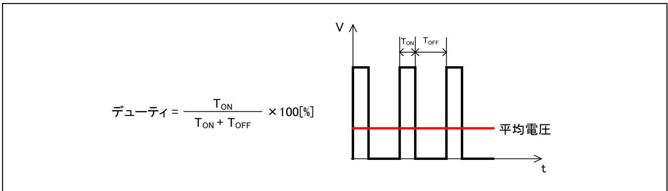
図 3-2 PWM 制御
