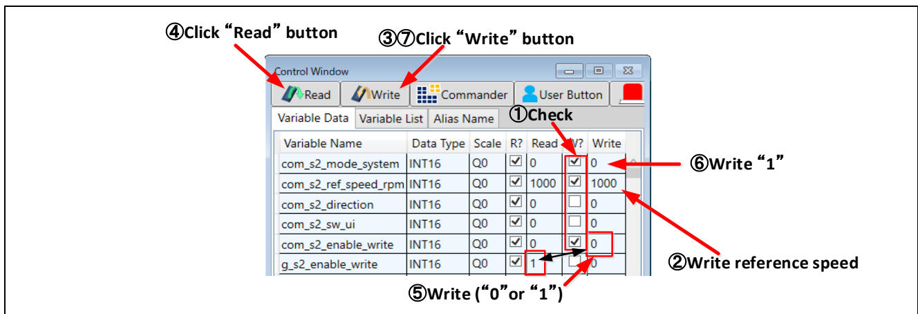
図 4-2 モータ回転の手順
