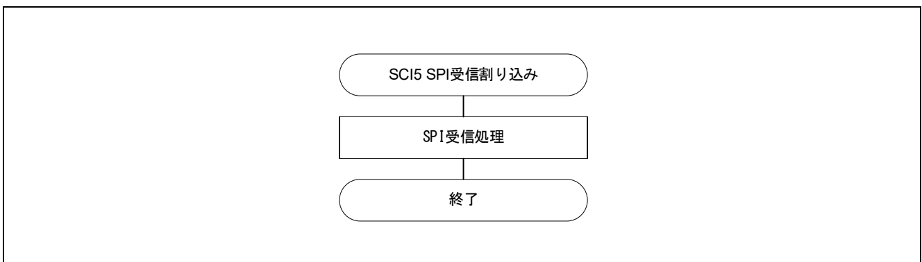
図 3-13 SCI5 SPI 受信割り込み処理フローチャート
