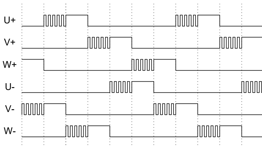
図 3-3 非相補前半 60 度チョッピング
