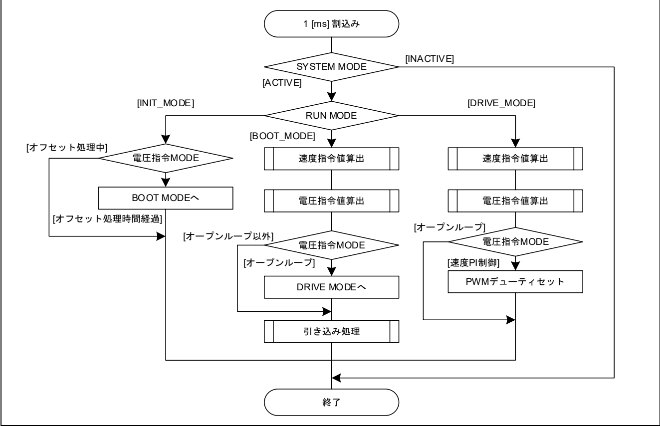
図 3-9 コンペアマッチタイマ 1 [ms]割り込み処理フローチャート
