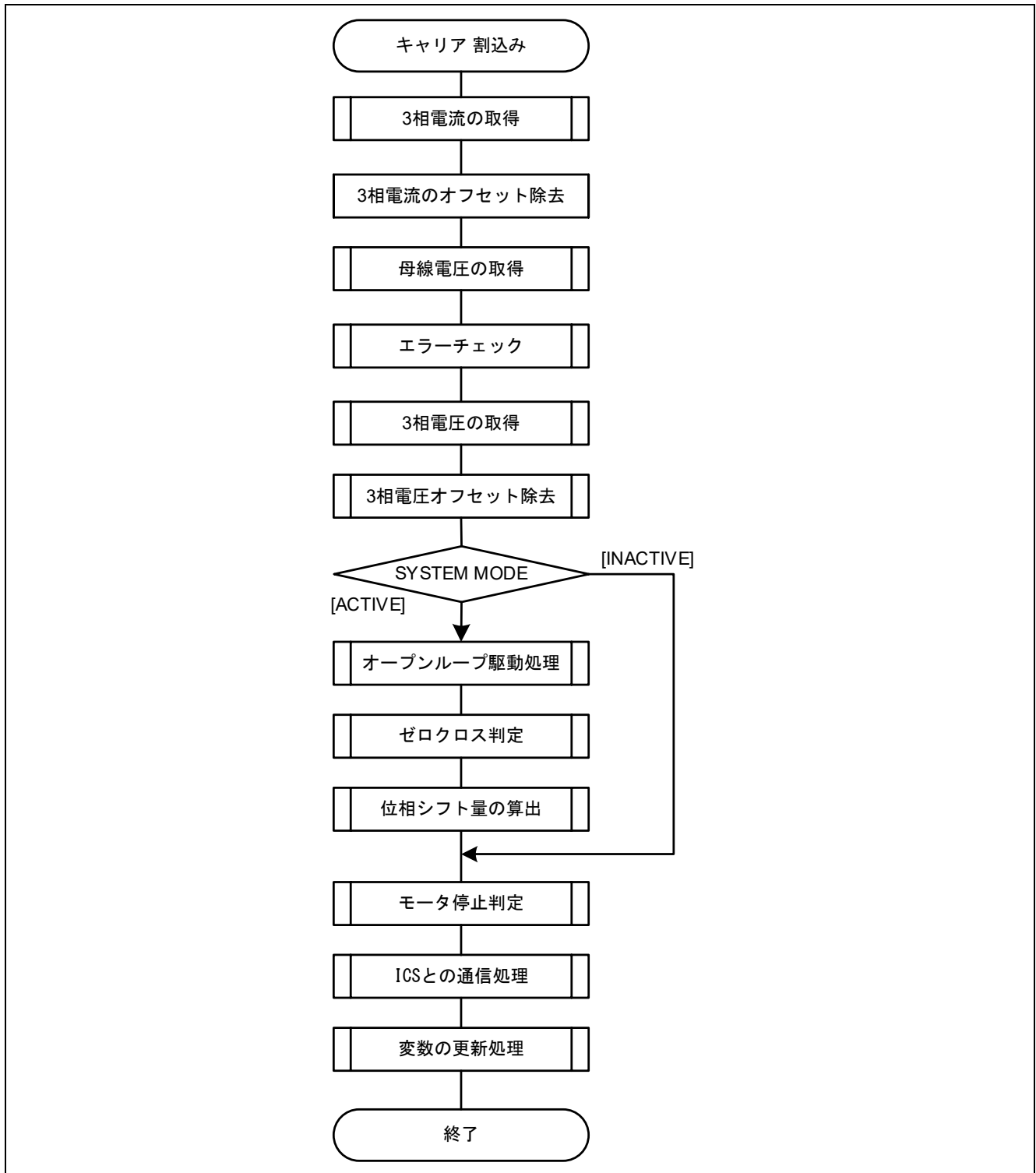
図 3-8 50 [μs]周期割り込み処理フローチャート (センサレス 120 度制御時)
