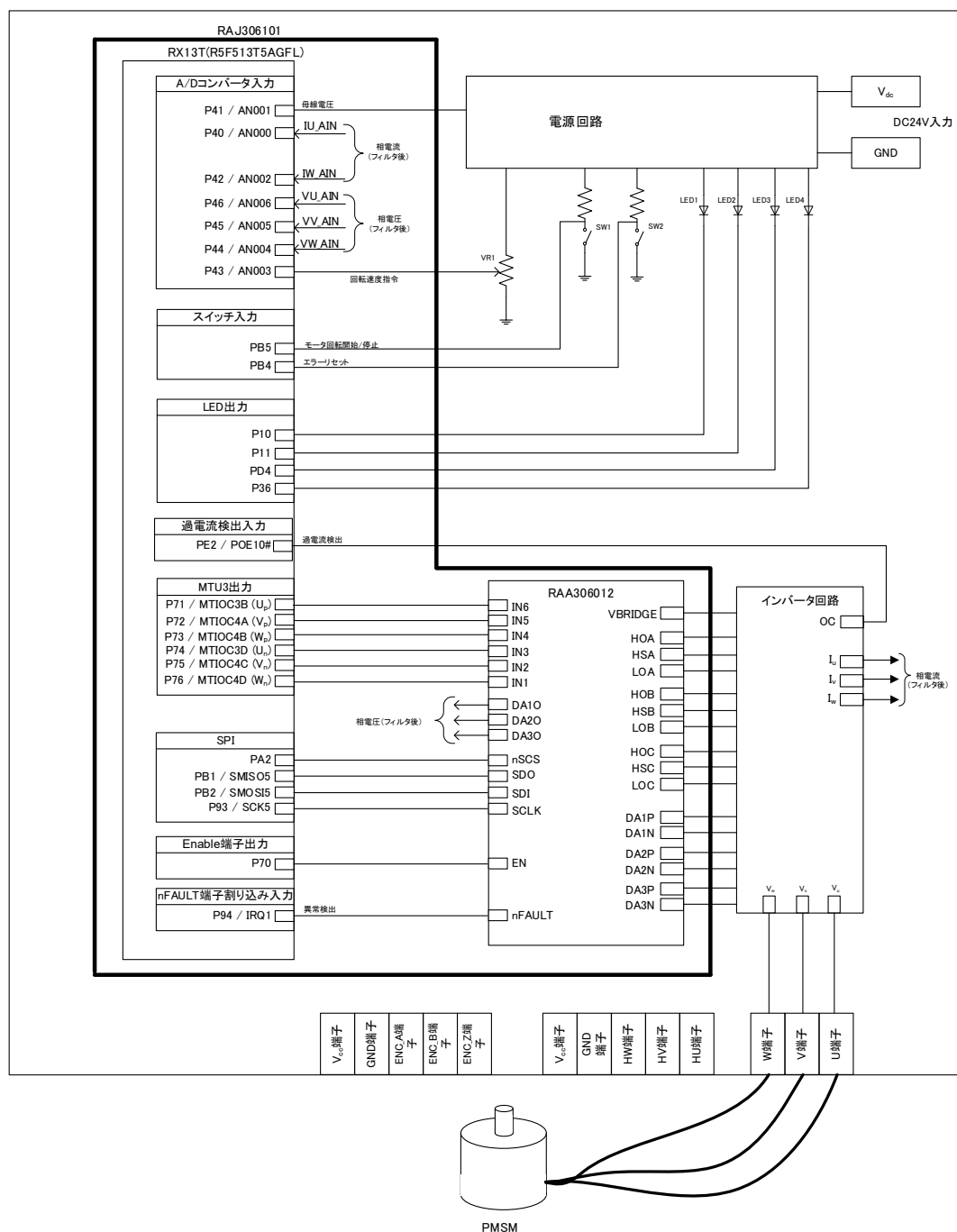
図 2-1 ハードウェア構成図
