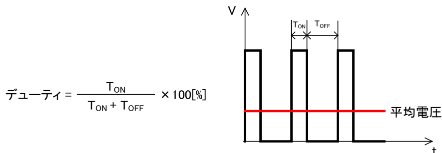
図 3-2 PWM 制御
